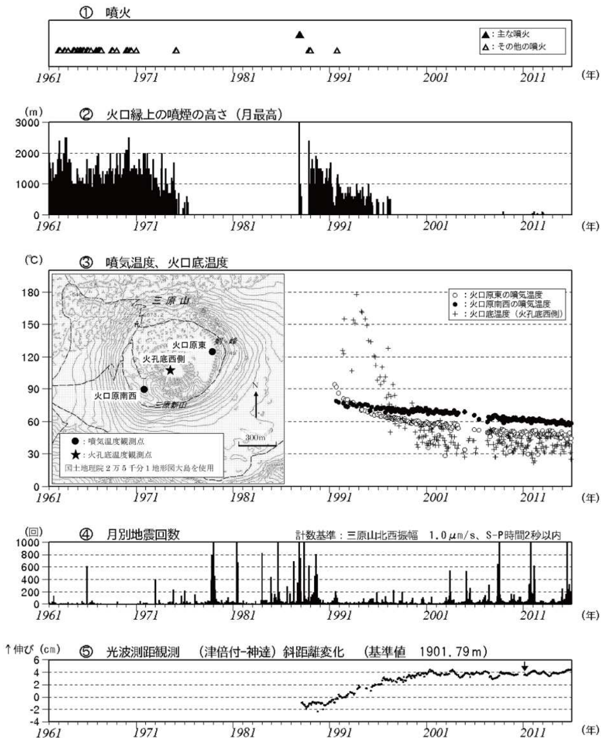
図 1 伊豆大島 長期間の火山活動経過図（1961 年 1 月～2015 年 1 月 31 日） 1991 年 12 月 18 日までは火口縁上 130m 以上、2002 年 2 月 28 日までは火口縁上 300m 以上の噴煙の高さを観測していました。 火口底温度（火口底西側）は赤外放射温度計を用いて離れた場所から測定した値。 噴気温度（火口原東、火口原南西）はサーミスタ温度計を用いて直接測定した値。 地震回数には伊豆大島周辺海域で発生した地震も一部含まれています。 光波距離計 4) による月平均値（観測開始は 1987 年 1 月）。グラフの空白部分は欠測。矢印は機器更新を示します。 4) レーザなどを用いて山体に設置した反射鏡までの距離を測定する機器。山体の膨張や収縮による距離の変化を観測します。
