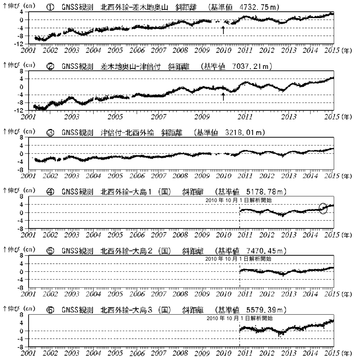
図3 伊豆大島 GNSS連続観測による基線長変化(2001年1月~2015年1月31日)(国): 国土地理院 2010年10月以降のデータについては、電離層の影響を補正する等、解析方法を改良しています。 ~ は図8のGNSS基線 ~ に対応しています。 グラフの空白部分は欠測。 の矢印は差木地奥山支柱工事を実施。 のグラフで7月28日頃みられる変動(丸印)は地震活動の活発化に伴う大島1観測点の動きによるものと考えられます。
