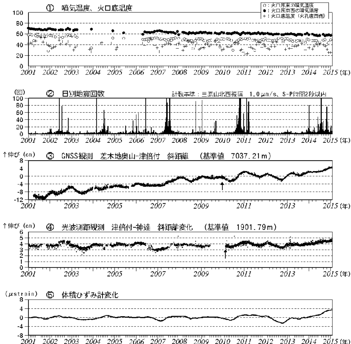
図 2 伊豆大島 最近の火山活動経過図（2001 年 1 月～2015 年 1 月 31 日）
