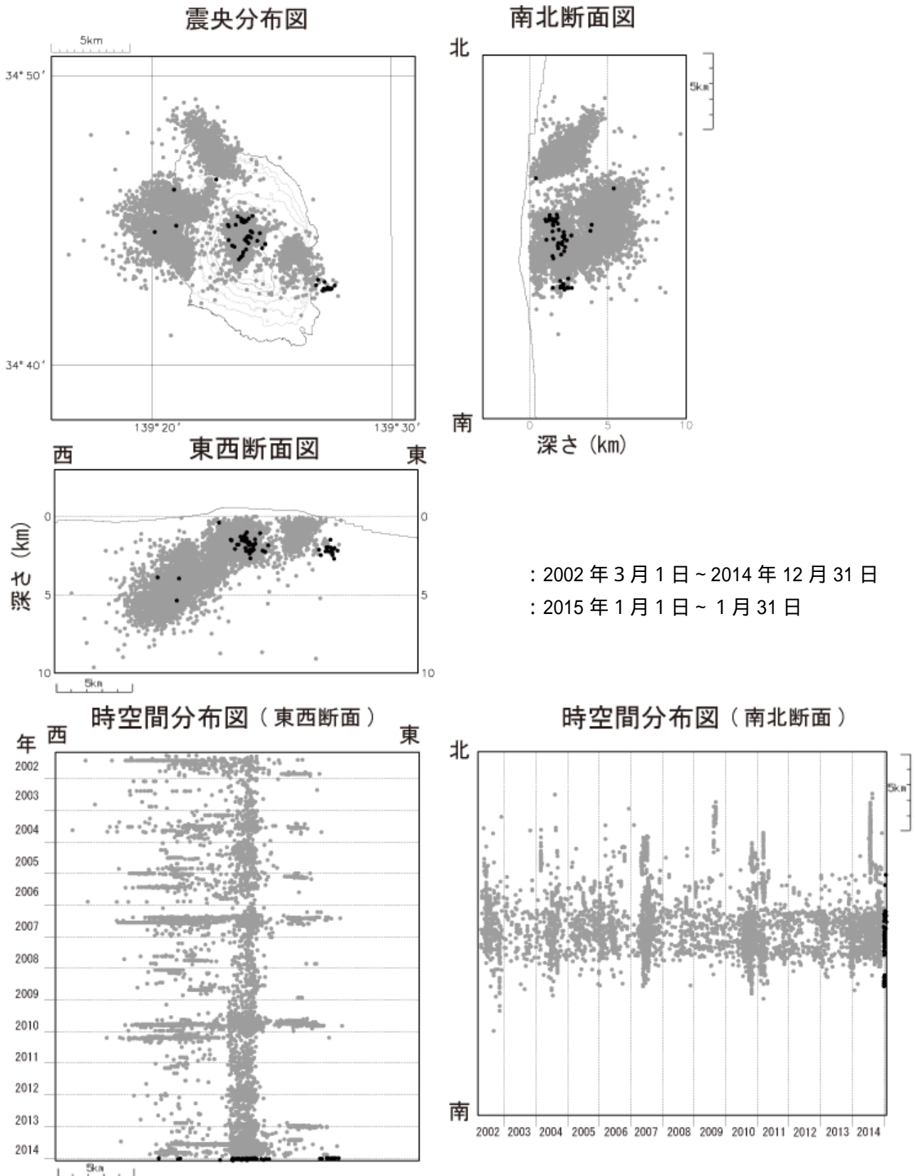
図 4 伊豆大島 震源分布図（2002 年 3 月 1 日 ~ 2015 年 1 月 31 日）
