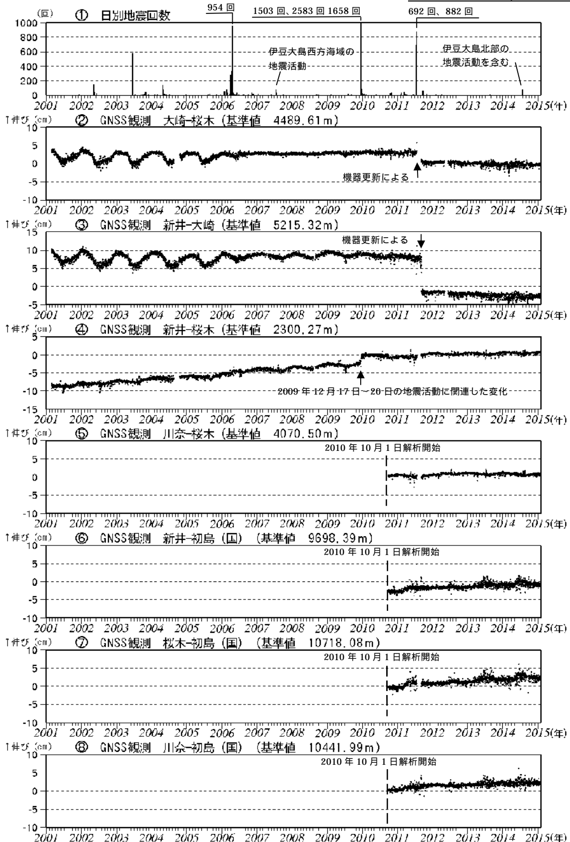
図3 伊豆東部火山群 火山活動経過図(2001年1月1日~2015年1月31日)
