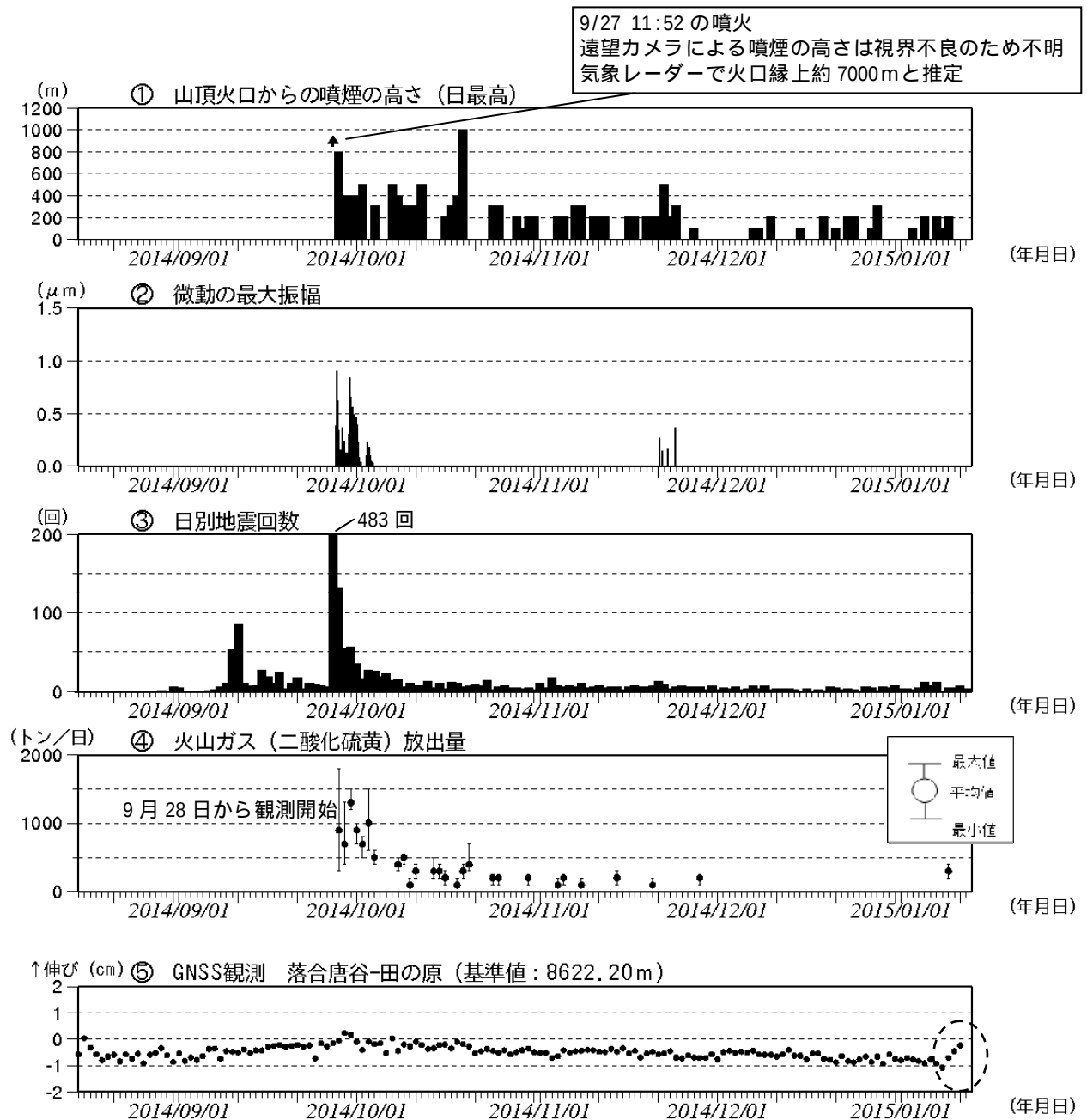
図 2 御嶽山 日別活動状況（2014 年 8 月 15 日～2015 年 1 月 12 日（速報値含む）） 遠望カメラによる噴煙の高さ 噴煙の高さは日最大値（噴火時以外は定時観測（09 時・15 時）の値）。 矢印は噴火開始を示します。また、視界不良時には噴煙の高さが表示されていませんが、噴火発生 以降は噴煙が連続的に発生しているものと考えられます。
