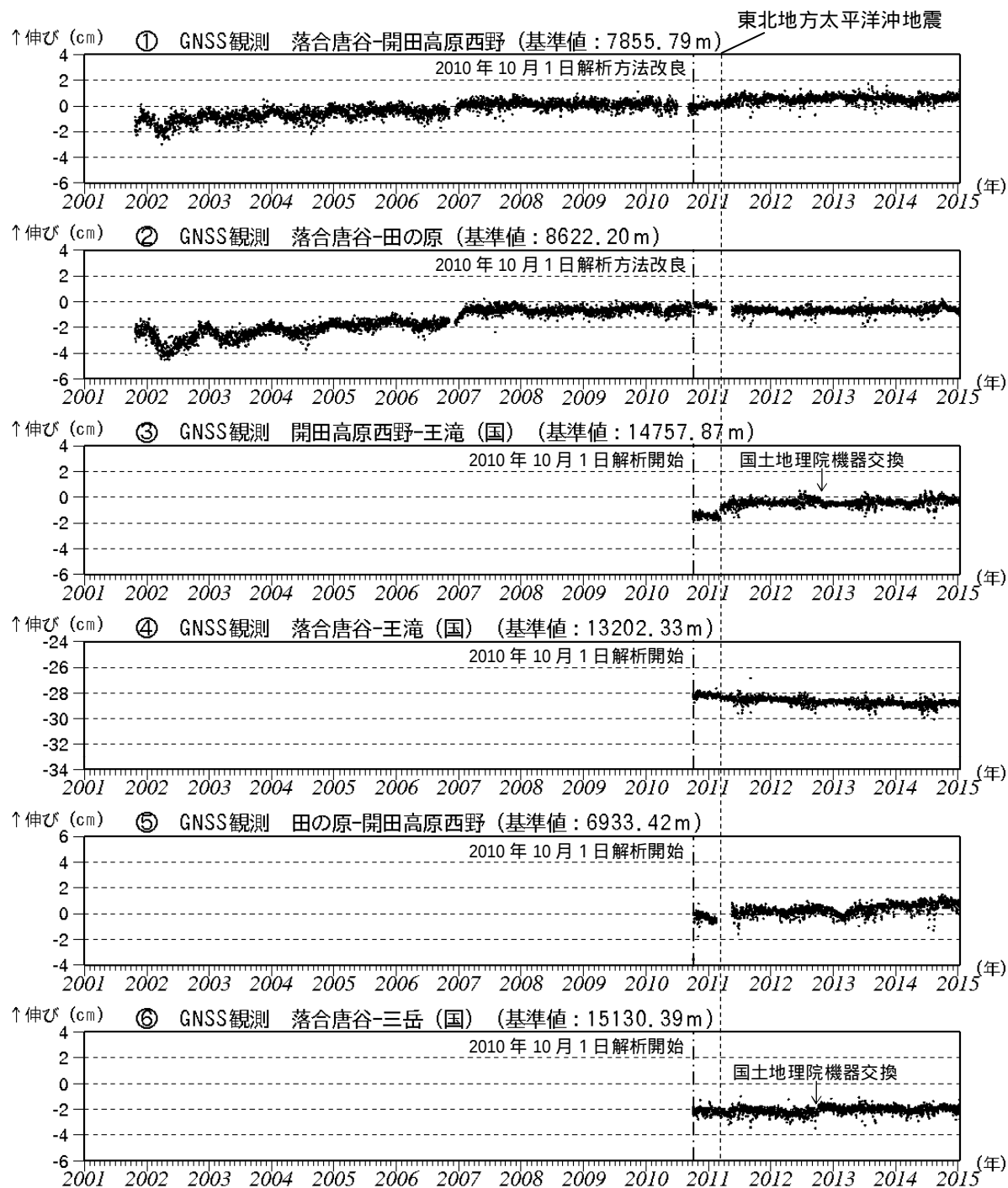
図3 御嶽山 GNSS連続観測による基線長の長期変化 (2001年1月1日～2015年1月11日)
