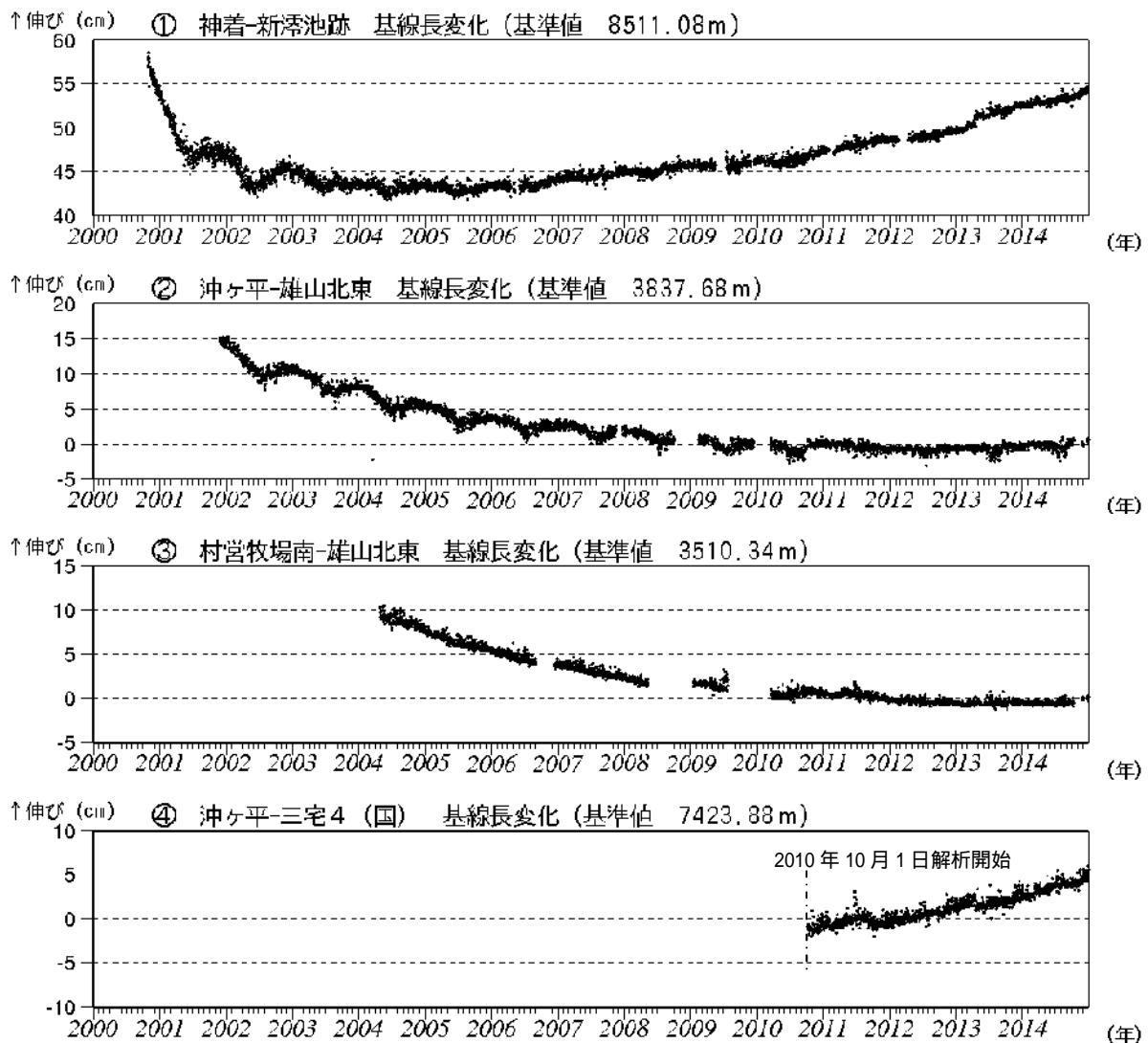
図5 三宅島 GNSS 連続観測結果(2000年1月1日～2014年12月31日) (国): 国土地理院 ・基線 ~ は図8(観測点配置図)の ~ にそれぞれ対応します。 ・グラフの空白部分は欠測を示します。 ・2010年10月以降のデータについては、電離層の影響を補正する等、解析方法を改良しています。
