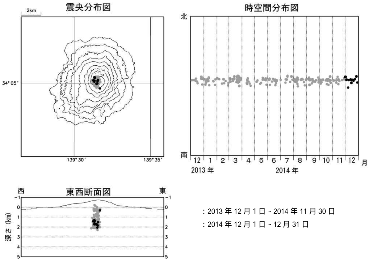
図6 三宅島 震源分布図(2013年12月1日~2014年12月31日)
