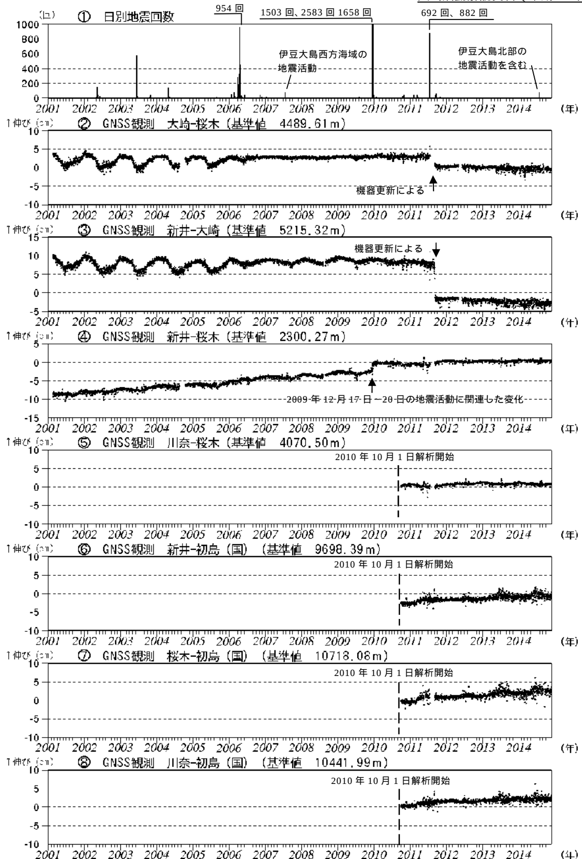
図3 伊豆東部火山群 火山活動経過図（2001年1月1日～2014年12月31日）
