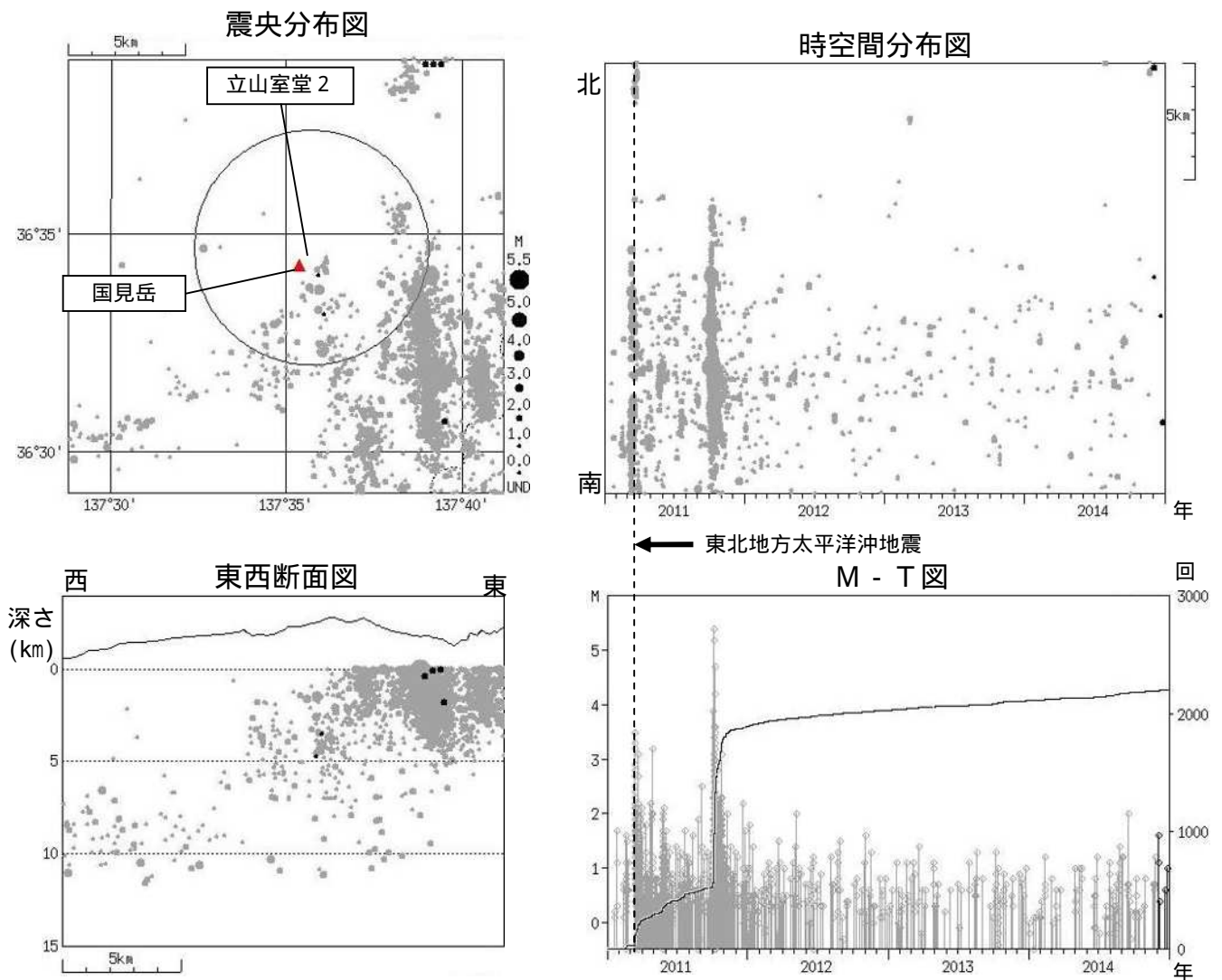
図2 弥陀ヶ原 広域地震観測網による山体・周辺の地震活動(2011年1月1日~2014年12月31日) : 2011年1月1日~2014年11月30日 : 2014年12月1日~12月31日 ・ 震央分布図内の円は、立山室堂に設置した地震計(立山室堂2)で地震回数を計数しているS-P時間1秒以内となるおよその範囲を示します。 ・ M(マグニチュード)は地震の規模を表します。 ・ 図中の震源要素は一部暫定値が含まれており、後日変更することがあります。 ・ 弥陀ヶ原近傍の地震活動は、低調に経過しています。
