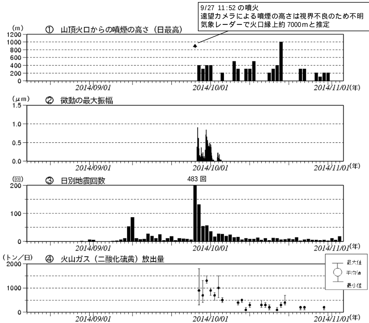
図 3 御嶽山 日別活動状況（2014 年 8 月 15 日～11 月 3 日（速報値含む））
