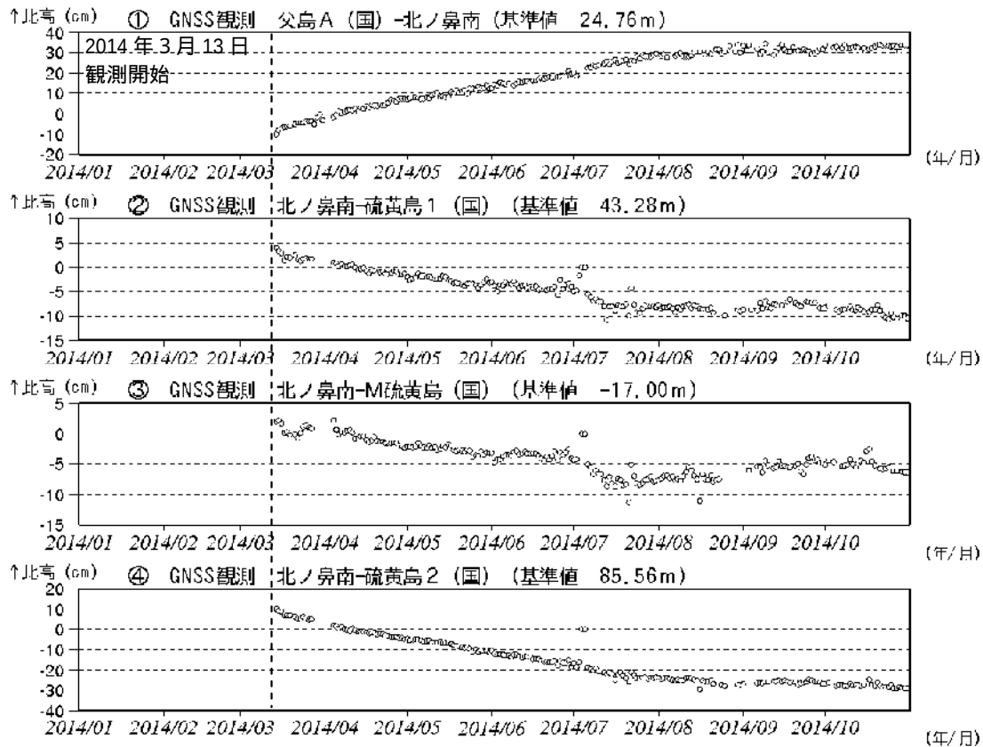
図7 硫黄島 GNSS 2) 観測結果（2014年1月～10月）（国）：国土地理院
