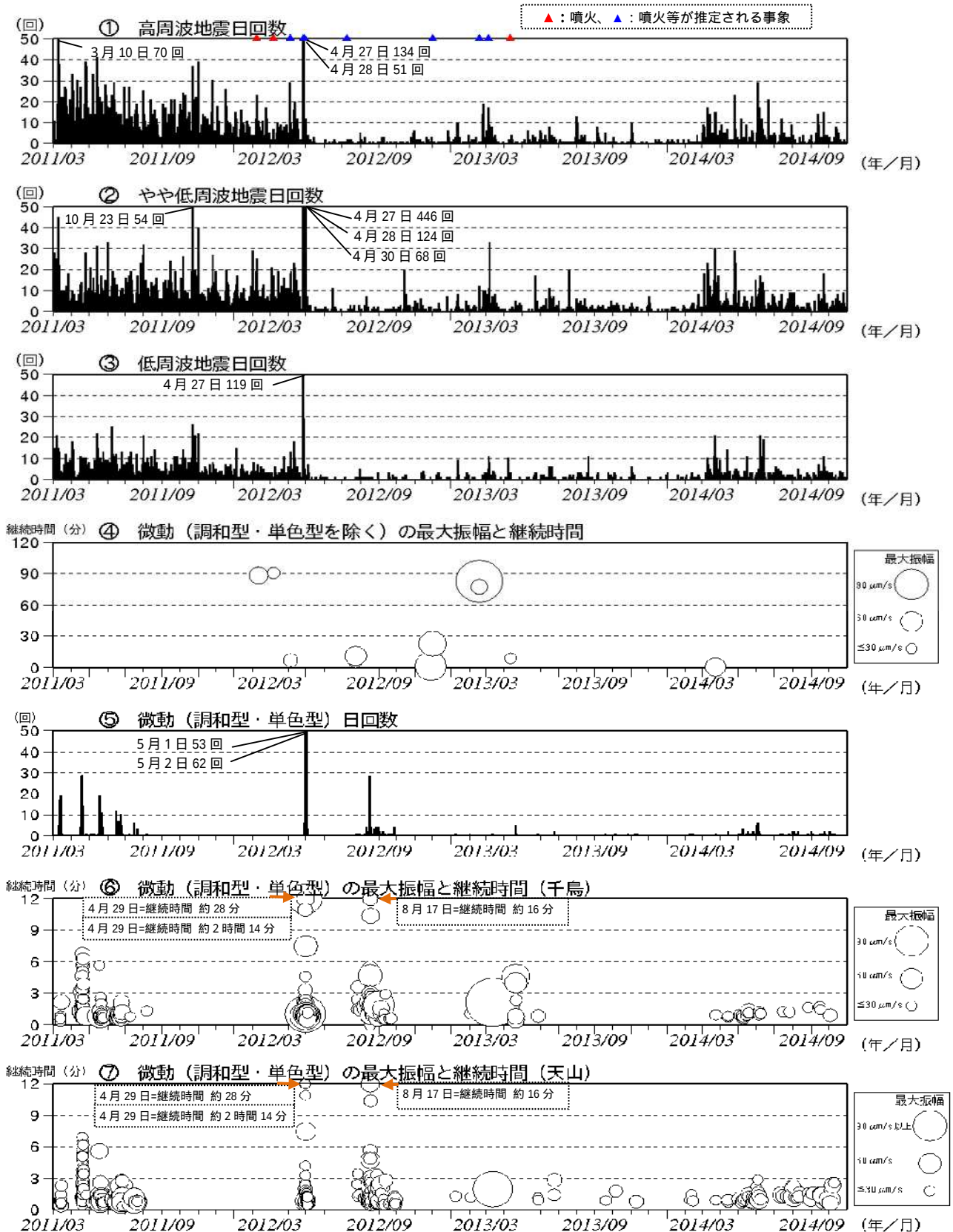
図5 硫黄島 火山活動経過図（2011年3月8日～2014年10月31日）
