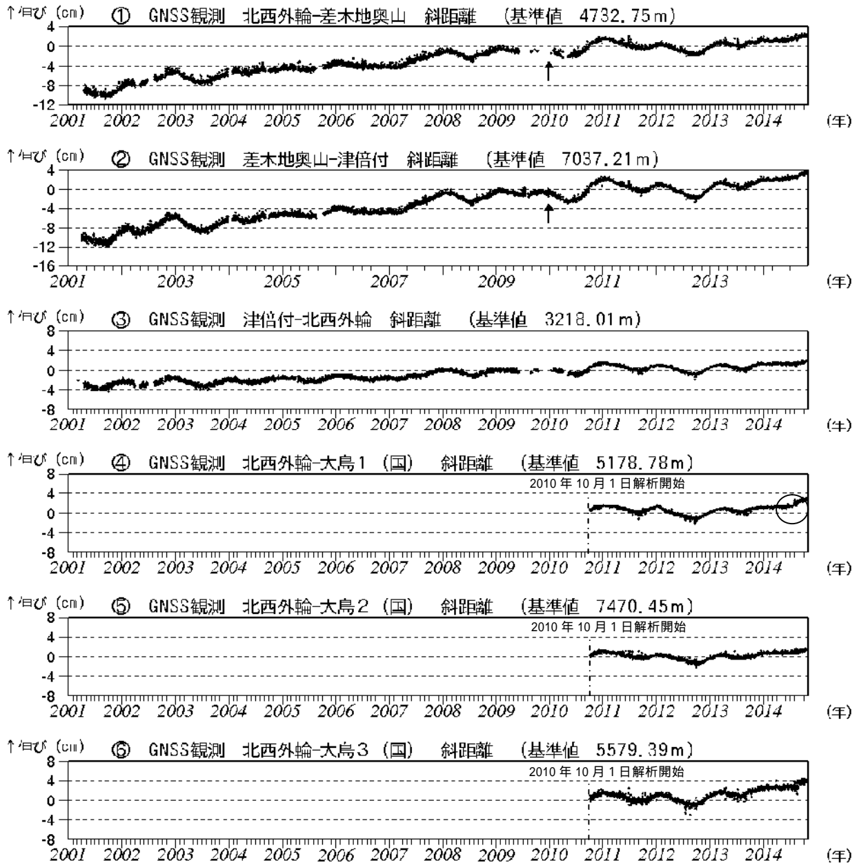
図3 伊豆大島 GNSS連続観測による基線長変化(2001年1月~2014年10月31日)(国): 国土地理院 2010年10月以降のデータについては、電離層の影響を補正する等、解析方法を改良しています。 ~ は図6のGNSS基線 ~ に対応しています。 グラフの空白部分は欠測。 の矢印は差木地奥山支柱工事を実施。 のグラフで7月28日頃みられる変動(丸印)は地震活動の活発化に伴う大島1観測点の動きによるものと考えられます。
