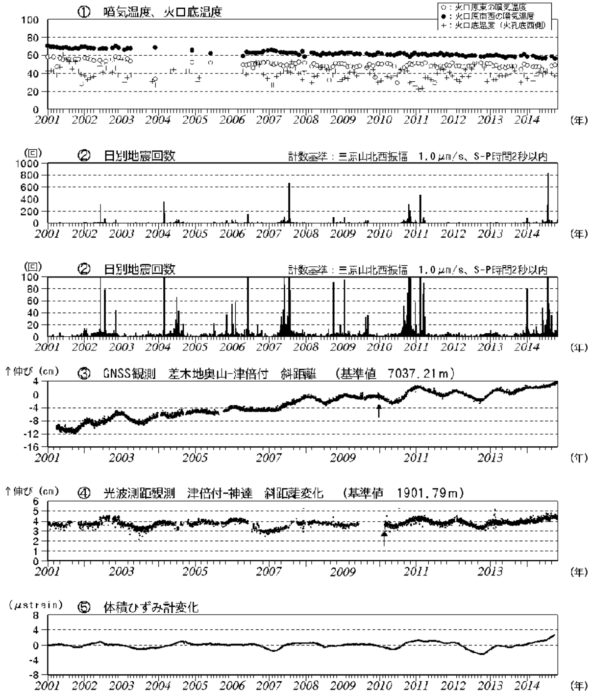
図2 伊豆大島 最近の火山活動経過図(2001年1月~2014年10月31日)
