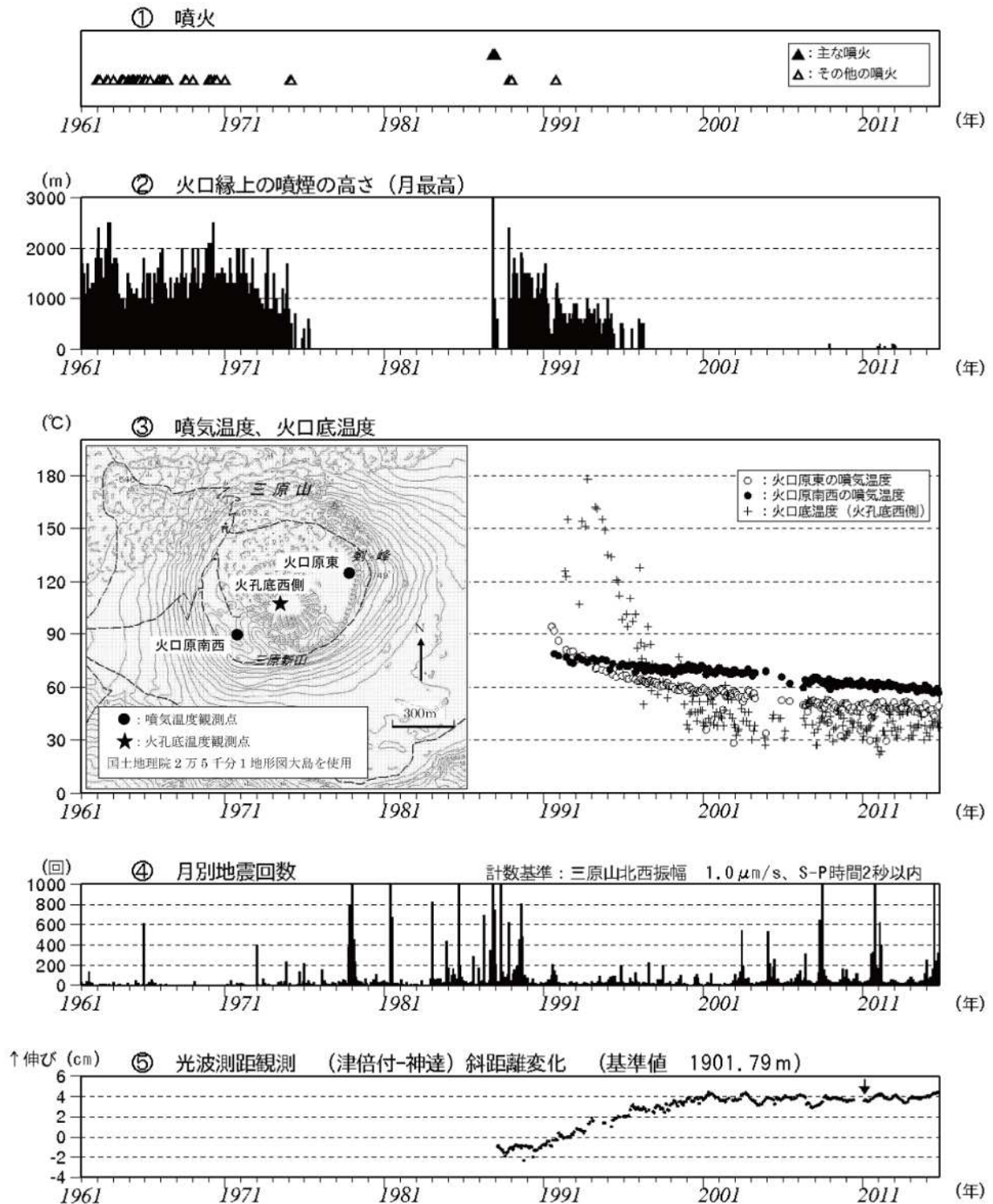
図1 伊豆大島 長期間の火山活動経過図(1961年1月~2014年10月31日) 1991年12月18日までは火口縁上130m以上、2002年2月28日までは火口縁上300m以上の噴煙の高さを観測していました。 火口底温度(火口底西側)は赤外放射温度計を用いて離れた場所から測定した値。 噴気温度(火口原東、火口原南西)はサーミスタ温度計を用いて直接測定した値。 地震回数には伊豆大島周辺海域で発生した地震も一部含まれています。 光波距離計 5) による月平均値(観測開始は1987年1月)。グラフの空白部分は欠測。矢印は機器更新を示します。
