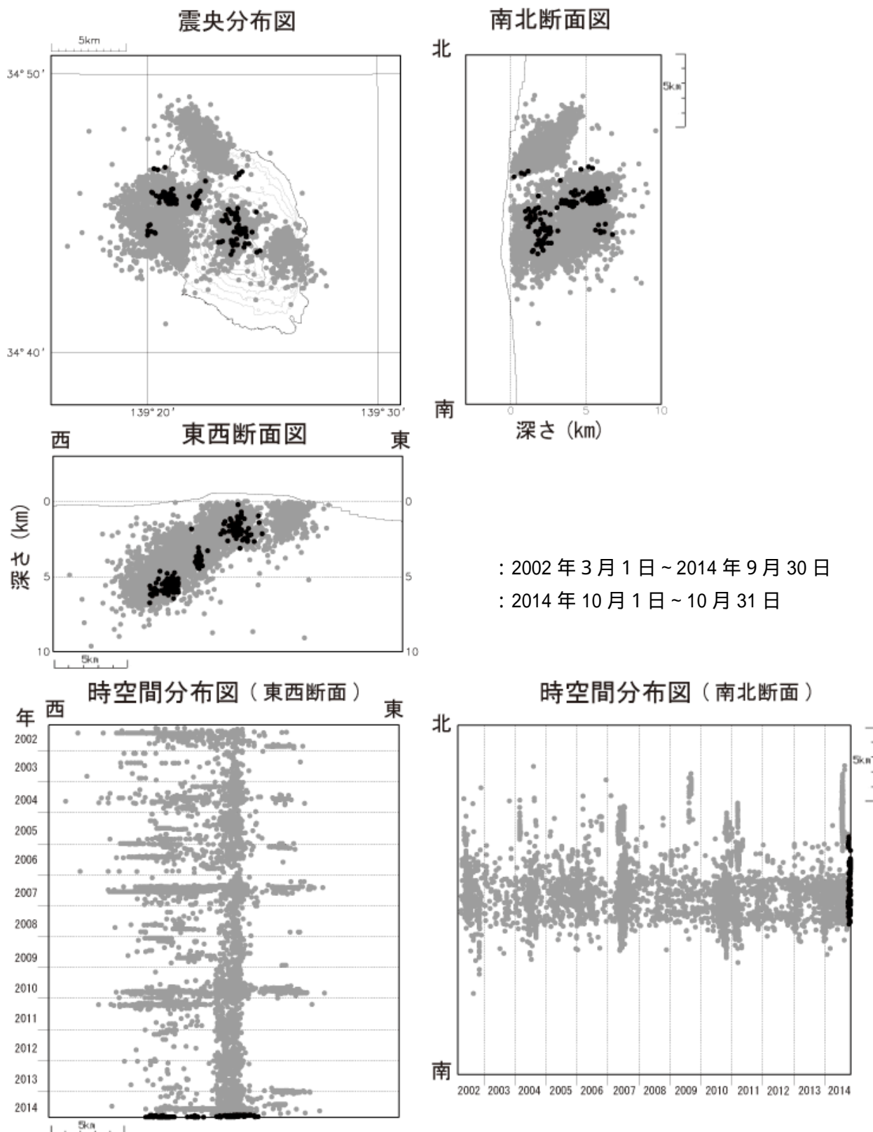
図4 伊豆大島 震源分布図（2002年3月1日～2014年10月31日）
