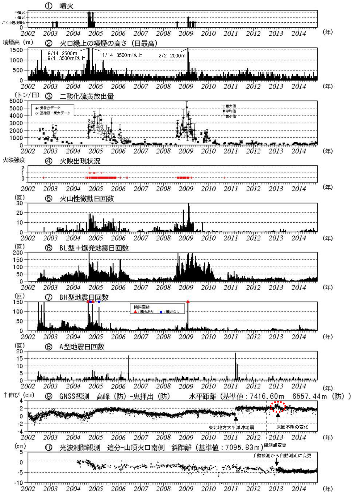
図 5 浅間山 火山活動経過図（2002 年 1 月 1 日～2014 年 10 月 31 日）
