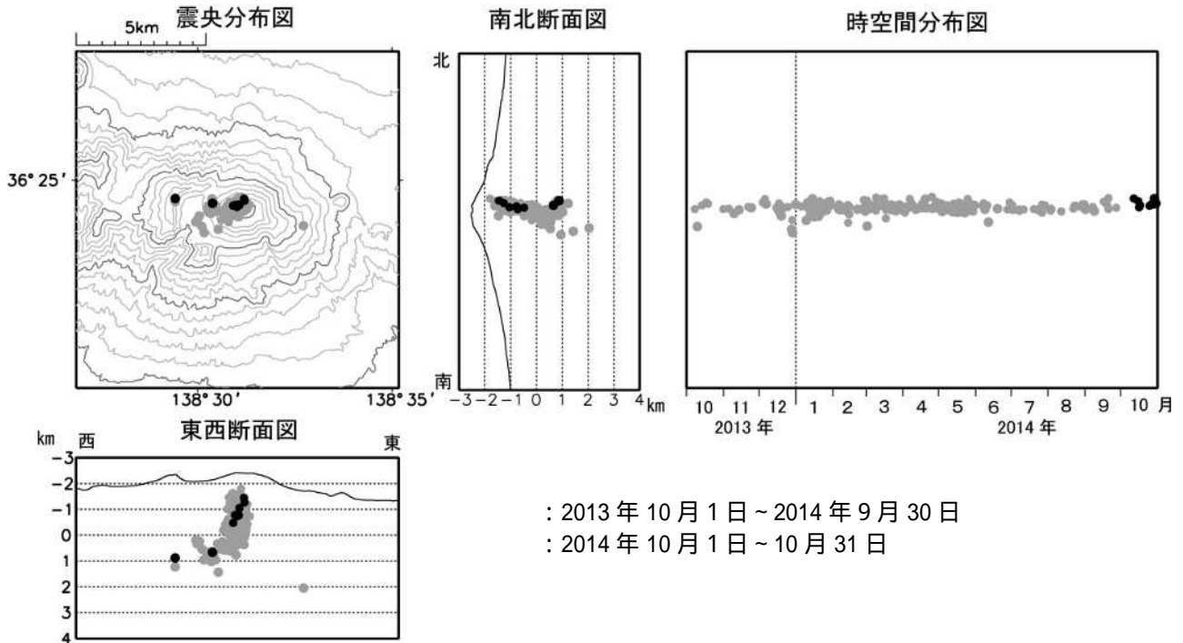
図 6 浅間山 震源分布図 ( 2013 年 10 月 1 日 ~ 2014 年 10 月 31 日 )
