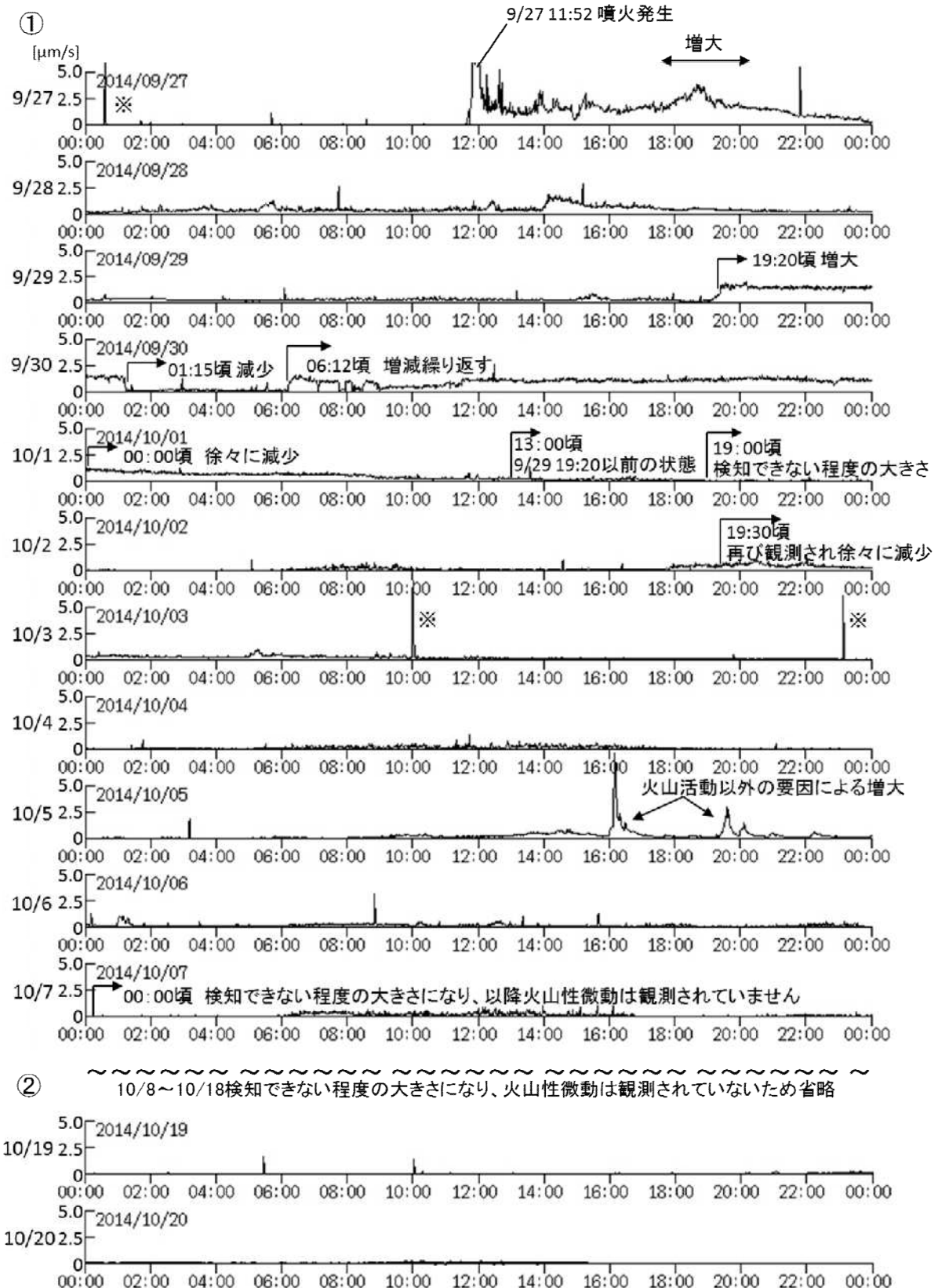
図 4 御嶽山 田の原上観測点（剣ヶ峰の南東約 2 km）の上下動地震波形の 1 分間振幅平均値の推移
