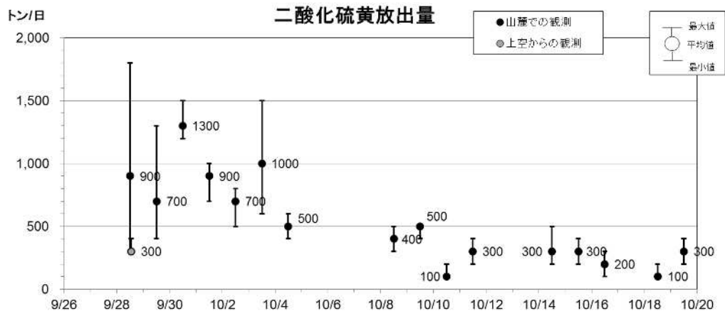
図2 御嶽山 火山ガス（二酸化硫黄）観測結果（9月28日～10月19日）
