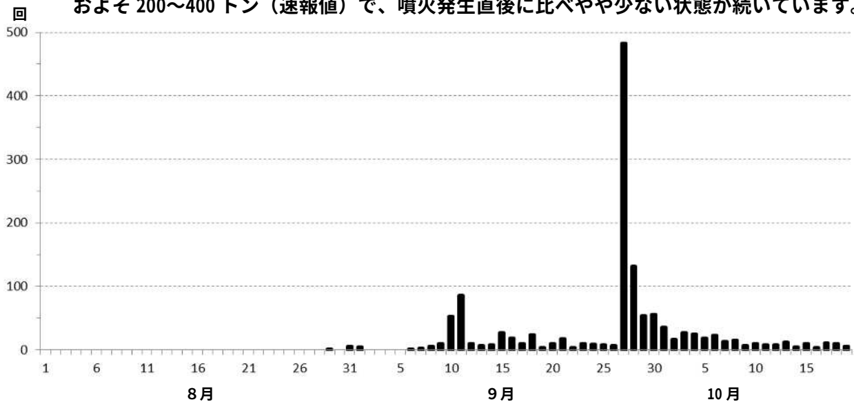
図3 御嶽山 日別地震回数（2014年8月1日～10月19日（速報値含む））
