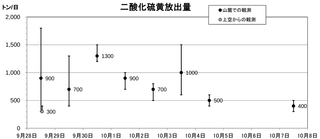
図 2 御嶽山 火山ガス（二酸化硫黄）観測結果（9 月 28 日～10 月 7 日）
