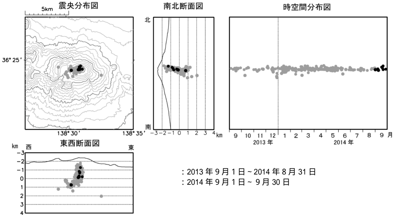
図4 浅間山 震源分布図(2013年9月1日~2014年9月30日)
