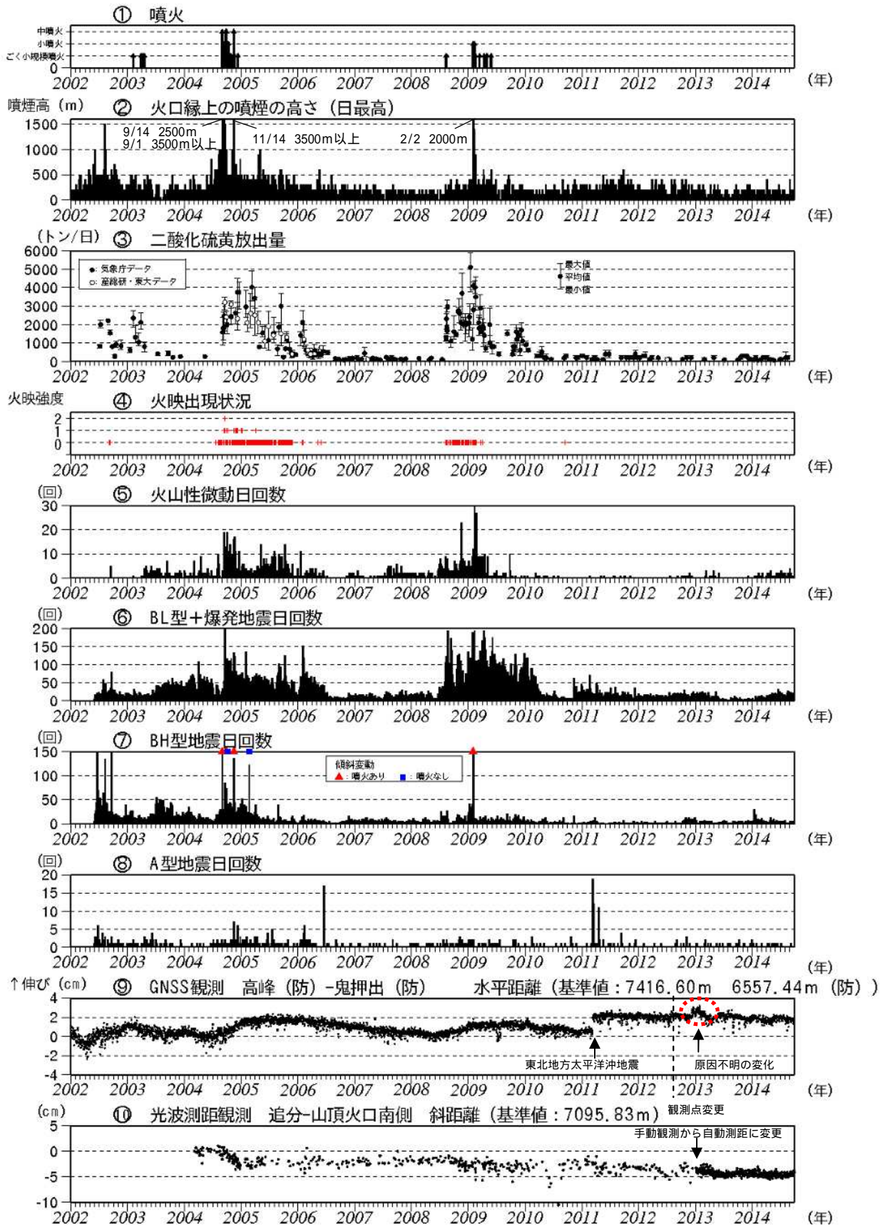
図3 浅間山 火山活動経過図(2002年1月1日~2014年9月30日)
