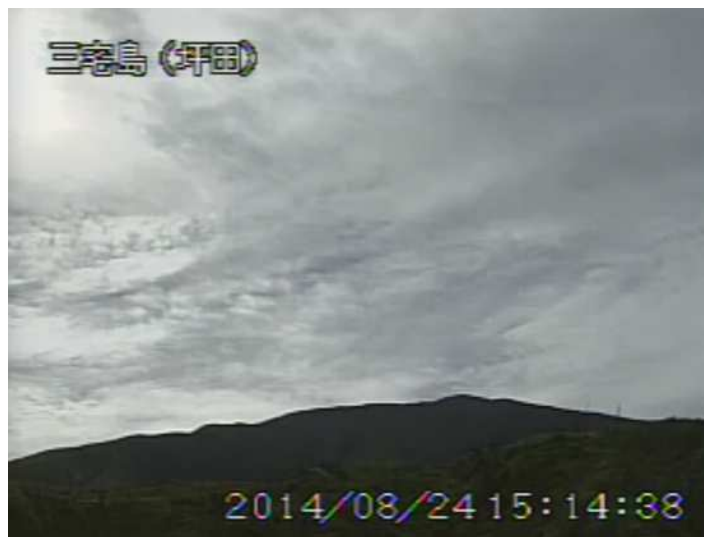
図1 三宅島 山頂火口からの噴煙の状況 （8月24日、坪田遠望カメラによる）
