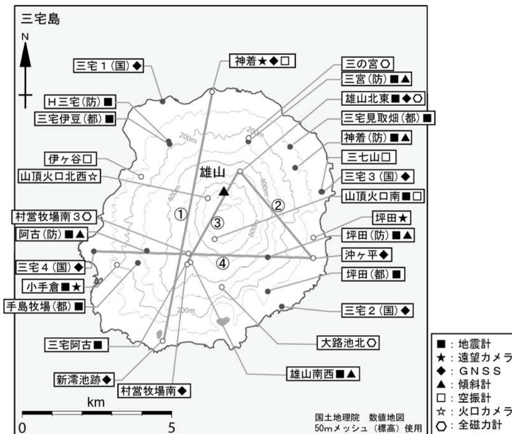
図2 三宅島 観測点配置図
