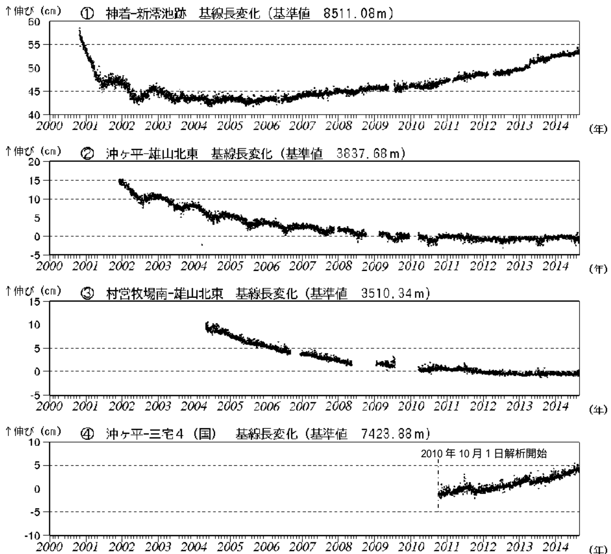
図 4 三宅島 GNSS 連続観測結果（2000 年 1 月～2014 年 8 月）（国）：国土地理院 ・基線 ～ は図 2（観測点配置図）の ～ にそれぞれ対応します。 ・グラフの空白部分は欠測を示します。 ・2010 年 10 月以降のデータについては、電離層の影響を補正する等、解析方法を改良しています。
