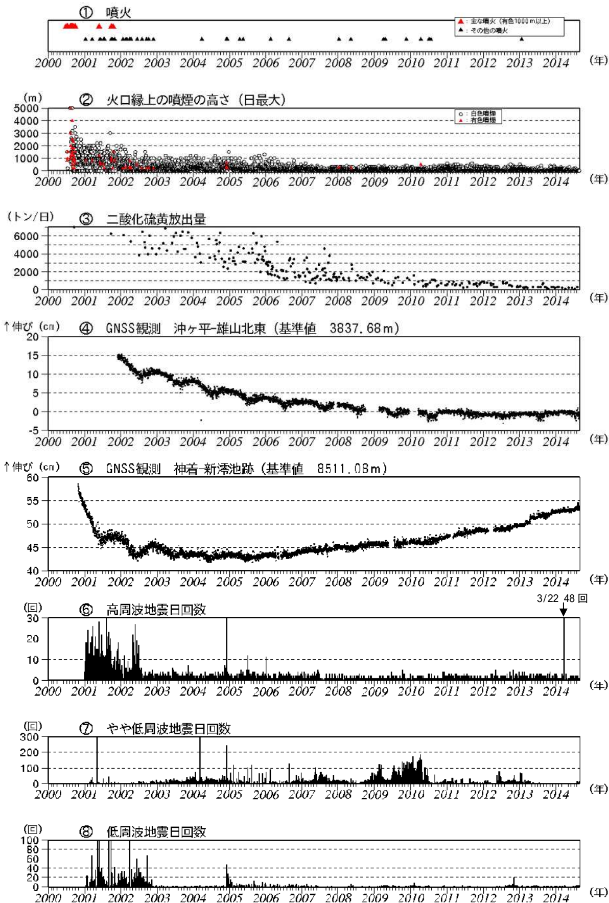
図3 三宅島 火山活動経過図(2000年1月~2014年8月)
