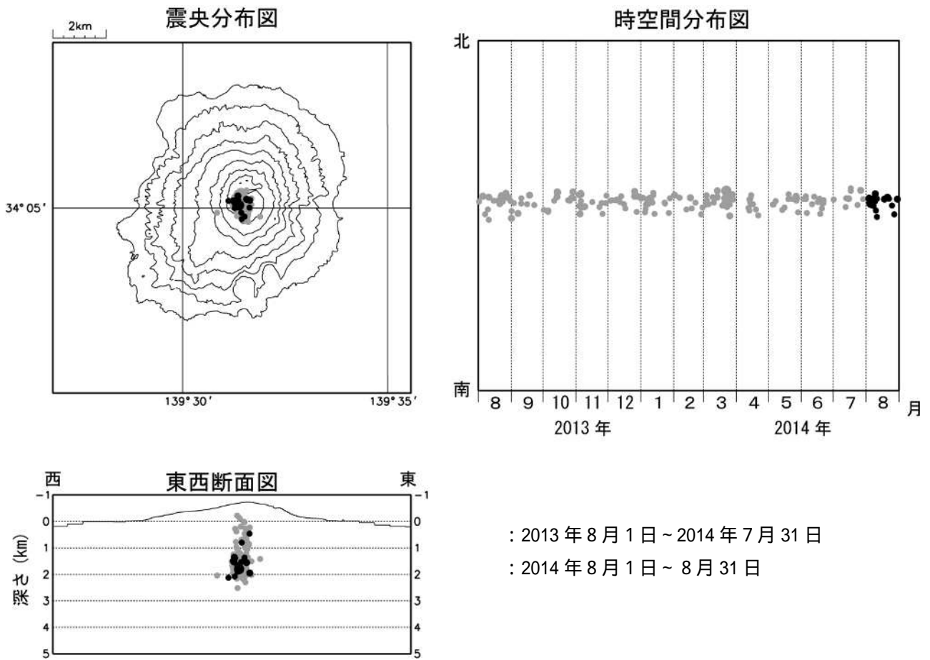
図5 三宅島 震源分布図(2013年8月1日~2014年8月31日)
