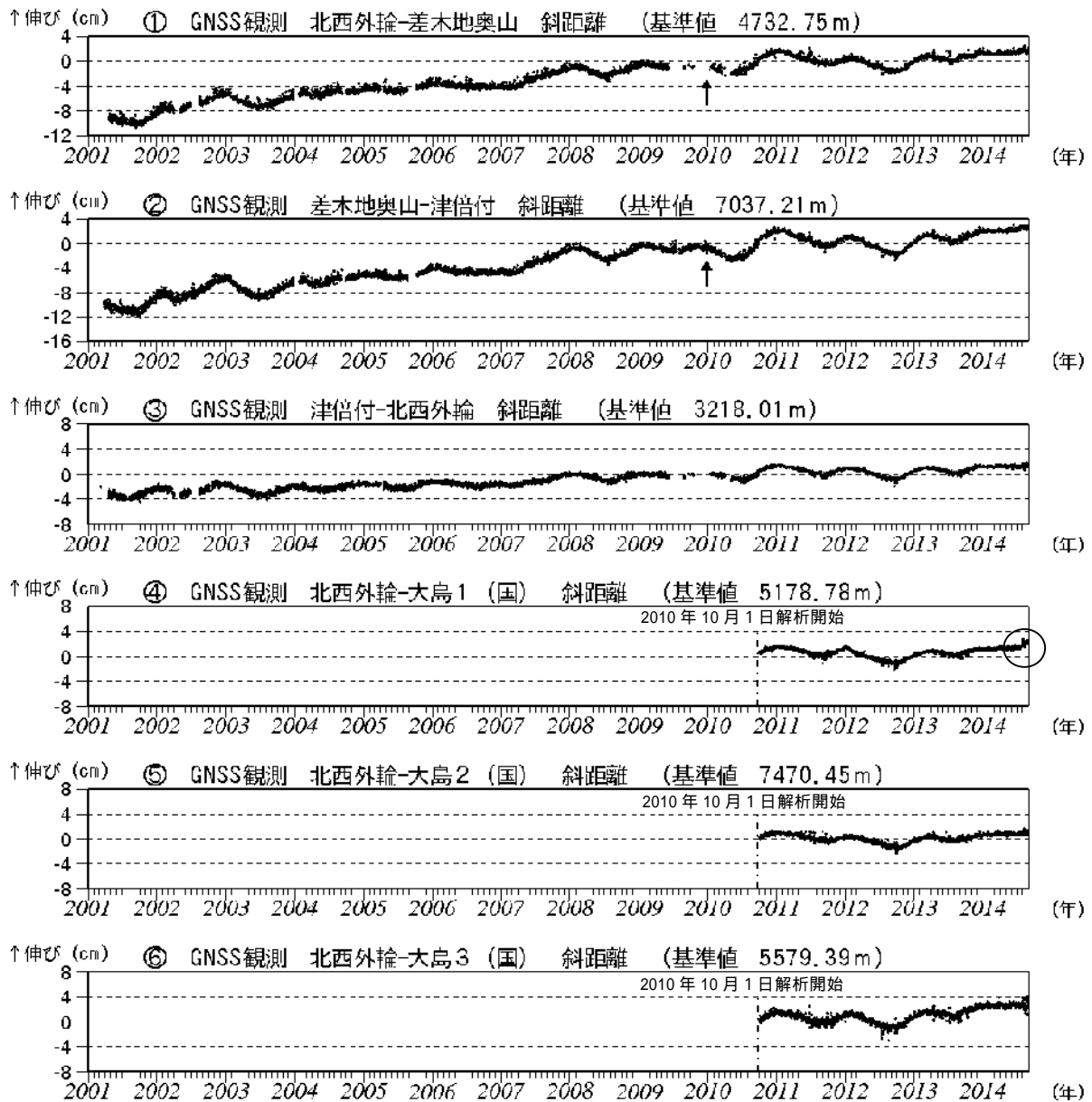
図3 伊豆大島 GNSS連続観測による基線長変化(2001年1月~2014年8月31日)(国): 国土地理院
