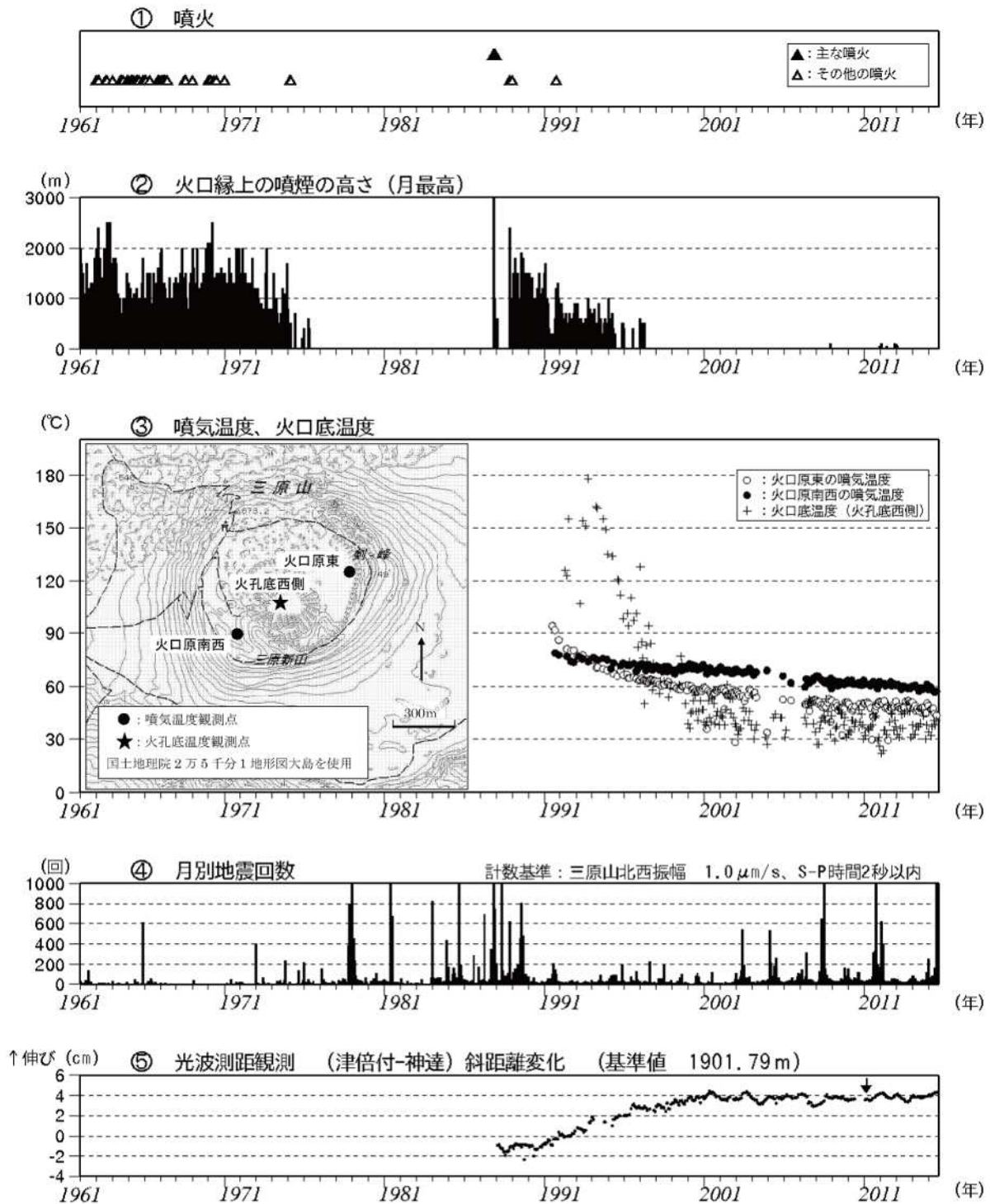
図 1 伊豆大島 長期間の火山活動経過図 (1961 年 1 月 ~ 2014 年 8 月 31 日) 1991 年 12 月 18 日までは火口縁上 130m 以上、2002 年 2 月 28 日までは火口縁上 300m 以上の噴煙の高さを観測していました。
