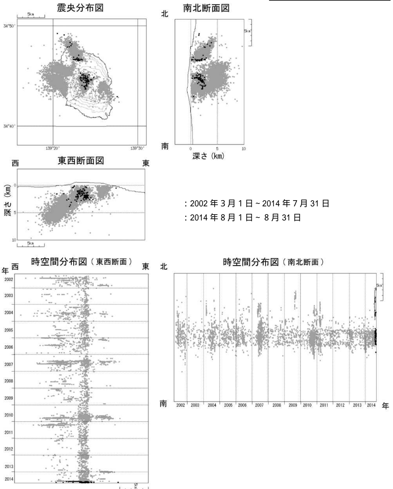
図4 伊豆大島 震源分布図(2002年3月1日~2014年8月31日)
