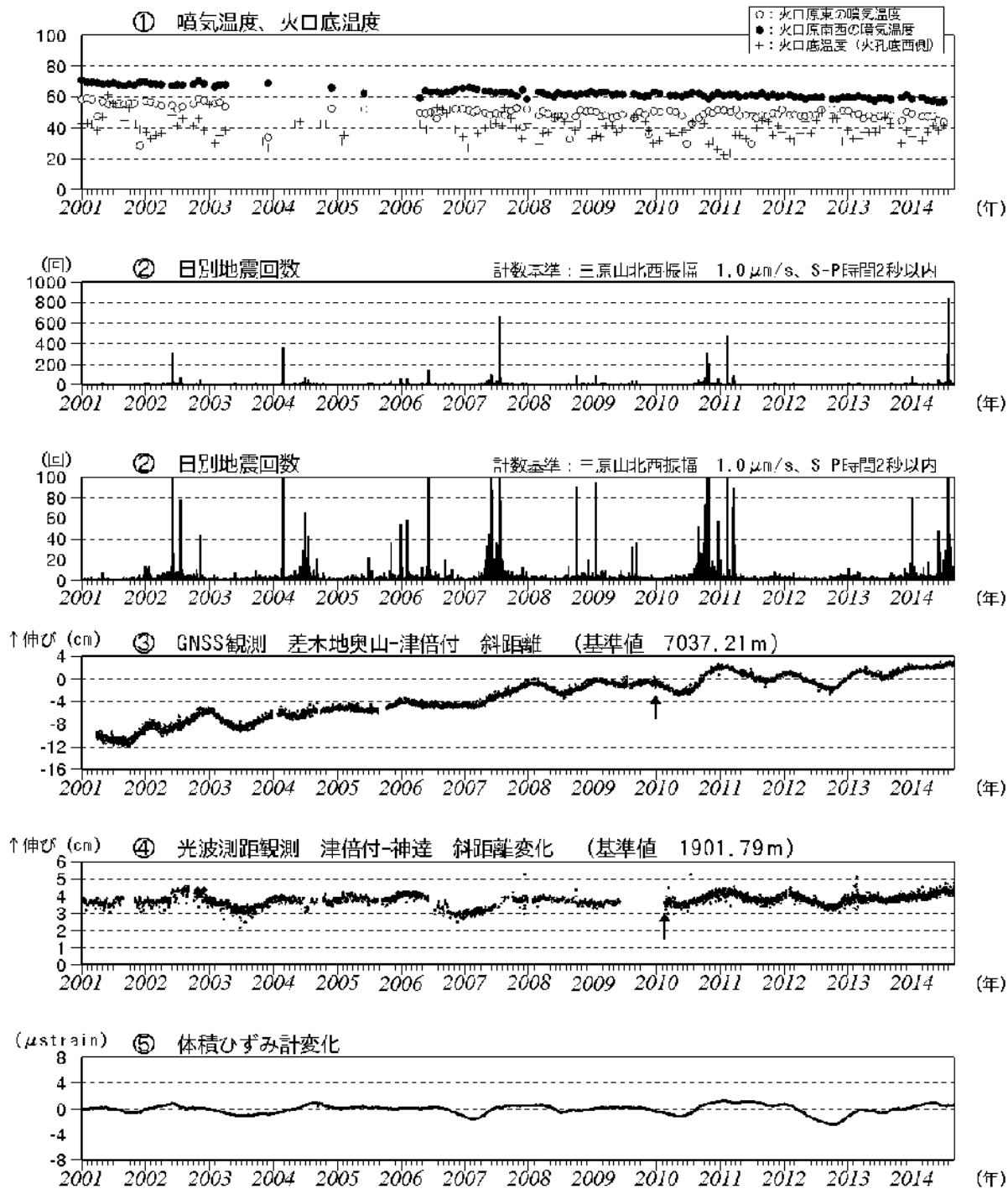
図2 伊豆大島 最近の火山活動経過図（2001年1月～2014年8月31日）
