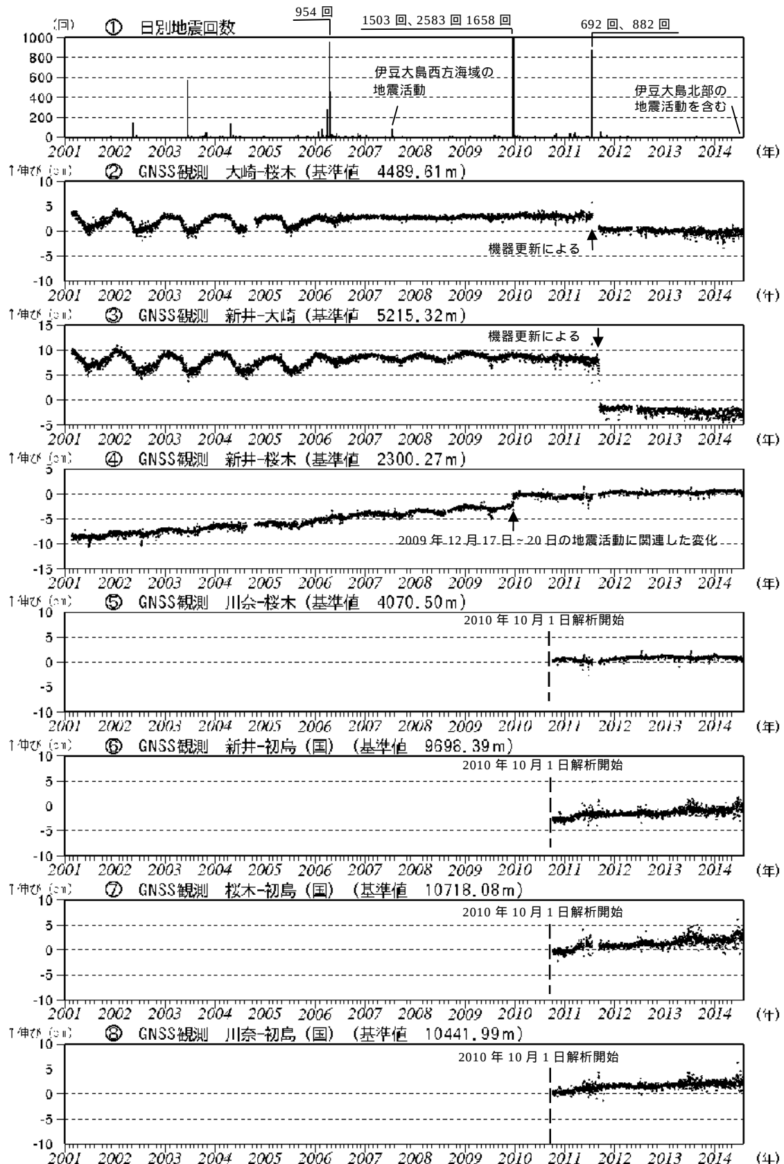
図3 伊豆東部火山群 火山活動経過図（2001年1月～2014年7月）
