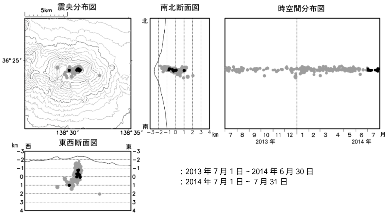
図6 浅間山 震源分布図(2013年7月1日～2014年7月31日)
