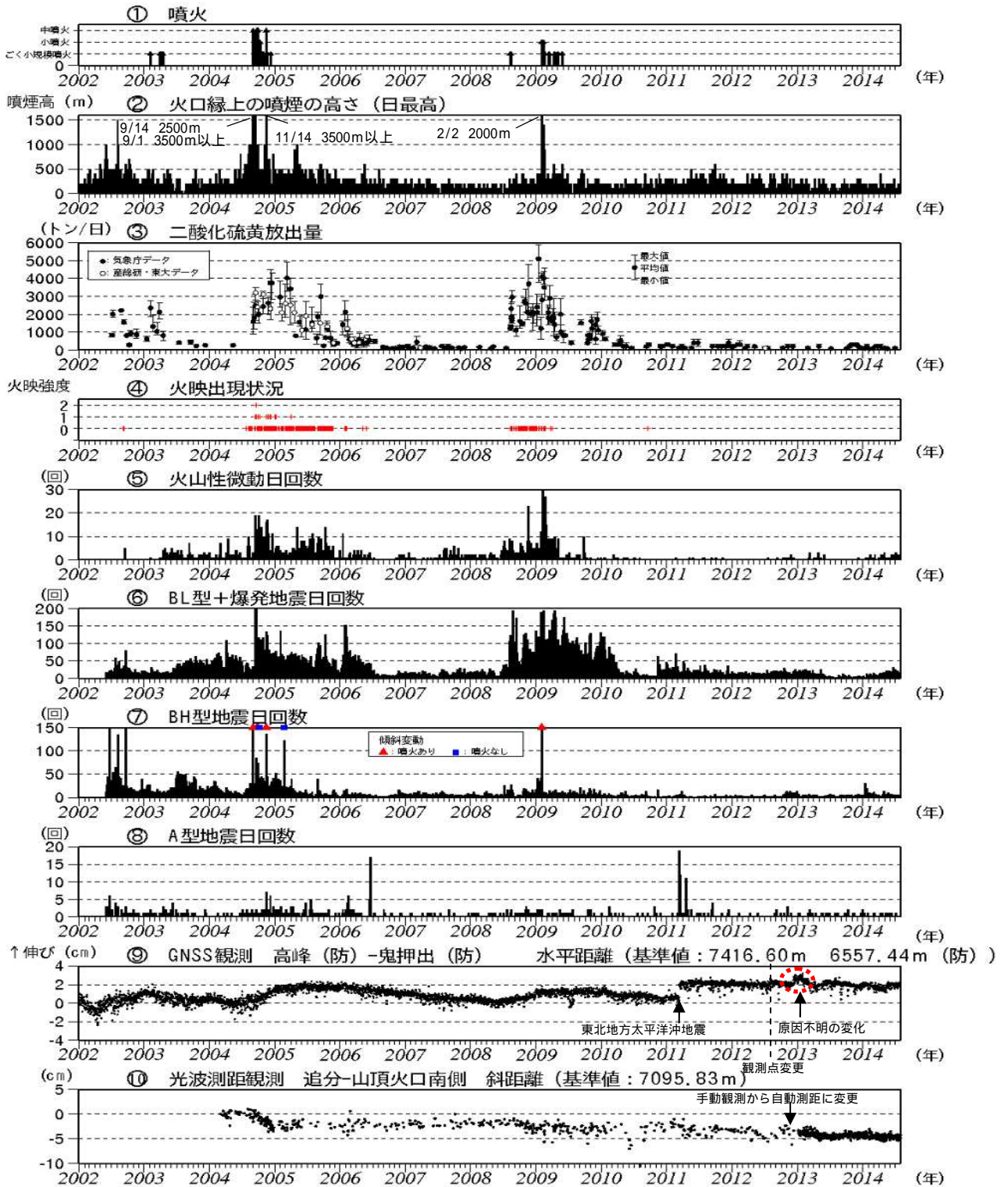
図5 浅間山 火山活動経過図(2002年1月1日~2014年7月31日)
