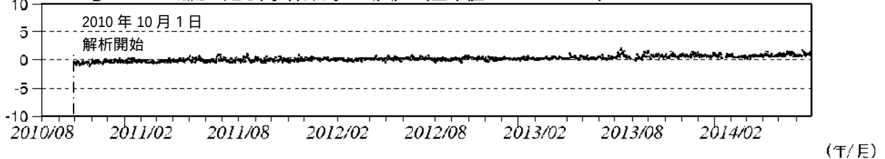
図 3 神津島 火山活動経過図(2010 年 8 月 2 日～2014 年 6 月 30 日)
