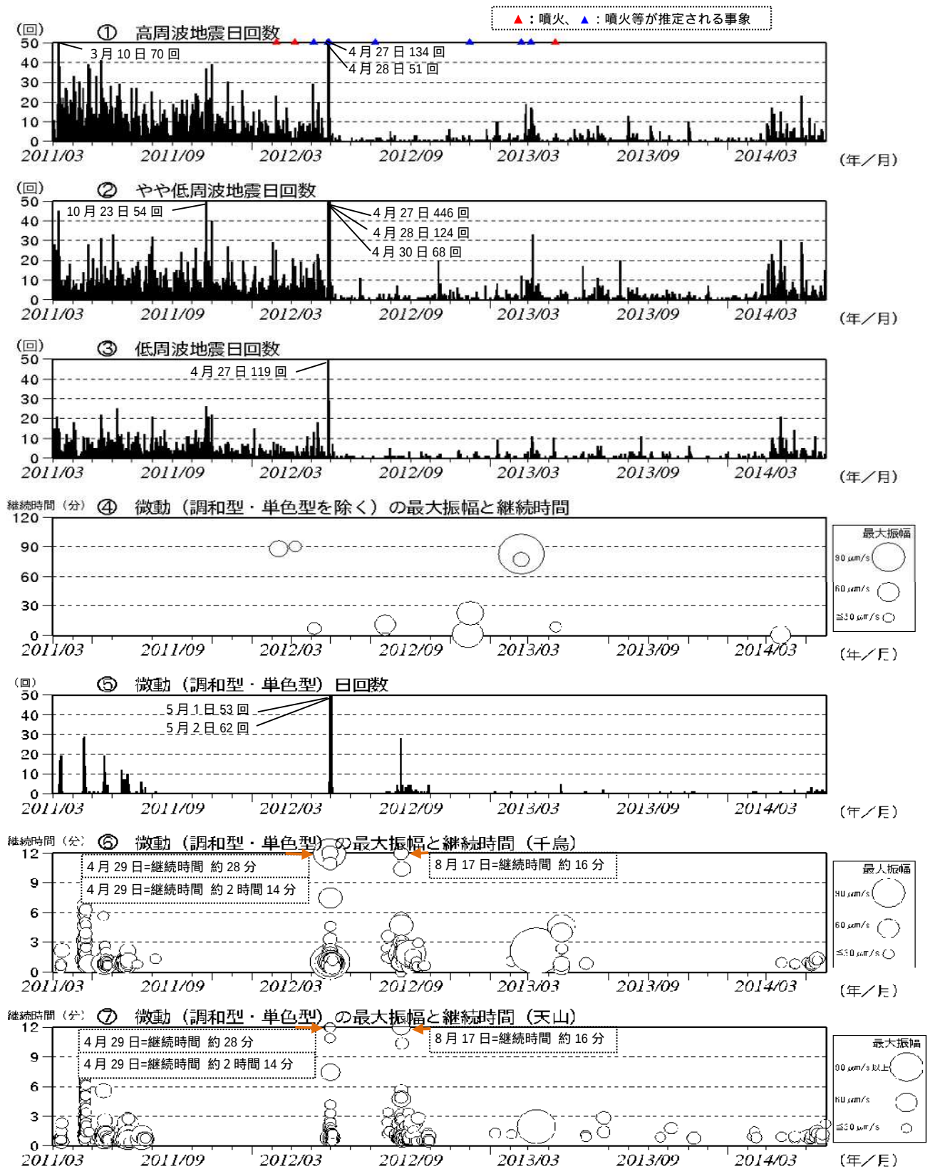
図5 硫黄島 火山活動経過図（2011年3月8日～2014年5月31日）
