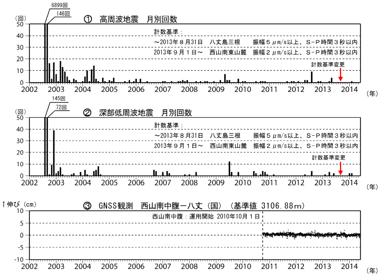
図2 八丈島 火山活動の経過図(2002年8月13日~2014年5月31日)
