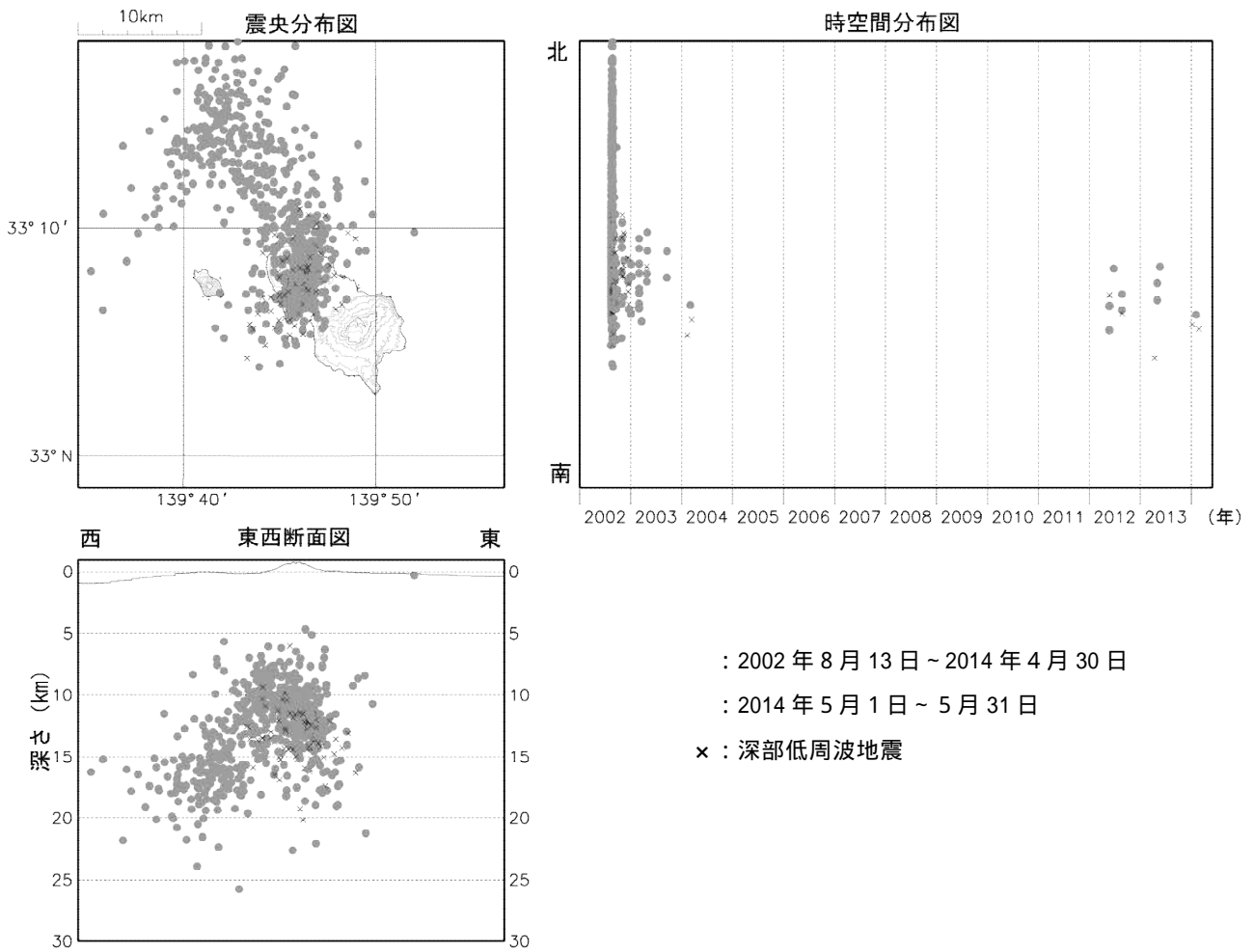
図3 八丈島 震源分布図(2002年8月13日~2014年5月31日) 今期間、八丈島付近に震源が決定された高周波地震及び深部低周波地震はありませんでした。
