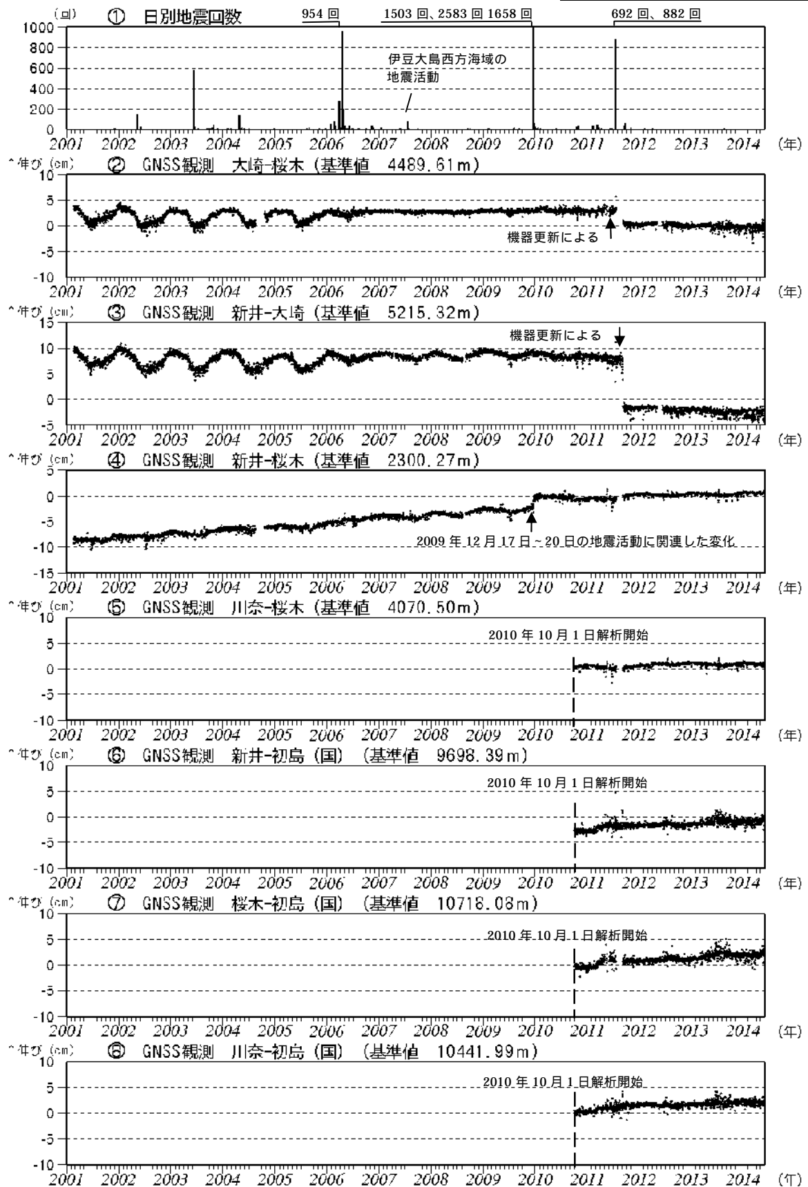
図3 伊豆東部火山群 最近の火山活動経過図(2001年1月~2014年5月)
