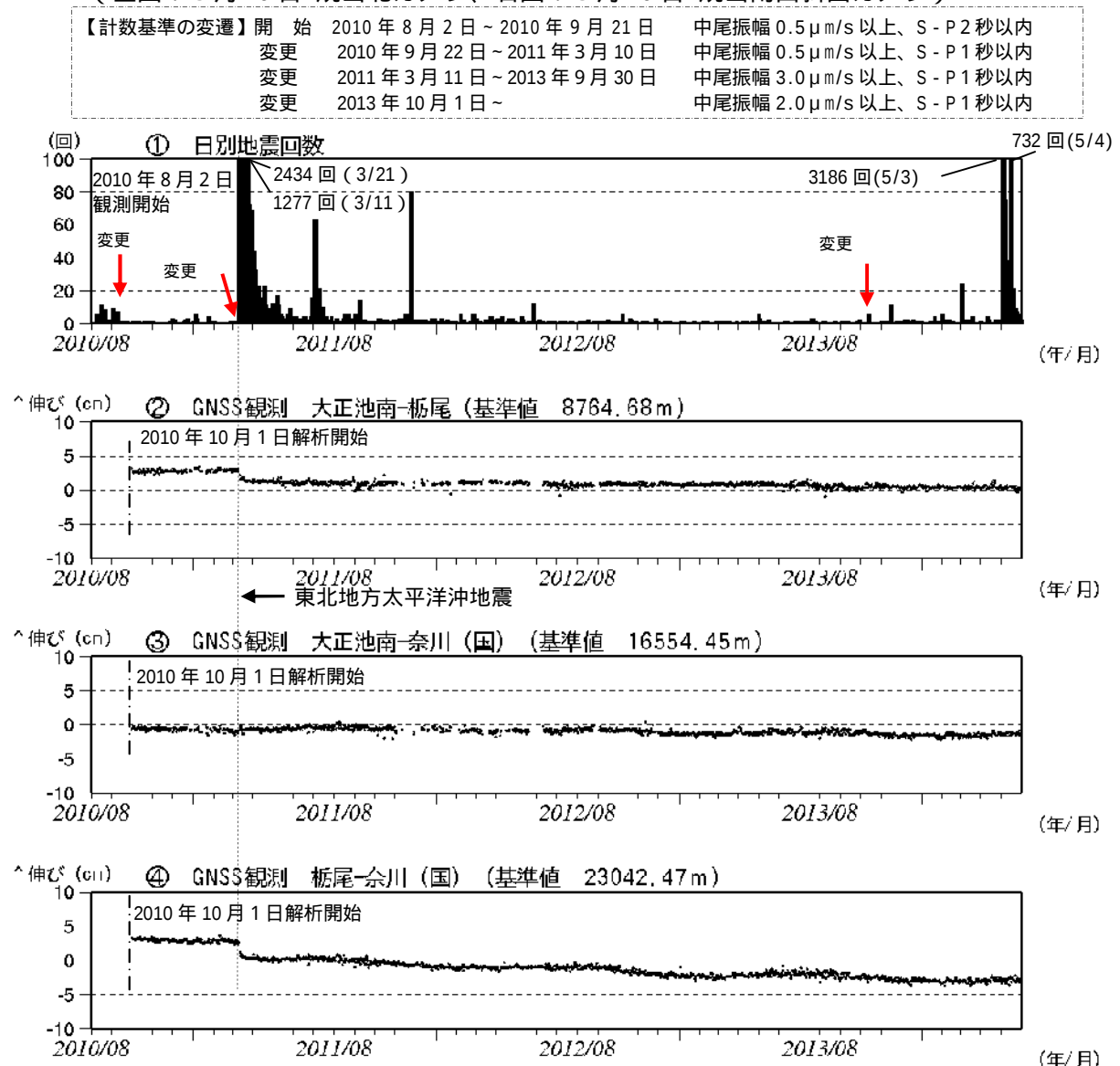
図 3 焼岳 火山活動経過図（2010年 8 月 2 日～2014年 5 月31日）
