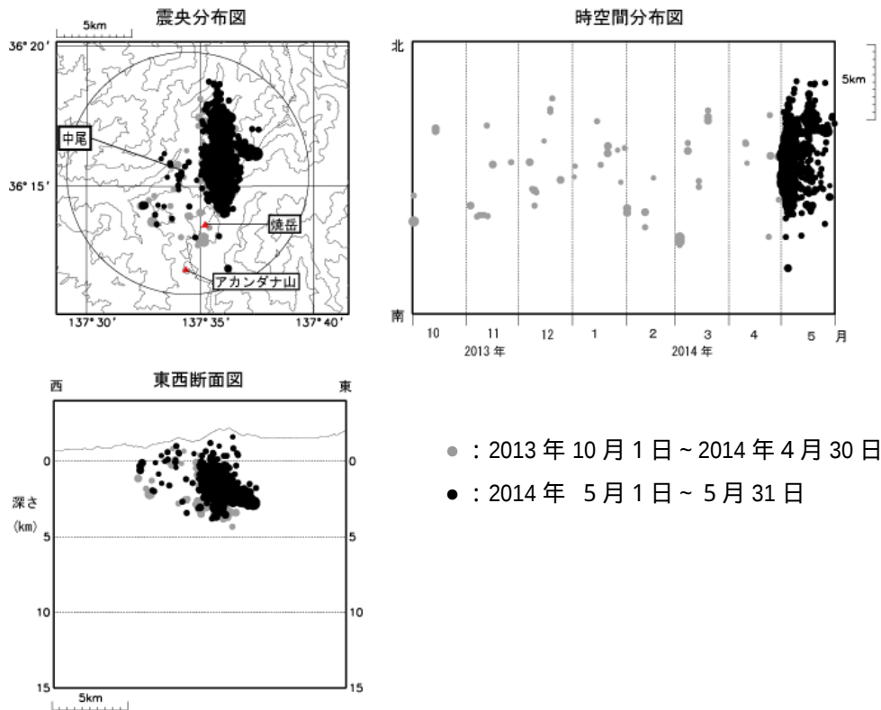
図 4 焼岳 震源分布図（2013 年 10 月 1 日～2014 年 5 月 31 日）
