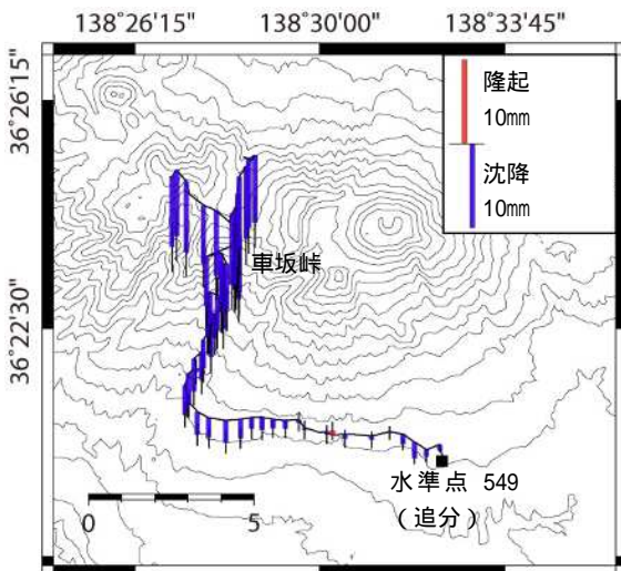
図 6 浅間山 車坂峠・高峰水準測量路線の位置と上下変動(2013年6月から2014年5月の比較)
