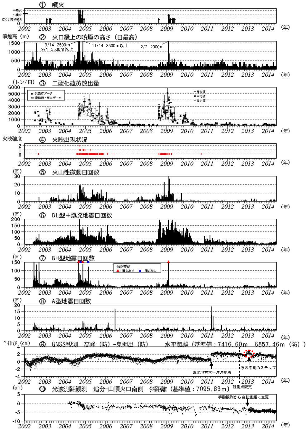
図3 浅間山 最近の火山活動経過図 (2002年1月1日~2014年5月31日)
