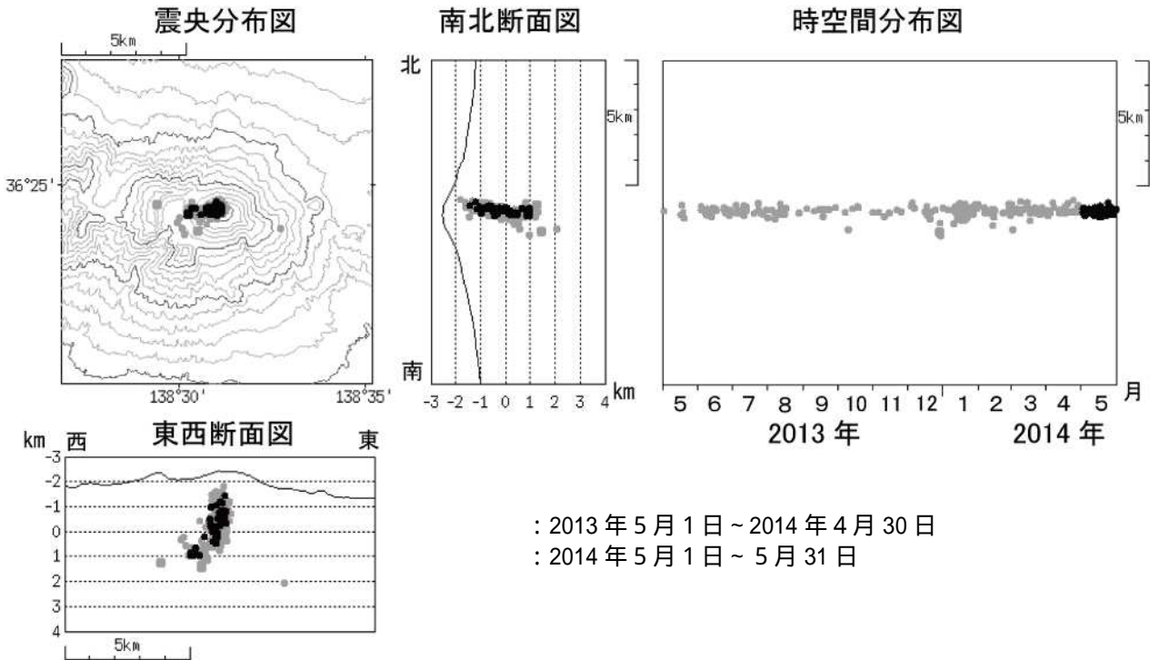
図 4 浅間山 震源分布図 (2013 年 5 月 1 日 ~ 2014 年 5 月 31 日)
