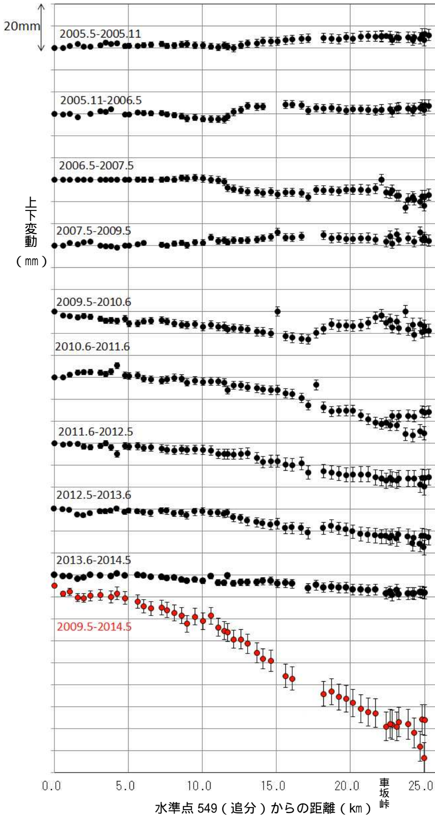
図7 浅間山 水準測量による各期間の上下変動 黒：各測量期間の上下変動、赤：2009年5月から2014年5月の積算の上下変動
