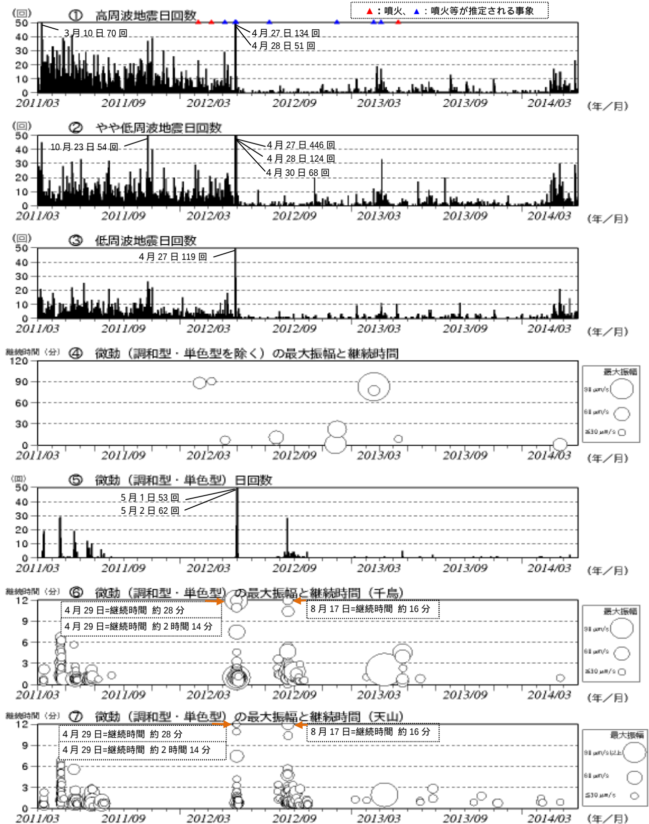
図5 硫黄島 火山活動経過図（2011年3月8日～2014年4月30日）
