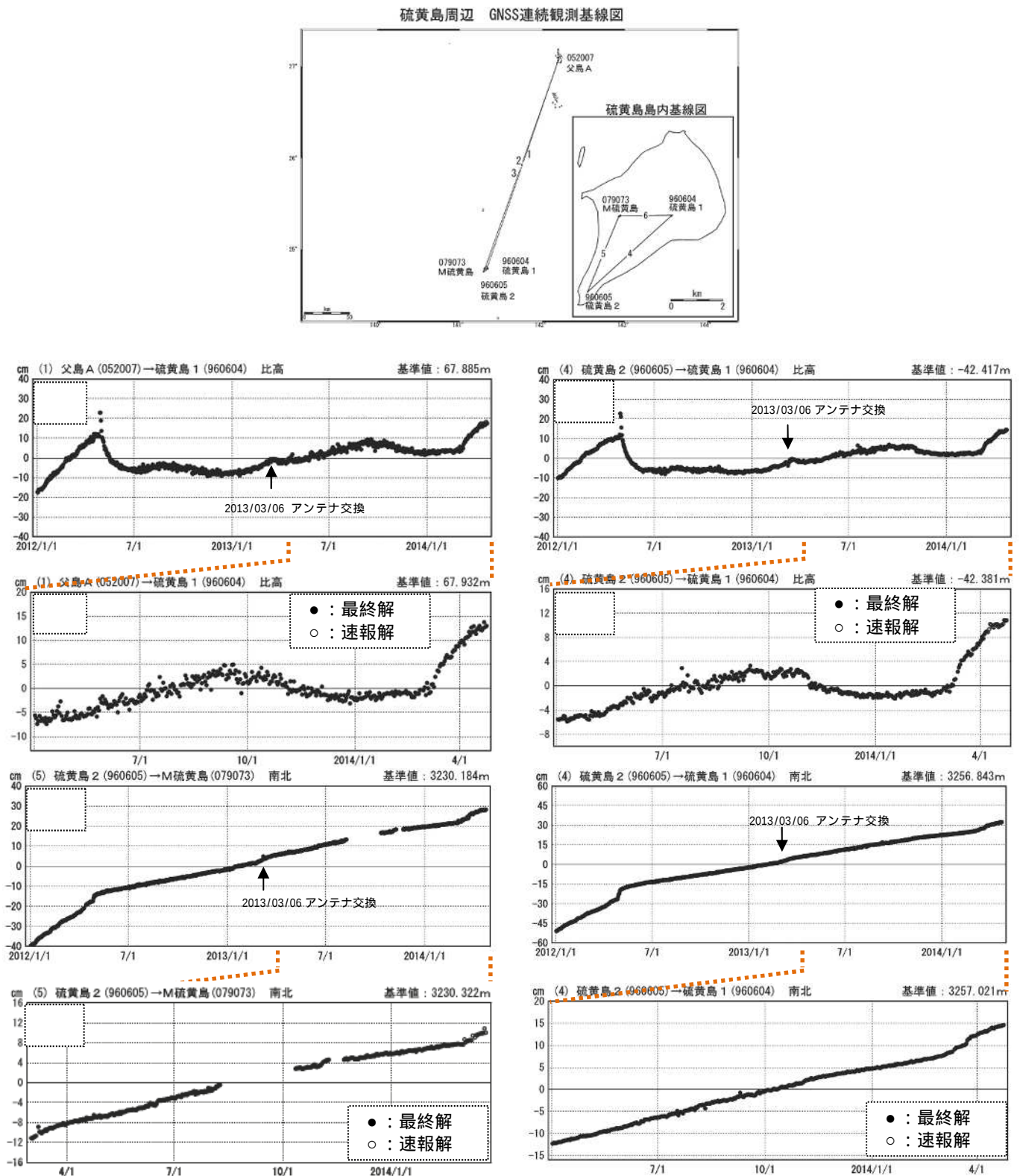
図 6 硫黄島 国土地理院による地殻変動観測結果 2)
