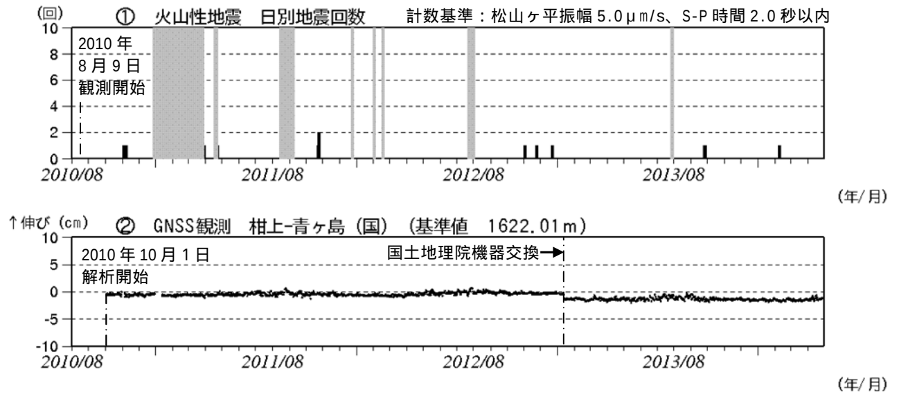
図2 青ヶ島 火山活動経過図（2010年8月9日～2014年4月30日）
