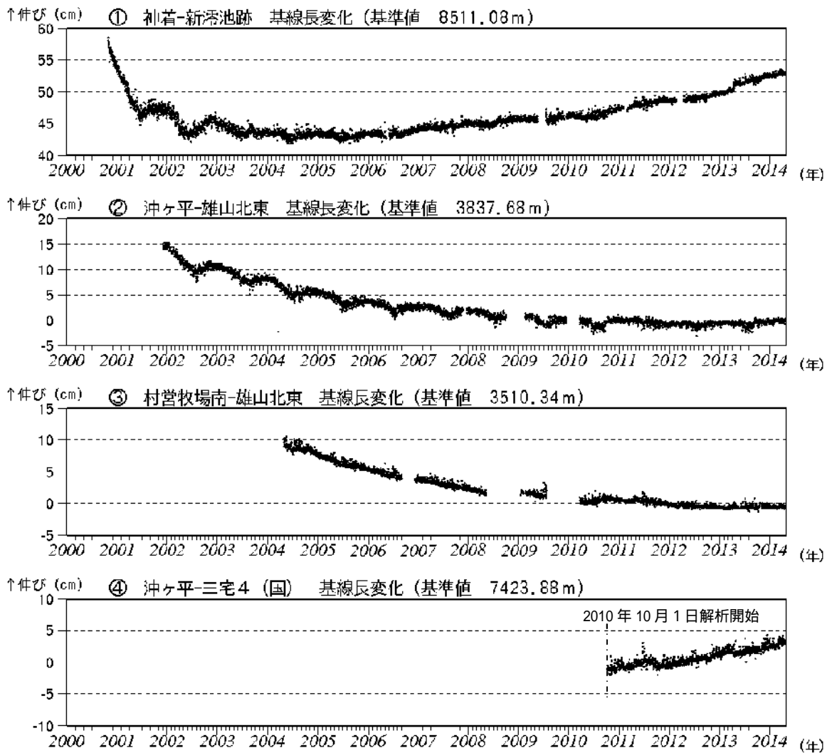
図 5 三宅島 GNSS 連続観測結果(2000 年 1 月~2014 年 4 月) (国): 国土地理院
