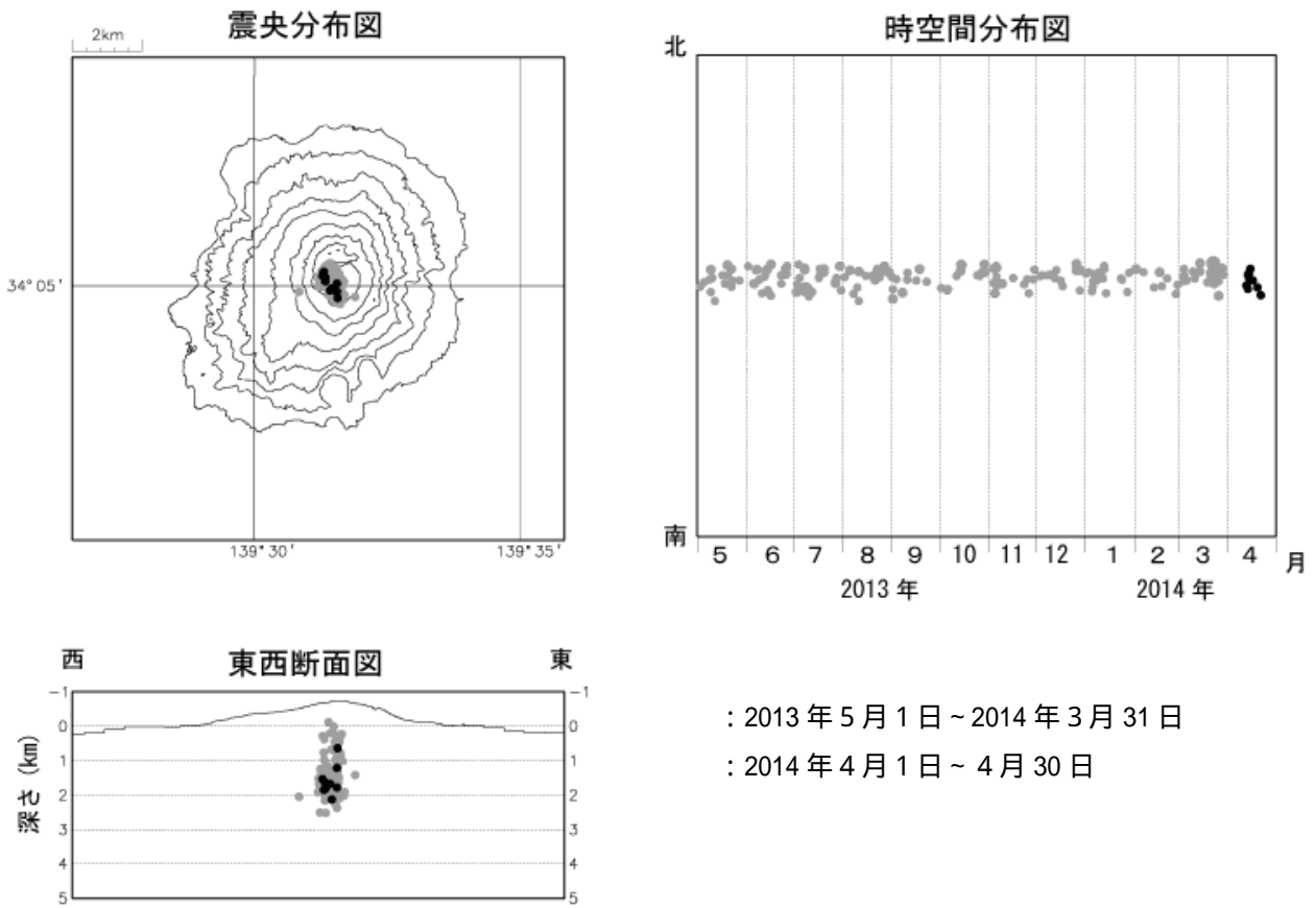
図6 三宅島 震源分布図(2013年5月1日～2014年4月30日)
