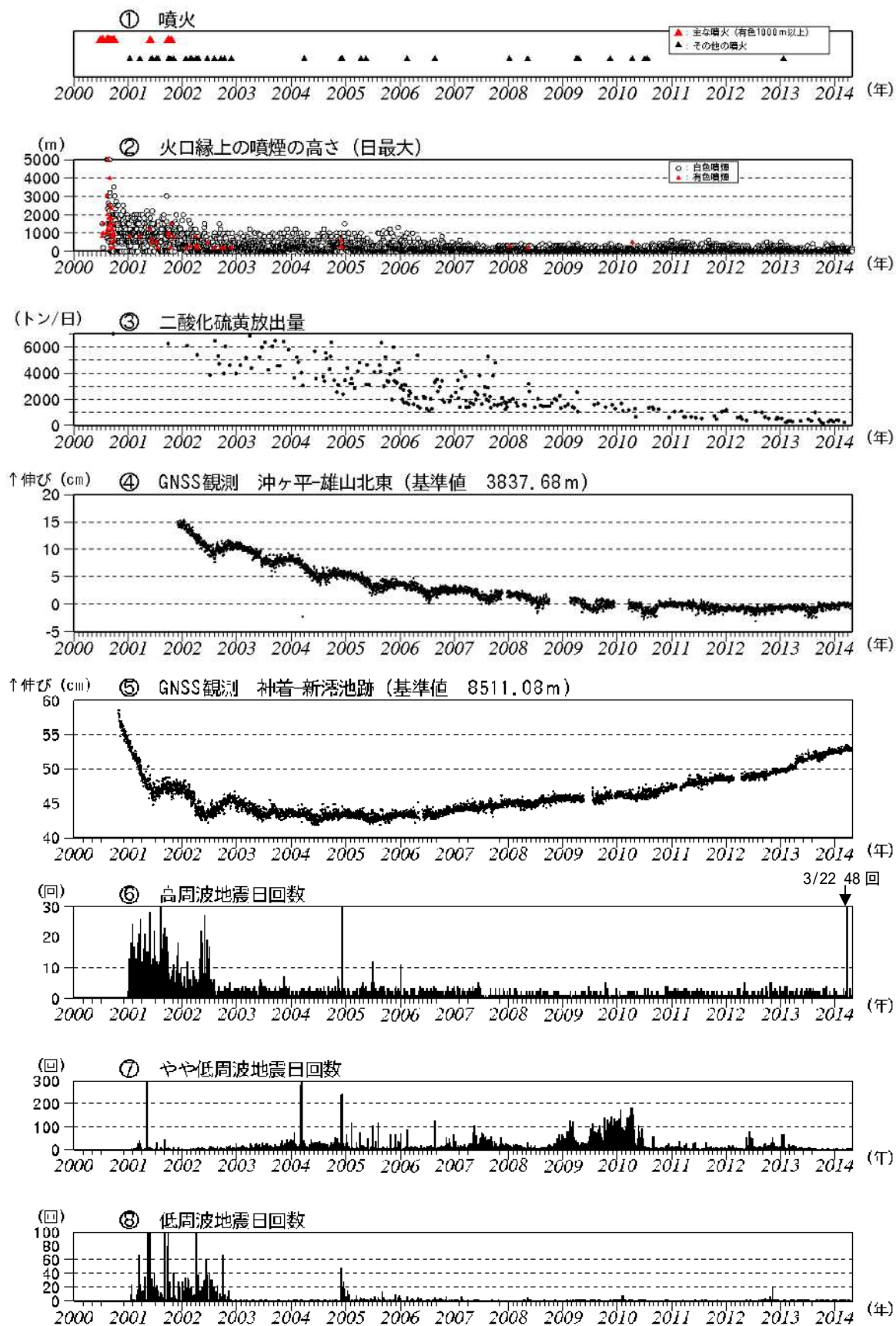
図4 三宅島 最近の火山活動の経過図（2000年1月～2014年4月）
