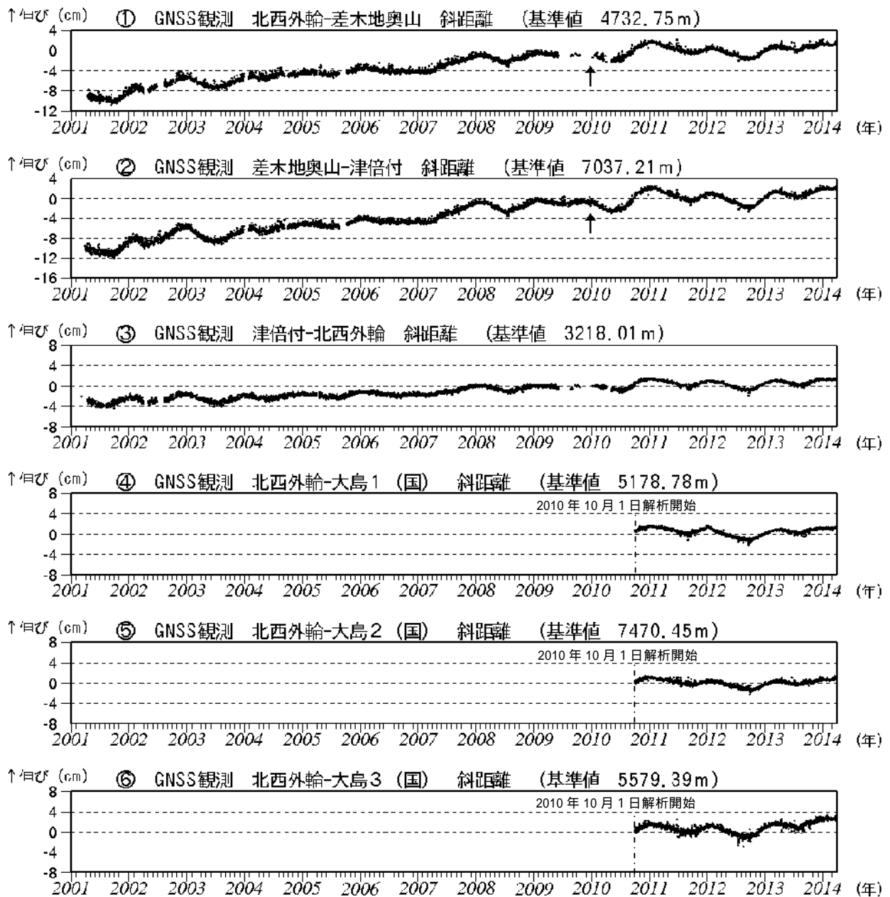
図3 伊豆大島 GNSS連続観測による基線長変化(2001年1月~2014年3月31日)(国): 国土地理院
