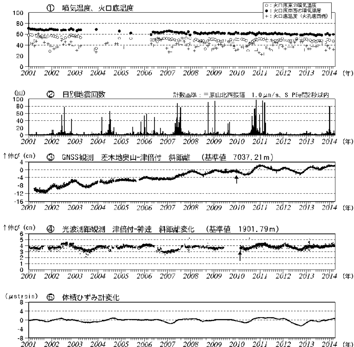
図2 伊豆大島 最近の火山活動経過図（2001年1月～2014年3月31日）
