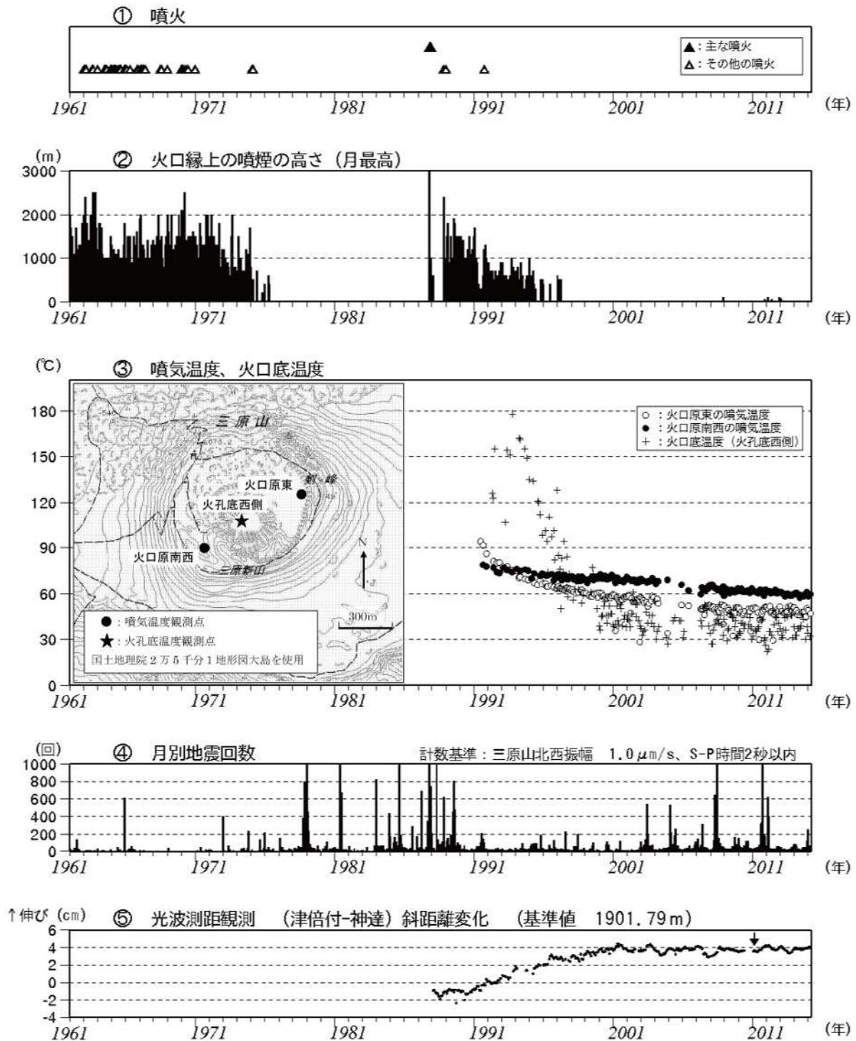
図 1 伊豆大島 長期間の火山活動経過図 (1961 年 1 月 ~ 2014 年 3 月 31 日) 1991 年 12 月 18 日までは火口縁上 130m 以上、2002 年 2 月 28 日までは火口縁上 300m 以上の噴煙の高さを観測していました。
