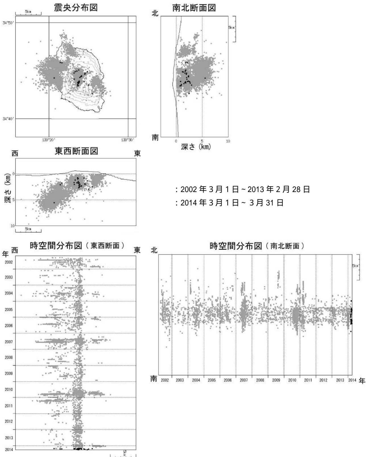
図7 伊豆大島 震源分布図（2002年3月1日～2014年3月31日）
