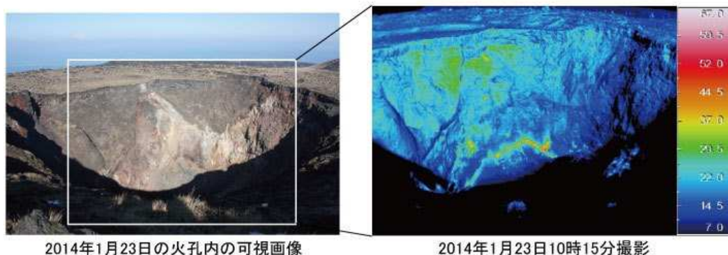
図5 伊豆大島 中央火孔内の状況（左）と地表面温度分布 1) （右）
