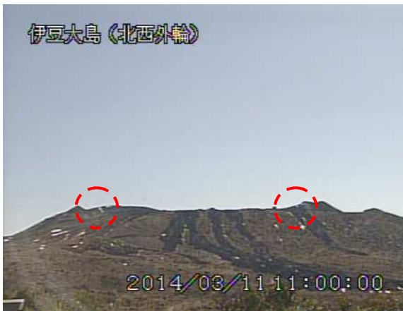
山頂部（3月11日、北西外輪遠望カメラによる） 剣ガ峰付近（3月17日、撮影方向は図6参照） 図4 伊豆大島 三原山山頂部及び山頂火口の状況 破線円内：ごく弱い噴気
