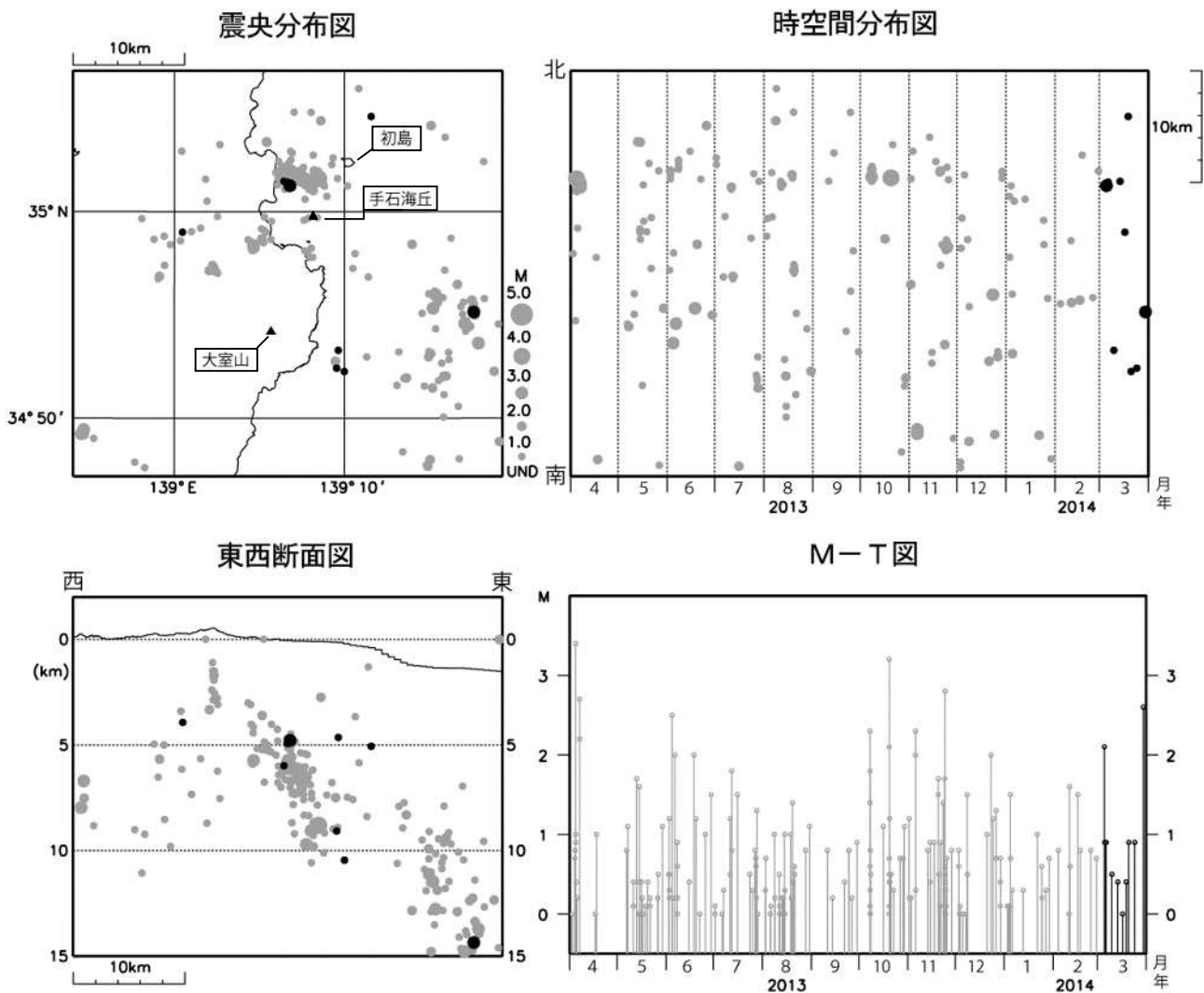
図2 伊豆東部火山群 広域地震観測網による震源分布図(2013年4月1日～2014年3月31日)
