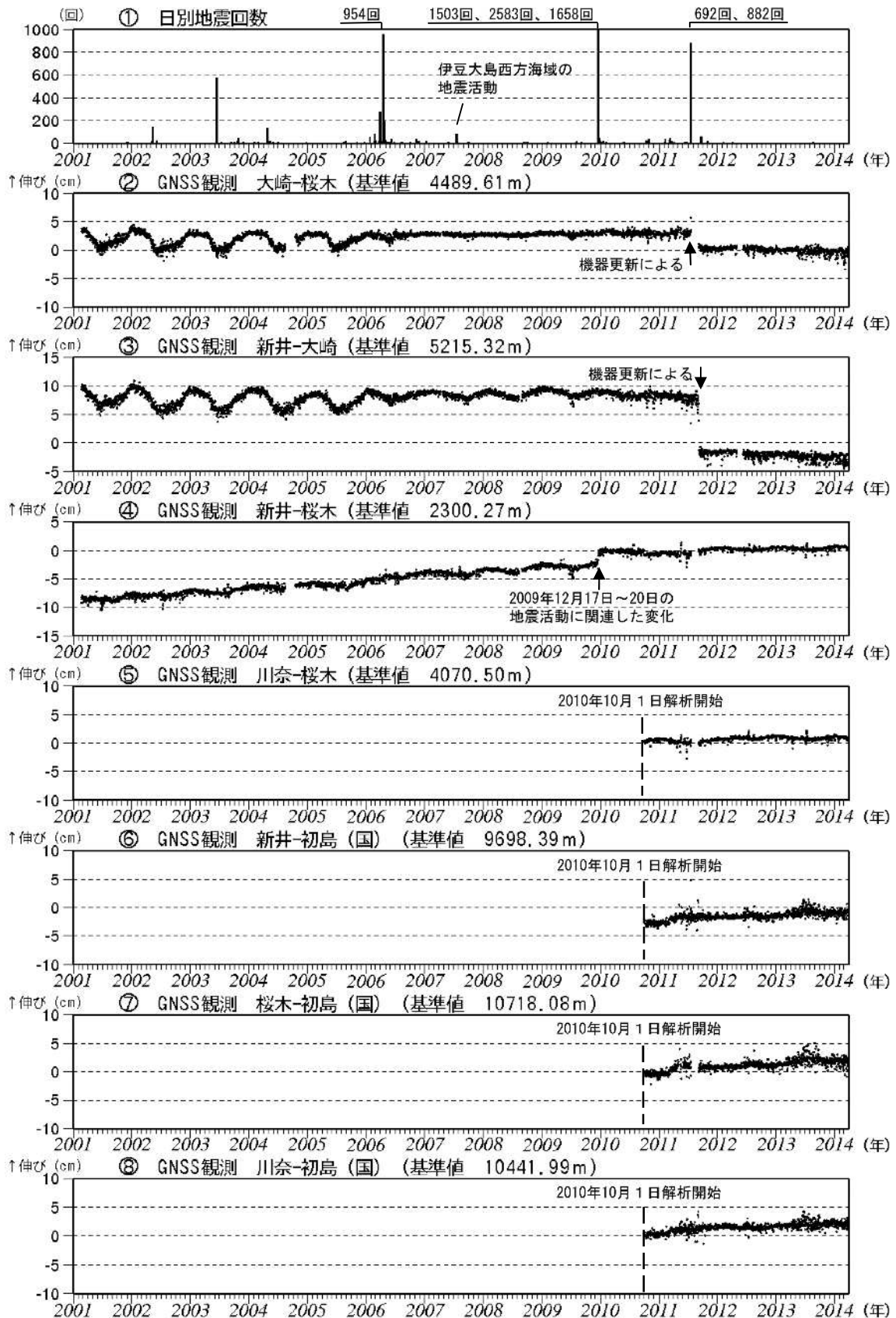
図3 伊豆東部火山群 最近の火山活動経過図(2001年1月~2014年3月)
