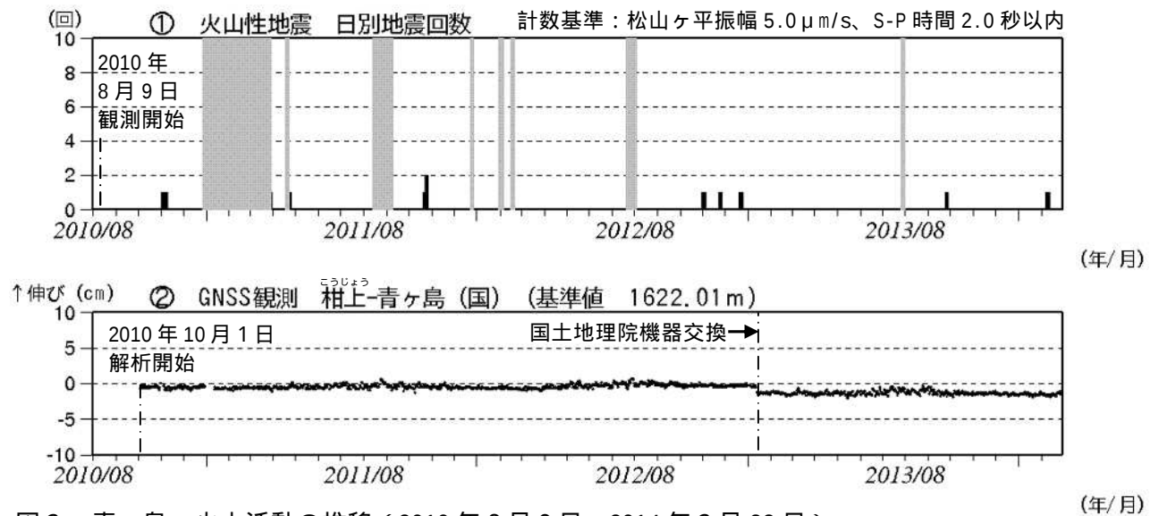
図 2 青ヶ島 火山活動の推移（2010 年 8 月 9 日～2014 年 2 月 28 日）
