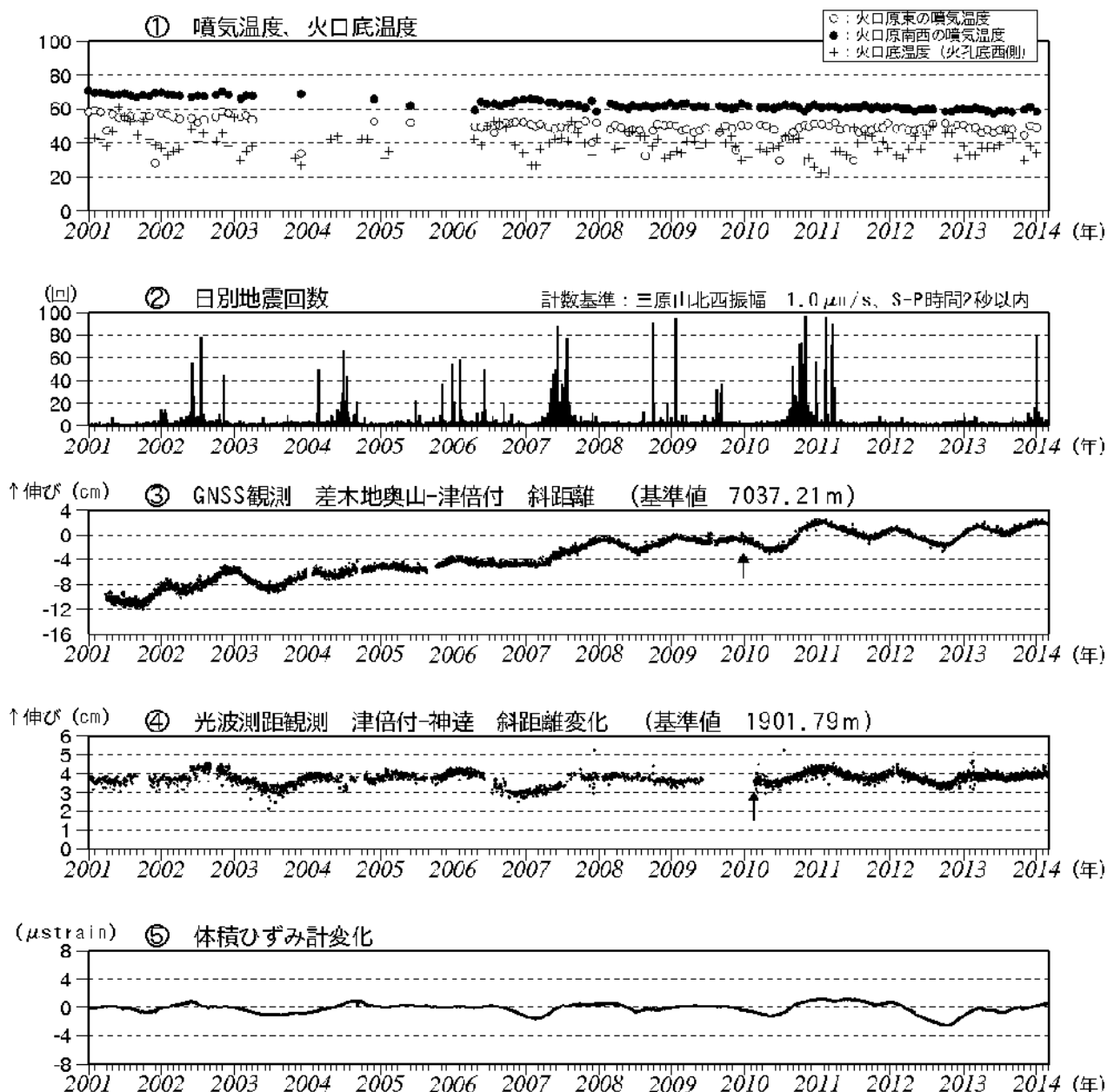
図4 伊豆大島 最近の火山活動経過図（2001年1月～2014年2月28日）
