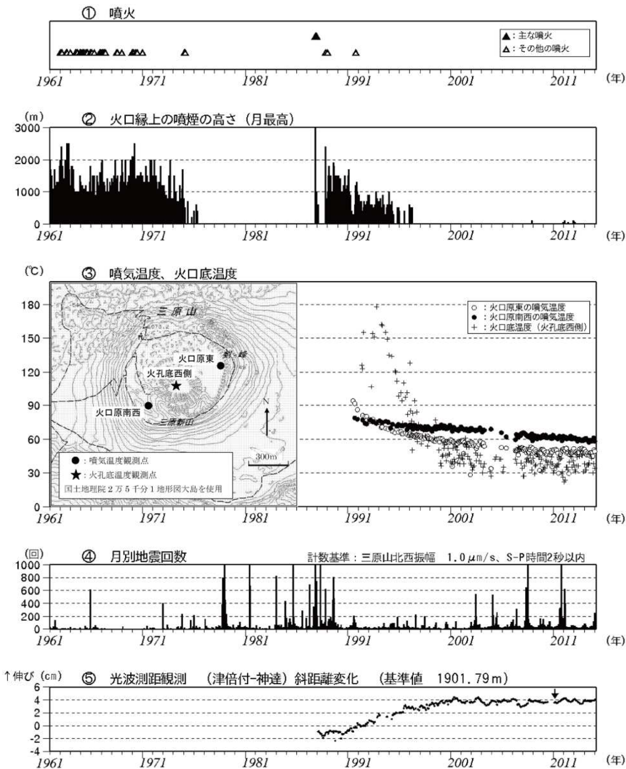
図 3 伊豆大島 長期間の火山活動経過図（1961 年 1 月～2014 年 2 月 28 日） 1991 年 12 月 18 日までは火口縁上 130m 以上、2002 年 2 月 28 日までは火口縁上 300m 以上の噴煙の高さを観測していました。 火口底温度（火口底西側）は赤外放射温度計を用いて離れた場所から測定した値。 噴気温度（火口原東、火口原南西）はサーミスタ温度計を用いて直接測定した値。 地震回数には伊豆大島周辺海域で発生した地震も一部含まれています。 光波距離計 4) による月平均値（観測開始は 1987 年 1 月）。グラフの空白部分は欠測。矢印は機器更新を示します。
