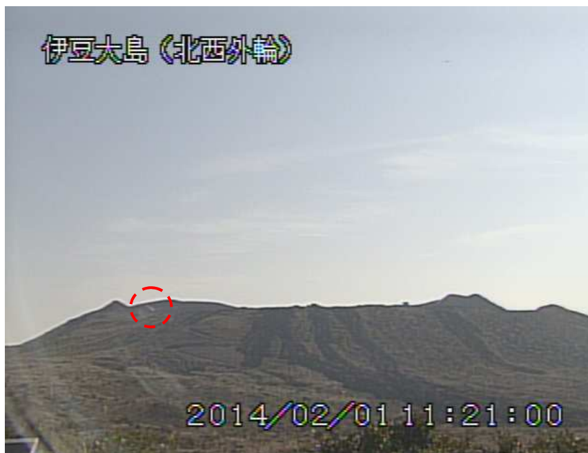
図 2 伊豆大島 三原山山頂部の状況（2月1日、北西外輪遠望カメラによる） 破線円内：ごく弱い噴気
