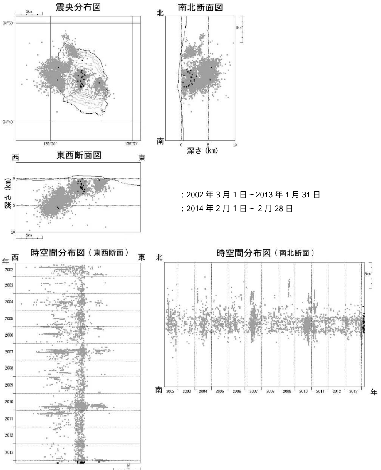
図 6 伊豆大島 震源分布図（2002 年 3 月 1 日 ~ 2014 年 2 月 28 日）
