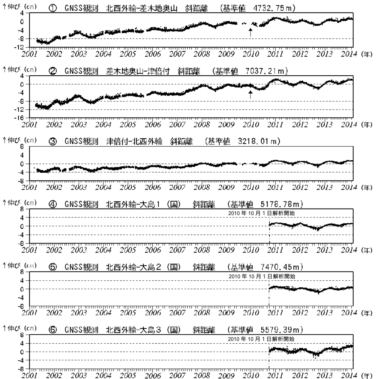
図5 伊豆大島 GNSS連続観測による基線長変化(2001年1月~2014年2月28日)(国): 国土地理院
