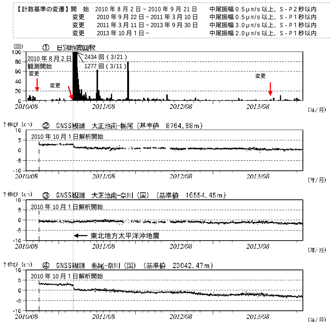
図 3 焼岳 火山活動経過図（2010年 8 月 2 日～2014年 2 月28日）
