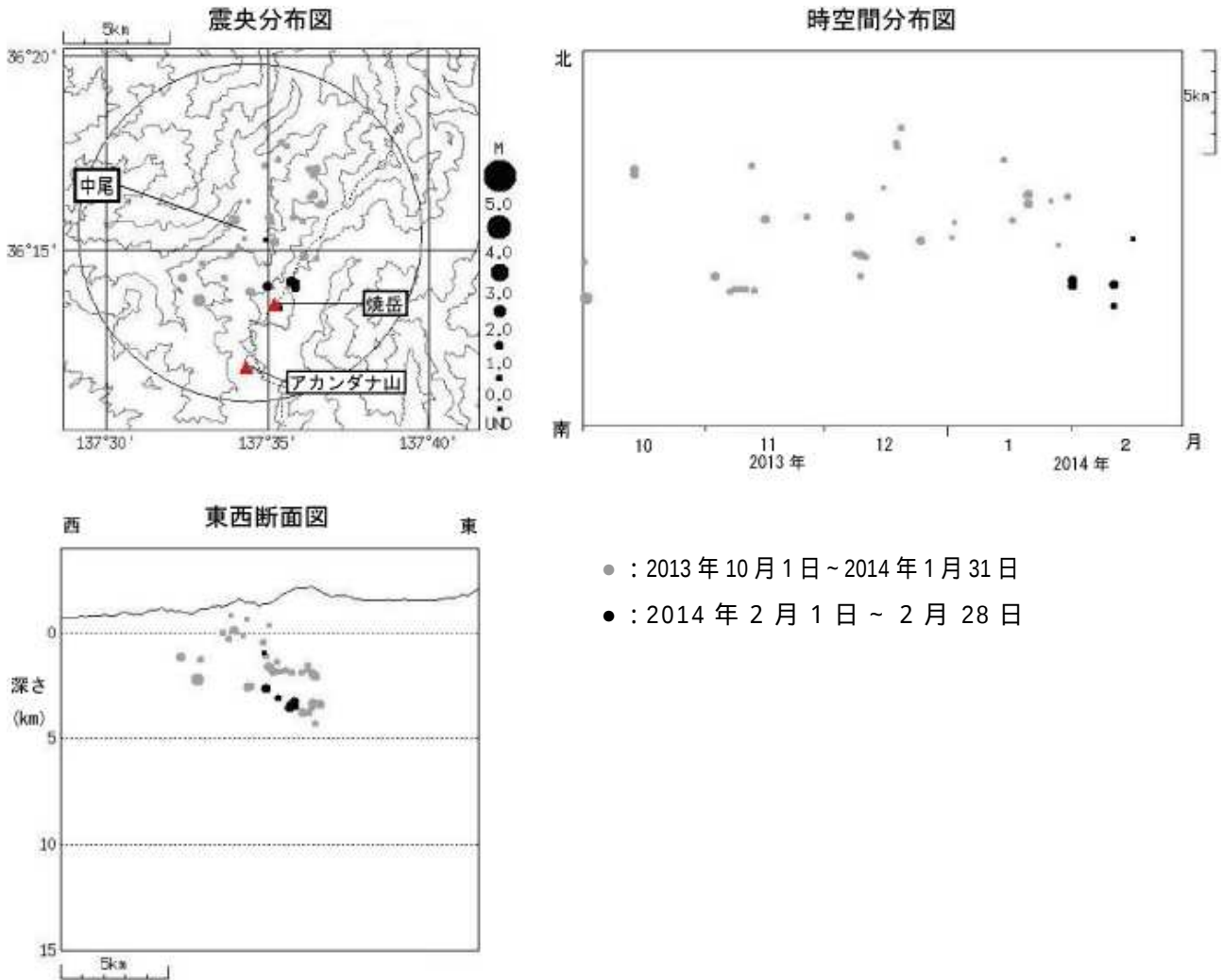
図 4 焼岳 震源分布図（2013 年 10 月 1 日 ~ 2014 年 2 月 28 日）
