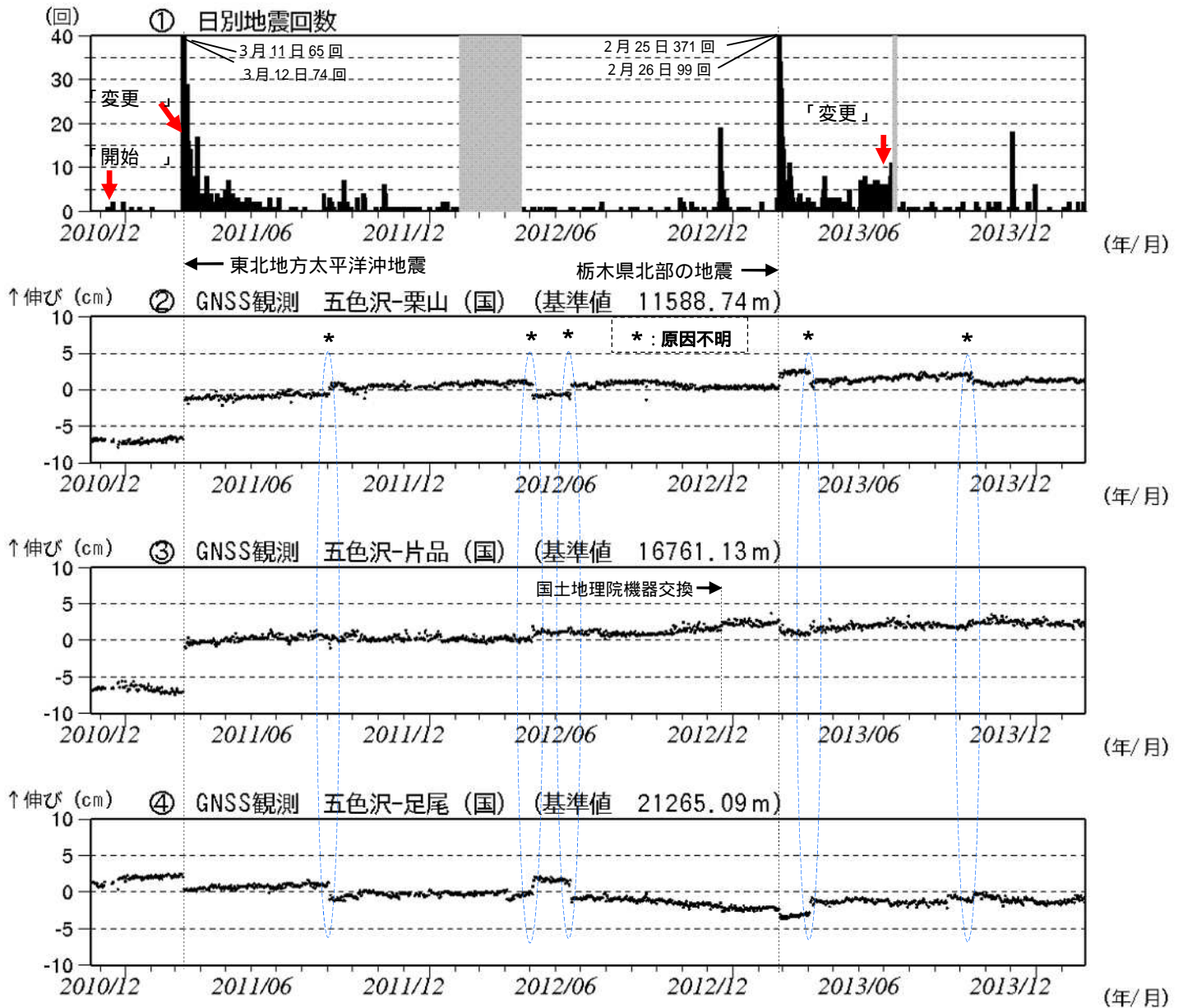
図2 日光白根山 火山活動経過図(2010年11月20日~2014年2月28日)
