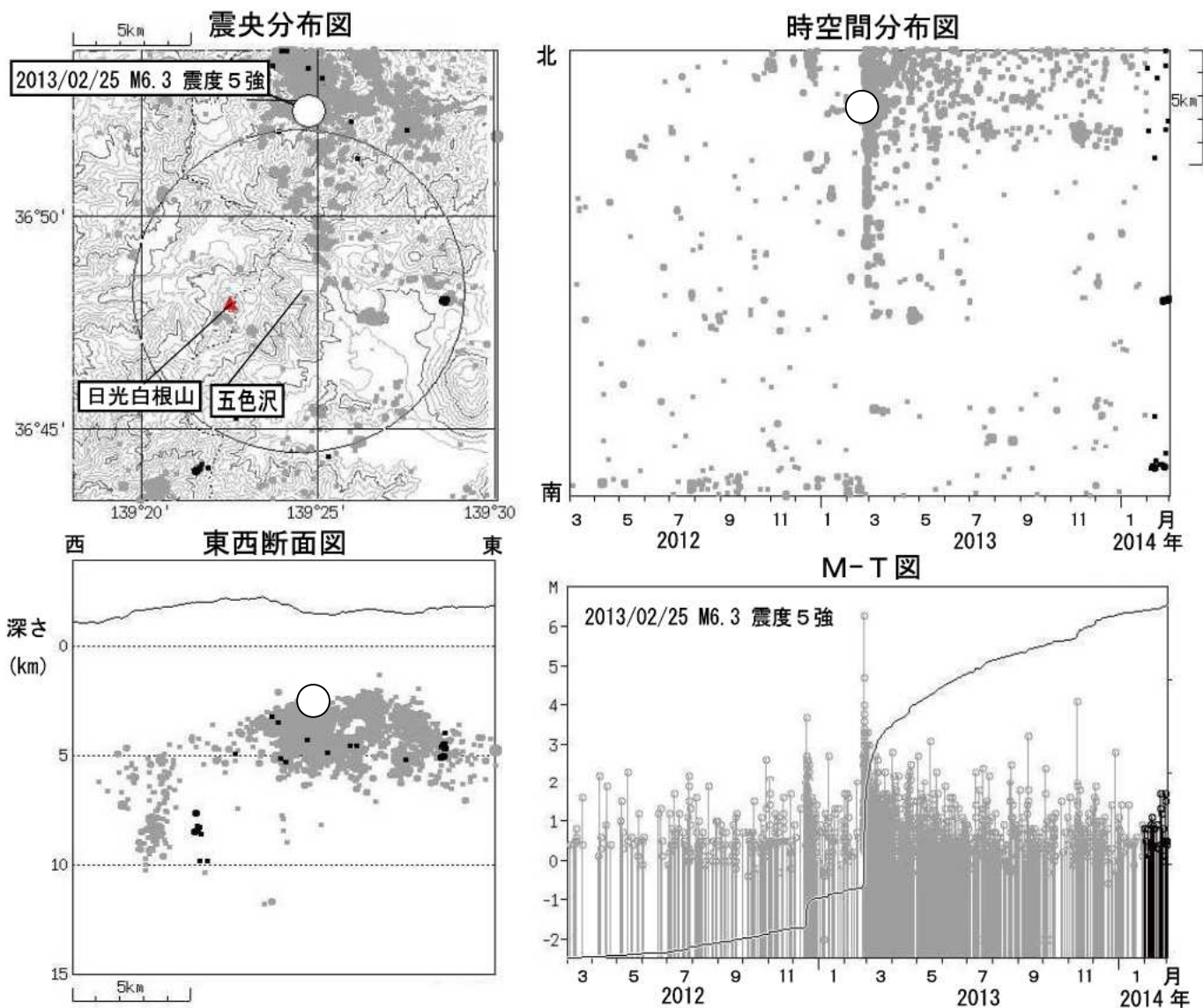
図3 日光白根山 広域地震観測網による山体・周辺の地震活動(2012年3月1日～2014年2月28日) : 2012年3月1日～2014年1月31日 : 2014年2月1日～2月28日 ・2013年2月25日に発生した栃木県北部の地震（M6.3：図中白抜きのシンボル）による余震活動は、低下しました。 ・震央分布図中の円は図2 - の計数対象地震（五色沢でS - P時間1秒以内）のおよその範囲を示します。 ・M（マグニチュード）は地震の規模を表します。 ・図中の震源要素は一部暫定値が含まれており、後日変更することがあります。 ・日光白根山付近を震源とする地震の発生は少なく、地震活動は静穏に経過しました。
