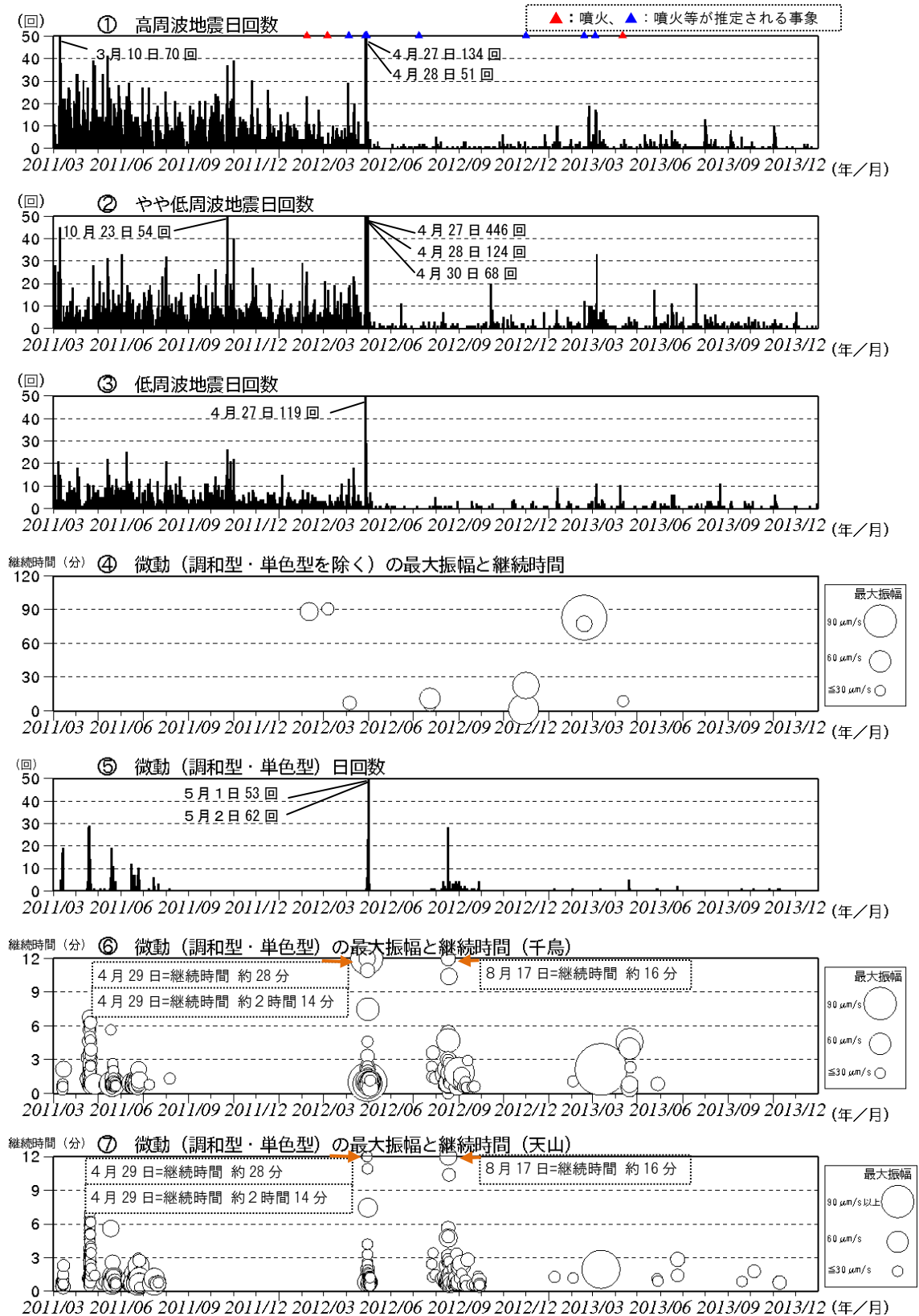
図5 硫黄島 火山活動経過図(2011年3月8日～2013年12月31日)
