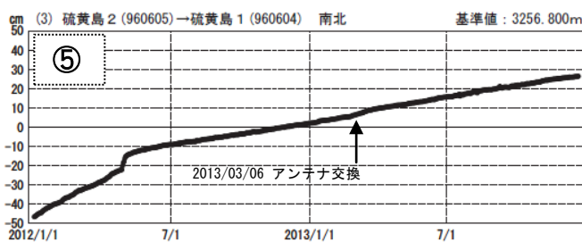
図 6 硫黄島 国土地理院による地殻変動観測結果 1)
