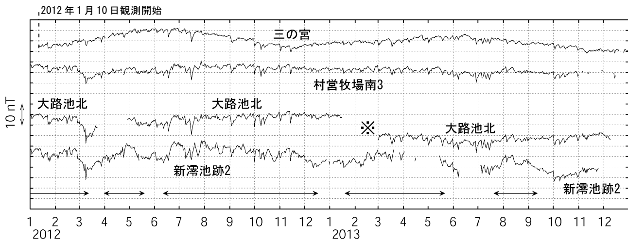
図4 三宅島 全磁力連続観測による全磁力値の変化 (2012 年 1 月～2013 年 12 月) 基準点 : 雄山北東
