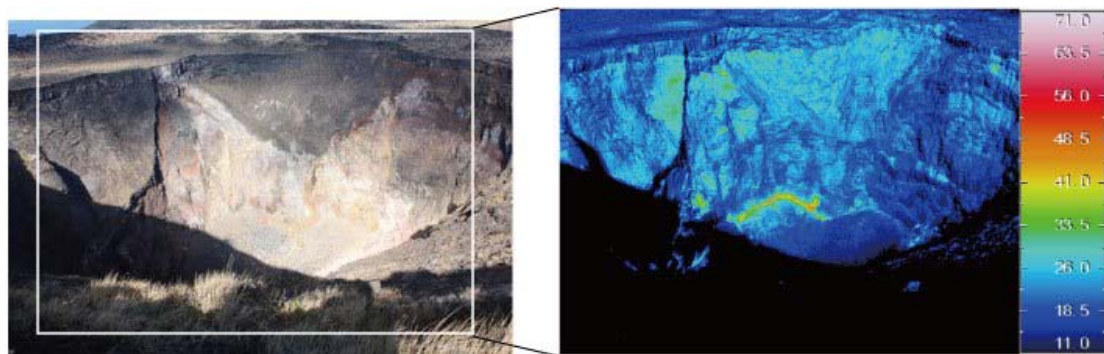
2013年12月16日の火口内の可視画像
