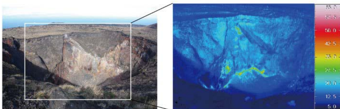
2013年11月27日の火口内の可視画像
