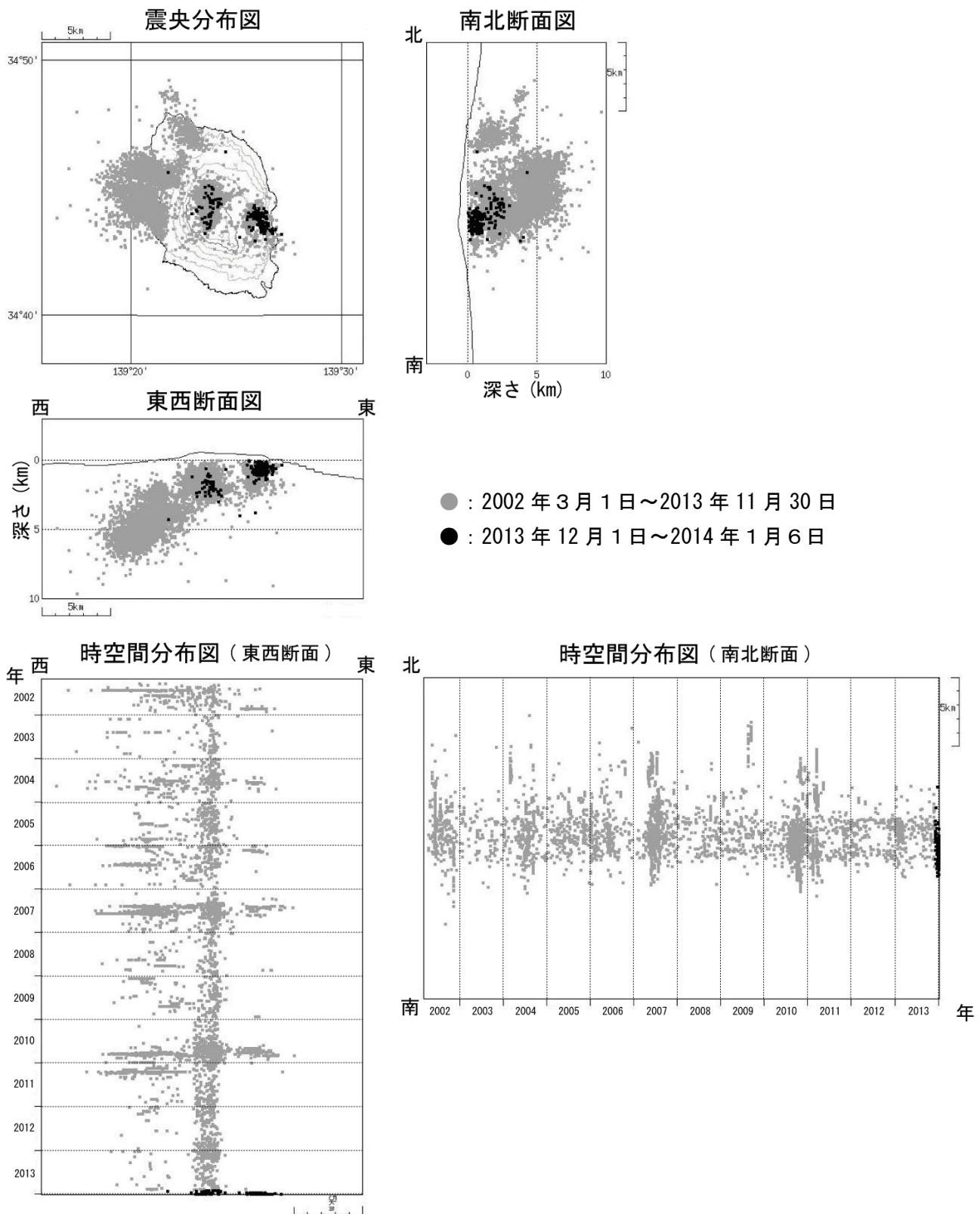
図 8 伊豆大島 震源分布図 (2002 年 3 月 1 日 ~ 2014 年 1 月 6 日)
