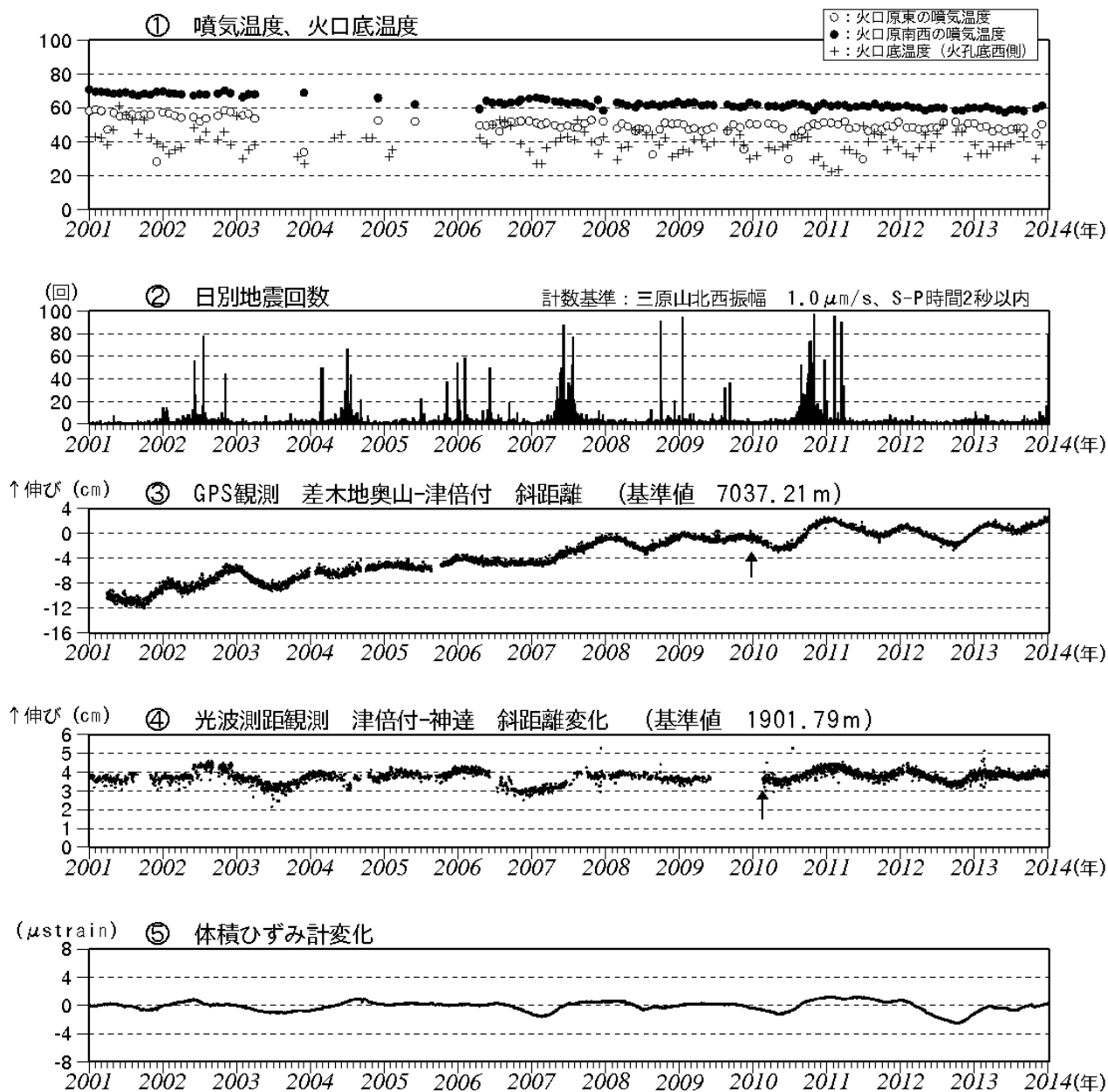
図3 伊豆大島 最近の火山活動経過図 (2001年1月～2014年1月6日)
