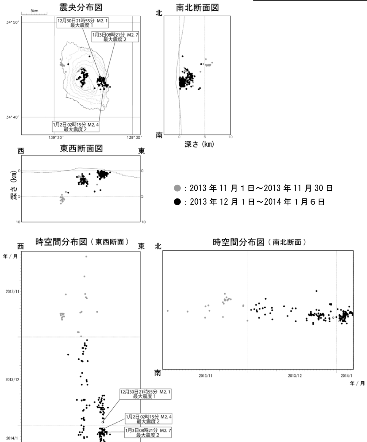
図 9 伊豆大島 震源分布図 (2013 年 11 月 1 日 ~ 2014 年 1 月 6 日)
