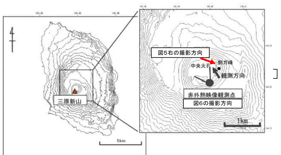
図6 伊豆大島 中央火口内の状況 (左) と地表面温度分布 1) (右)
