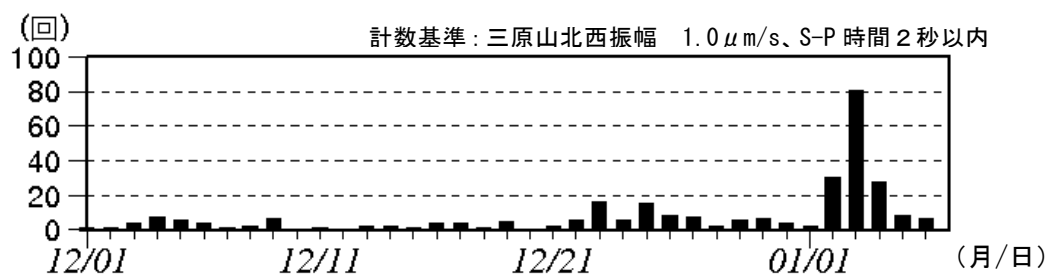
図 10 伊豆大島 日別地震回数 (2013 年 12 月 1 日 ~ 2014 年 1 月 6 日)
