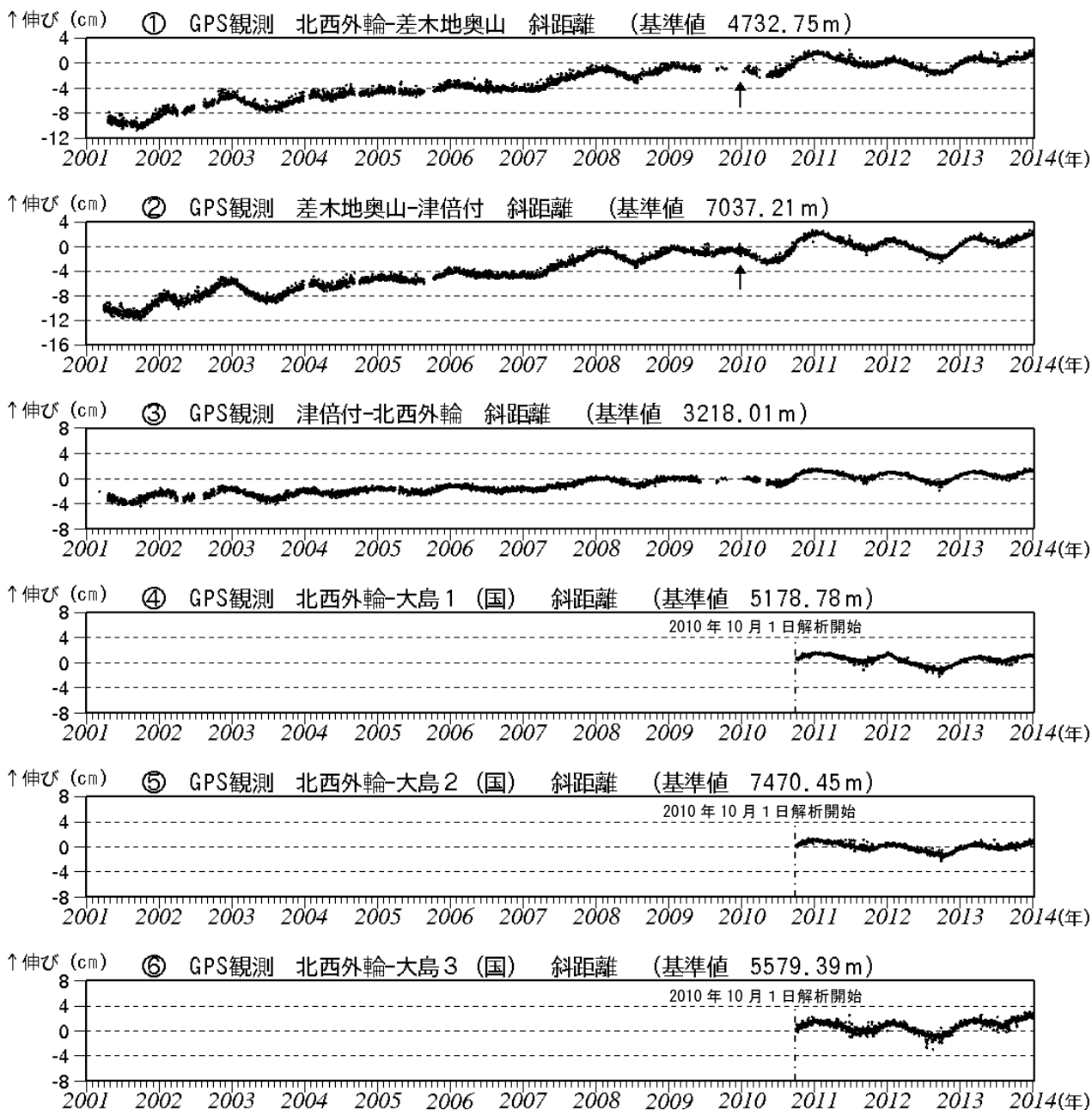
図4 伊豆大島 GPS連続観測による基線長変化(2001年1月～2014年1月6日)(国): 国土地理院 2010年10月以降のデータについては、電離層の影響を補正する等、解析方法を改良しています。 ①～⑥は図1のGPS基線①～⑥に対応しています。 グラフの空白部分は欠測。 ①②の矢印は差木地奥山支柱工事を実施。
