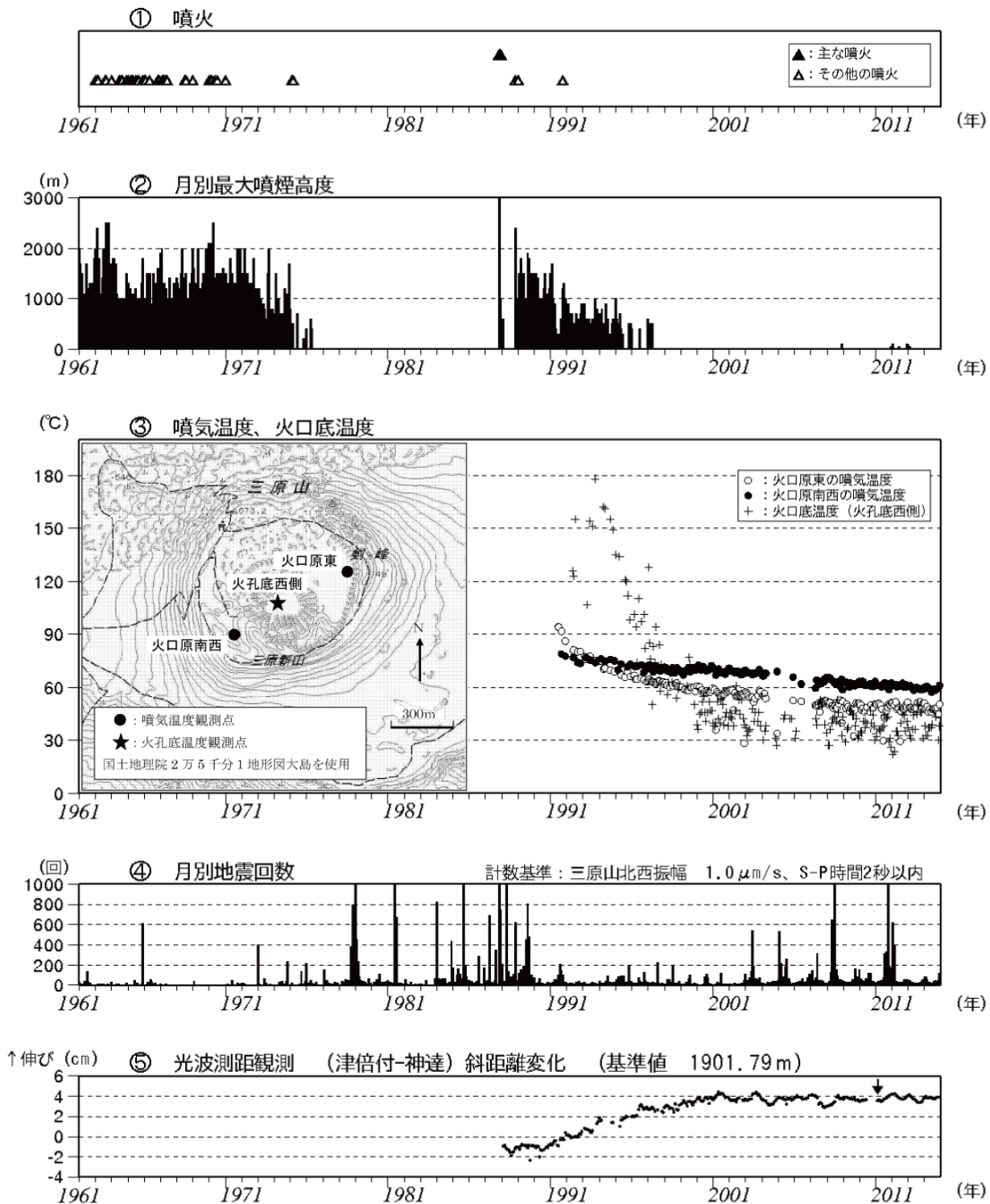
図2 伊豆大島 長期間の火山活動経過図 (1961年1月~2013年12月)
