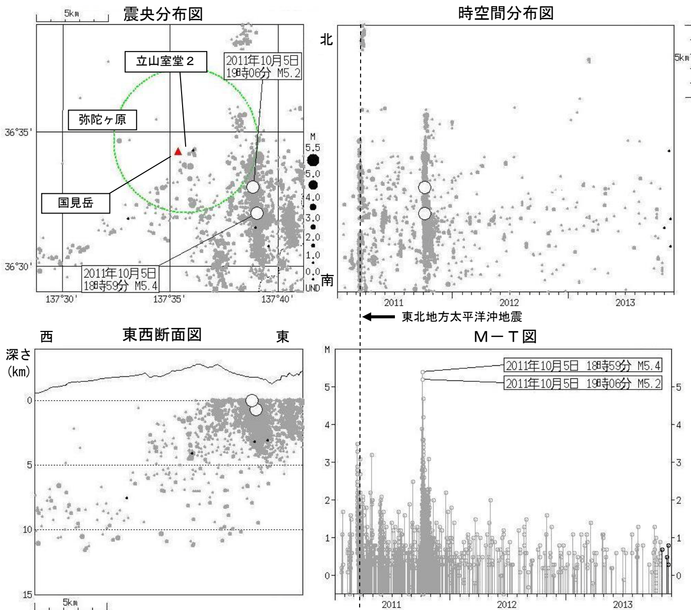
図2 弥陀ヶ原 広域地震観測網による山体・周辺の地震活動 (2011年1月1日~2013年11月30日) ● : 2011年1月1日~2013年10月31日 ● : 2013年11月1日~11月30日 ・ 緑色の点線の円は、立山室堂に設置した地震計(立山室堂2)でS-P時間1秒以内となるおよその範囲を示します。 ・ 今期間、周辺の地震活動は低下しながら継続しています。 ・ 弥陀ヶ原近傍の地震活動は、低調な状況で経過しました。 ・ M (マグニチュード) は地震の規模を表します。 ・ 図中の震源要素は一部暫定値が含まれており、後日変更することがあります。
