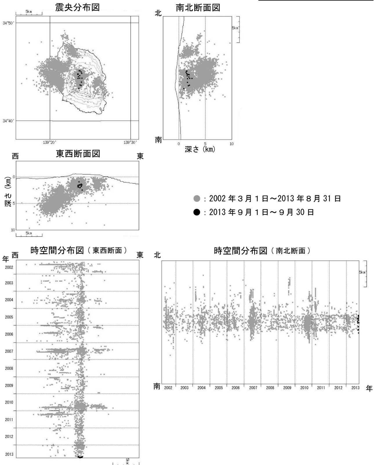
図 7 伊豆大島 震源分布図 (2002 年 3 月 1 日 ~ 2013 年 9 月 30 日)
