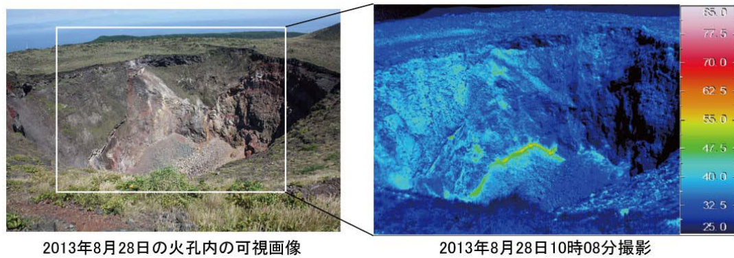
2013年9月19日の火口内の可視画像 2013年9月19日10時14分撮影 2013年8月28日の火口内の可視画像 2013年8月28日10時08分撮影 図5 伊豆大島 中央火口内の状況（左）と地表面温度分布 1) （右）
