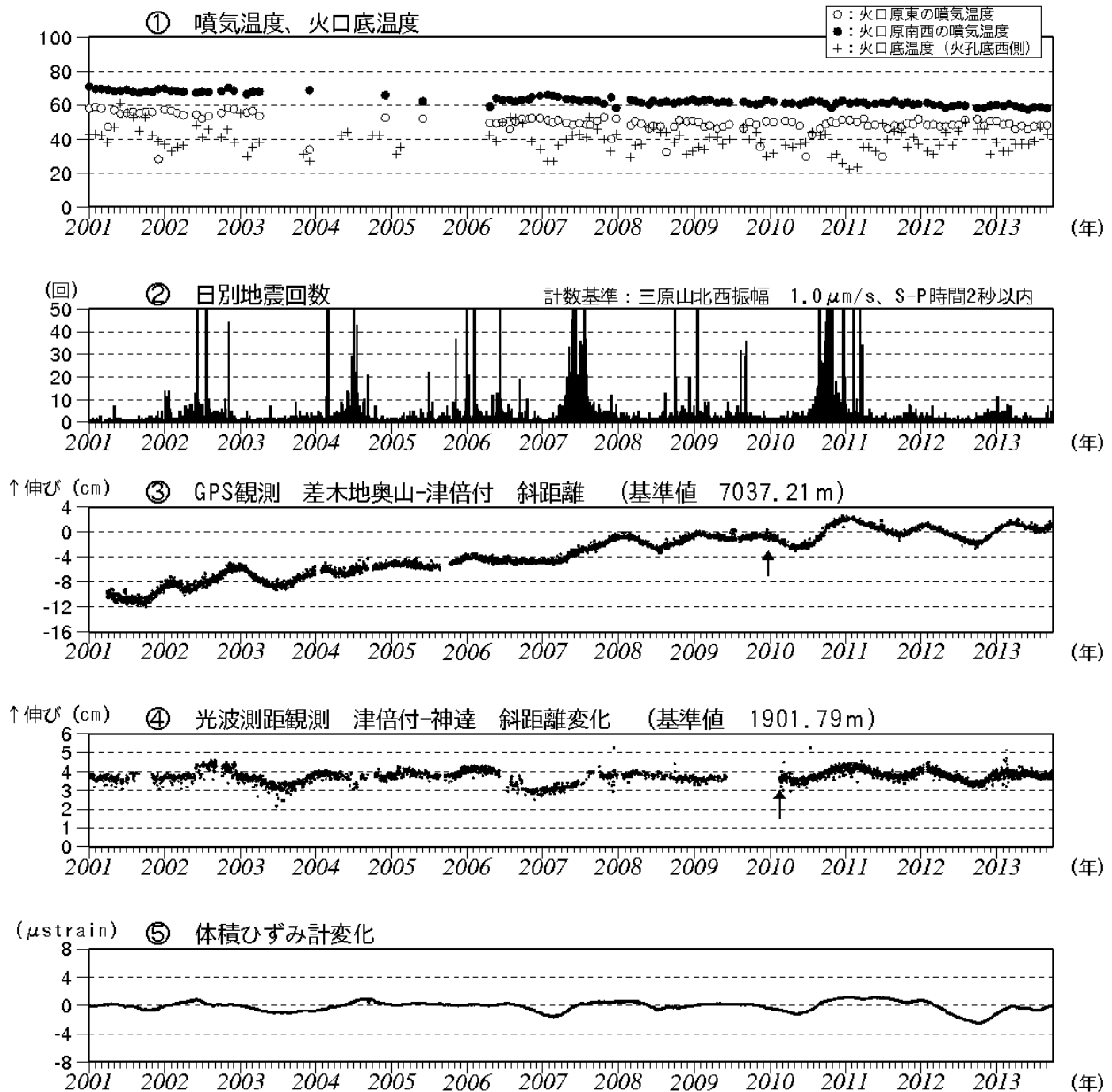
図2 伊豆大島 最近の火山活動経過図 (2001年1月~2013年9月)
