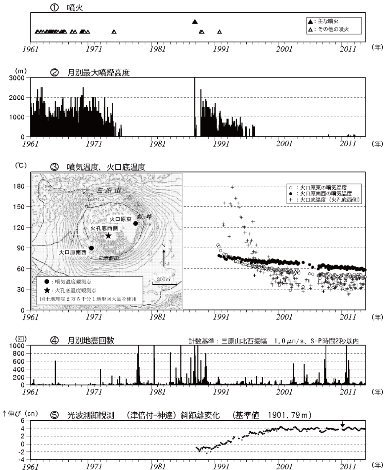
図 1 伊豆大島 長期間の火山活動経過図 (1961 年 1 月～2013 年 9 月)
