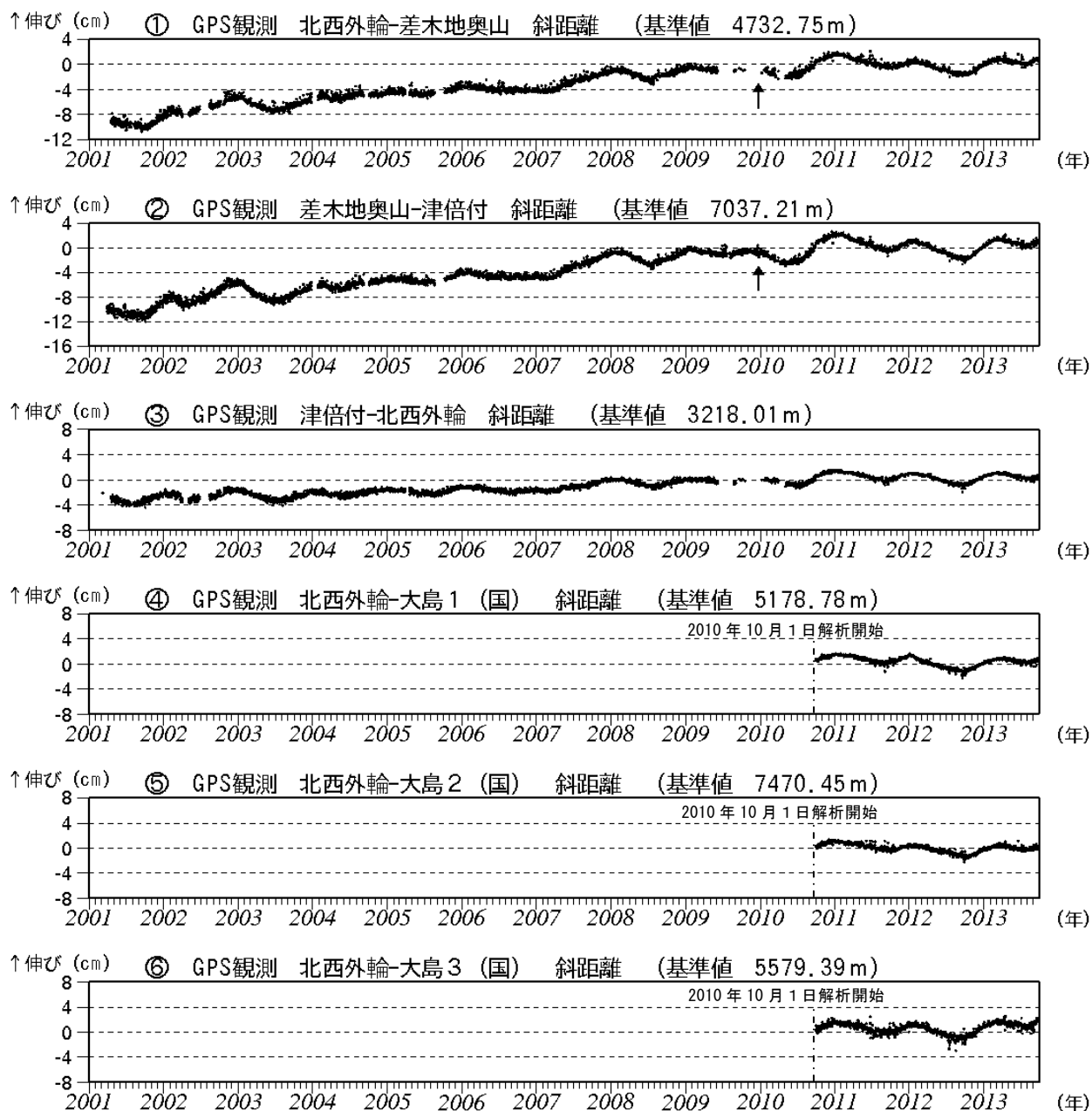
図3 伊豆大島 GPS 連続観測による基線長変化 (2001 年 1 月～2013 年 9 月) (国) : 国土地理院 2010 年 10 月以降のデータについては、電離層の影響を補正する等、解析方法を改良しています。 ①～⑥は図 8 の GPS 基線①～⑥に対応しています。 グラフの空白部分は欠測。 ①②の矢印は差木地奥山支柱工事を実施。
