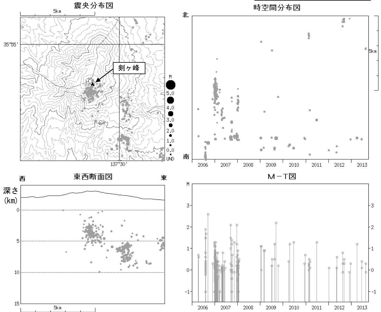
図 4 御嶽山 広域地震観測網による山体・周辺の震源分布図（2006 年 1 月 1 日～2013 年 9 月 30 日）
