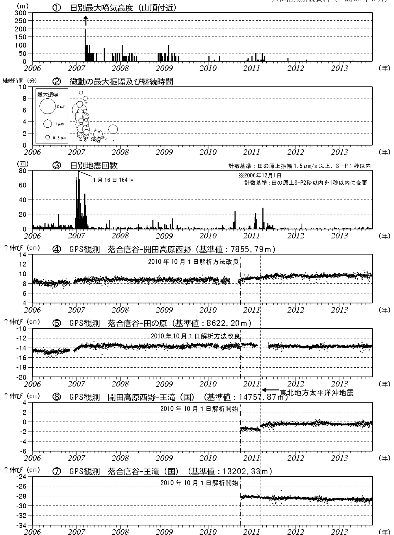
図3 御嶽山 最近の火山活動経過図（2006年1月1日～2013年9月30日）
