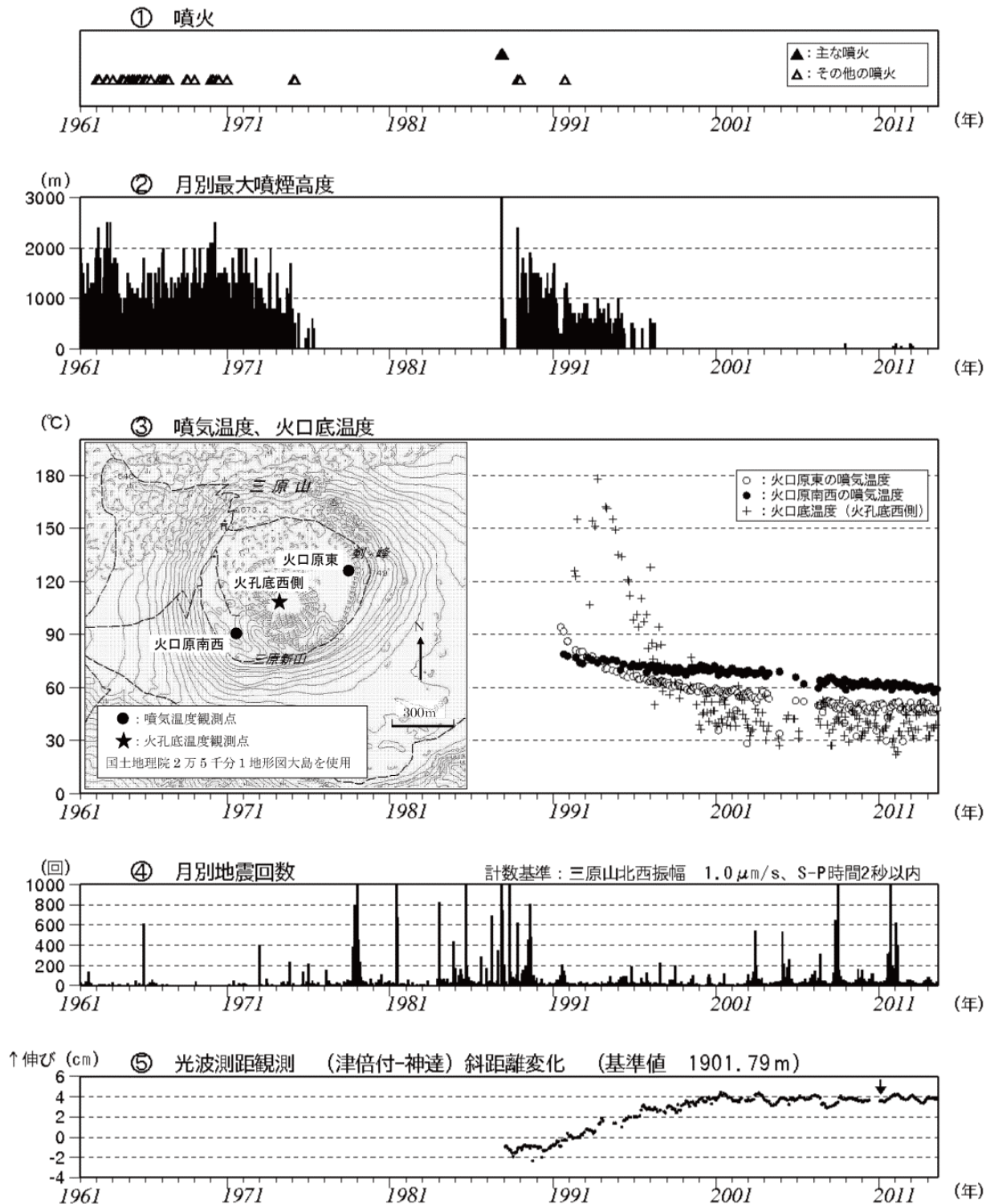
図 1 伊豆大島 長期間の火山活動経過図（1961 年 1 月～2013 年 8 月）
