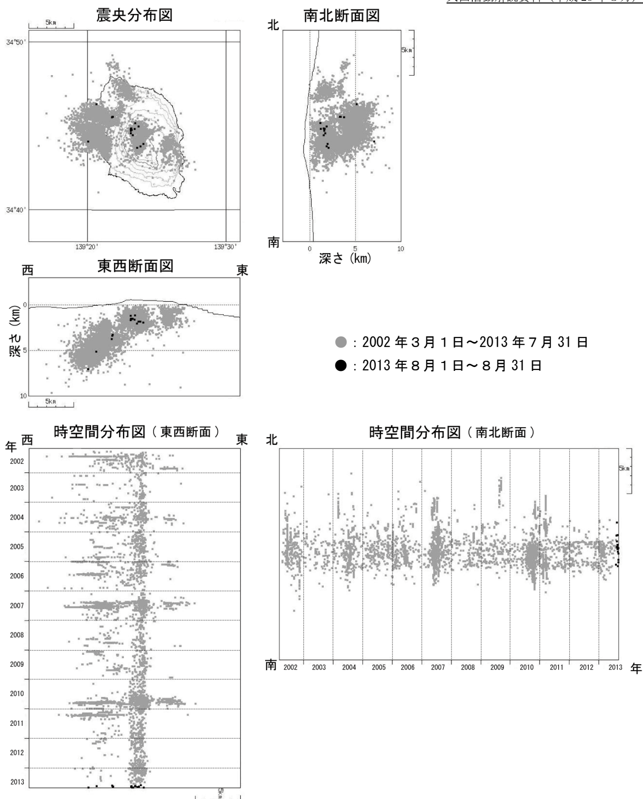
図 7 伊豆大島 震源分布図（2002 年 3 月 1 日～2013 年 8 月 31 日）
