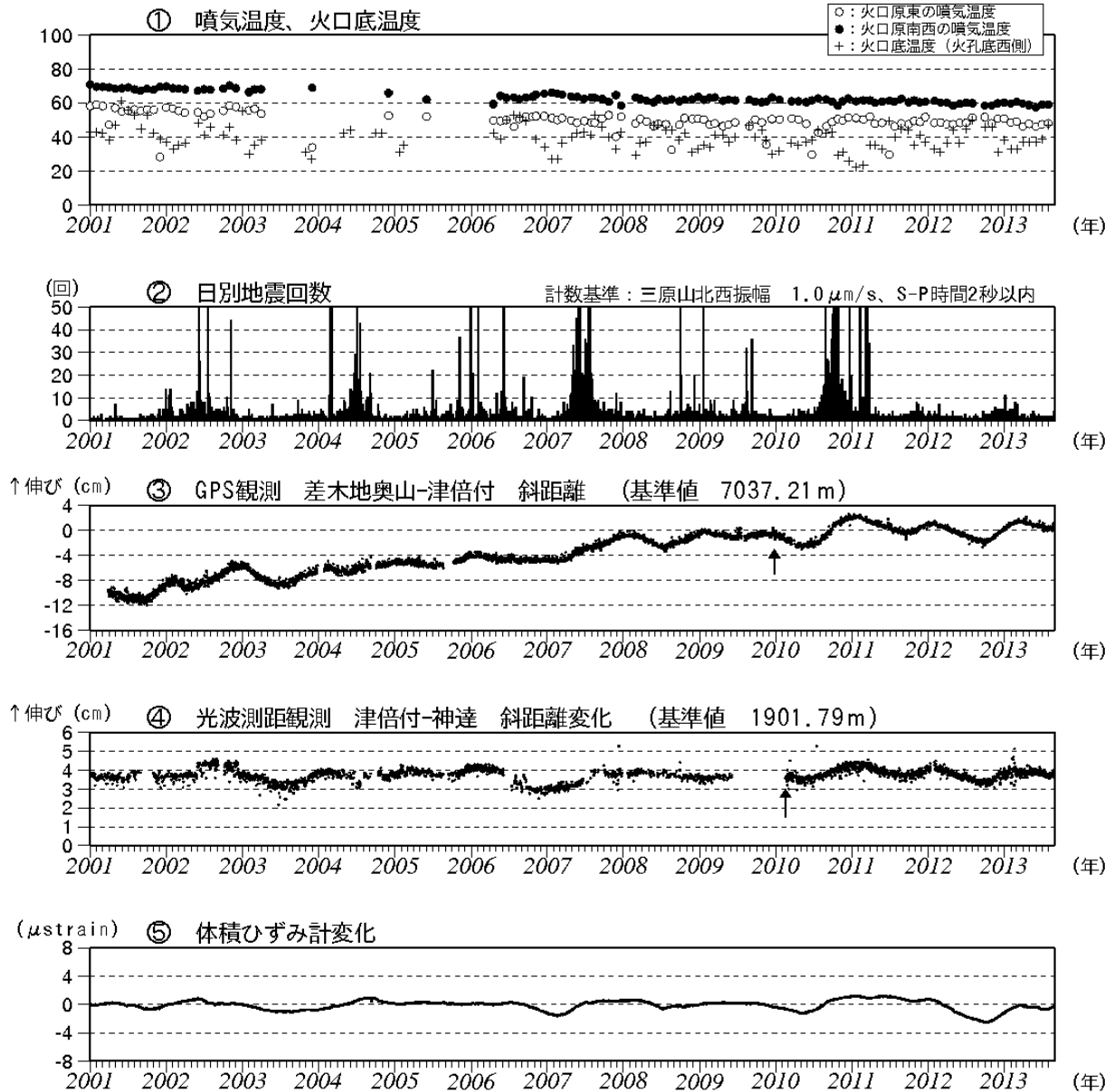
図2 伊豆大島 最近の火山活動経過図（2001年1月～2013年8月）
