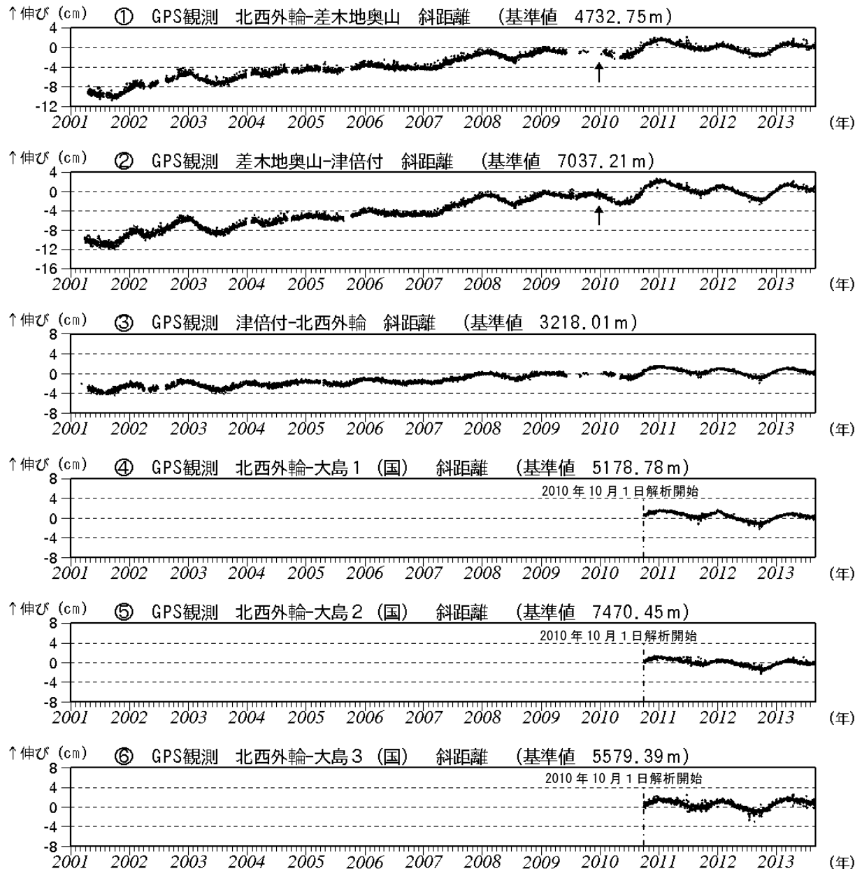
図3 伊豆大島 GPS連続観測による基線長変化(2001年1月～2013年8月) (国): 国土地理院 2010年10月以降のデータについては、電離層の影響を補正する等、解析方法を改良しています。 ①～⑥は図8のGPS基線①～⑥に対応しています。 グラフの空白部分は欠測。 ①②の矢印は差木地奥山支柱工事を実施。
