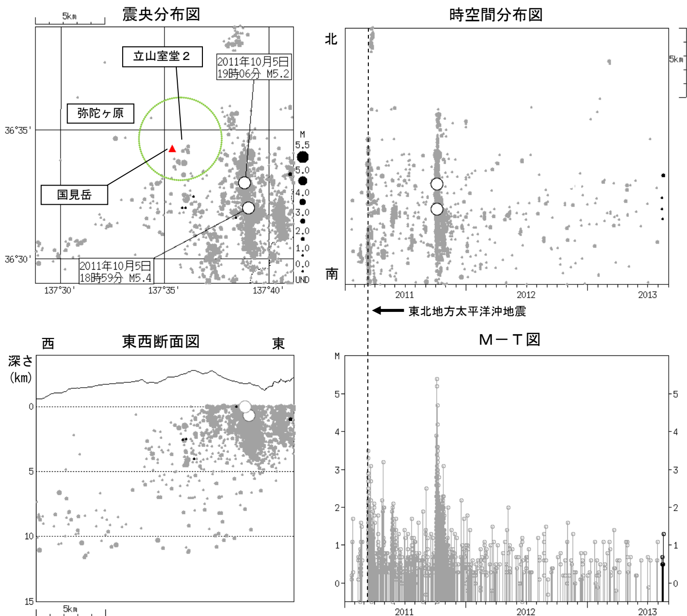
図2 弥陀ヶ原 広域地震観測網による山体・周辺の地震活動（2011年1月1日～2013年8月31日）
