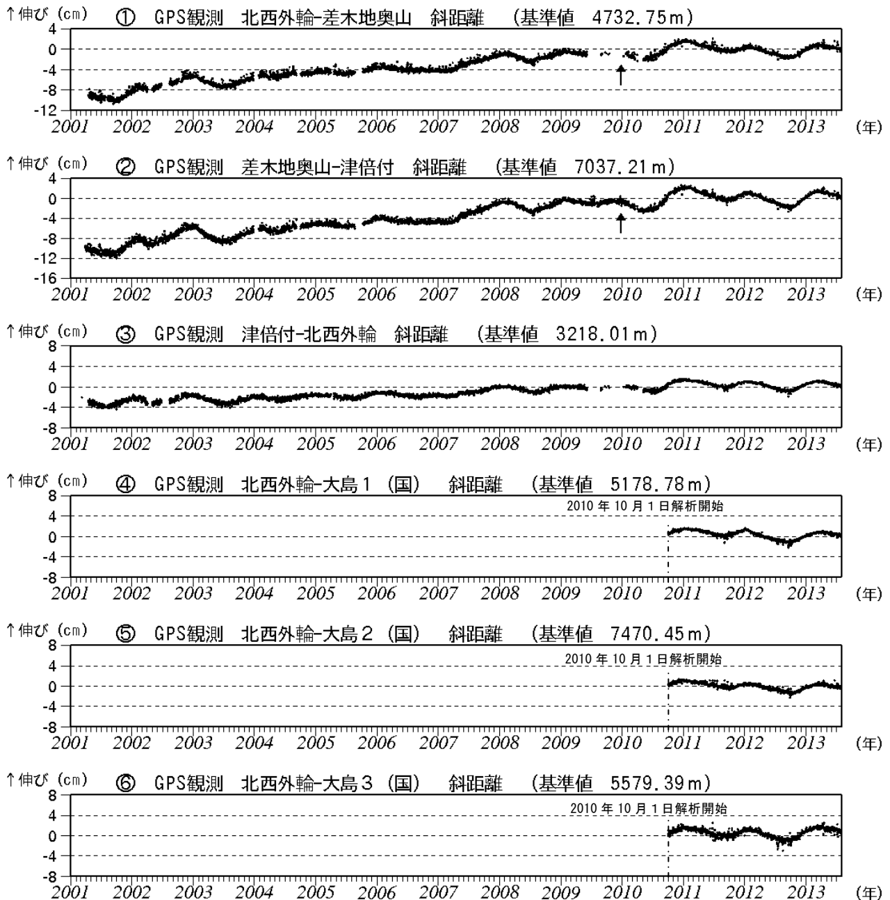
図3 伊豆大島 GPS 連続観測による基線長変化 (2001 年 1 月～2013 年 7 月) (国) : 国土地理院 2010 年 10 月以降のデータについては、電離層の影響を補正する等、解析方法を改良しています。 ①～⑥は図8の GPS 基線①～⑥に対応しています。 グラフの空白部分は欠測。 ①②の矢印は差木地奥山支柱工事を実施。
