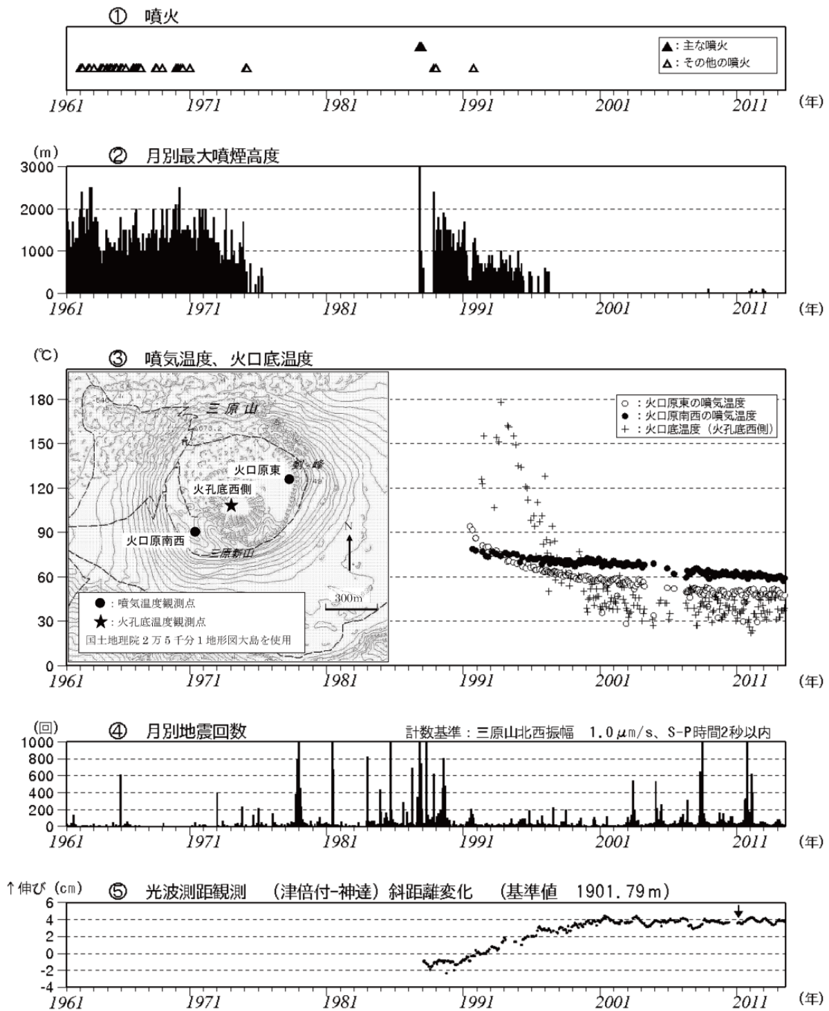
図 1 伊豆大島 長期間の火山活動経過図（1961 年 1 月～2013 年 7 月）
