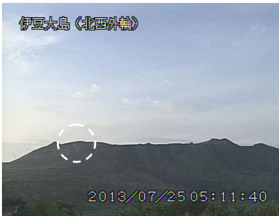
山頂部 (7月25日、北西外輪遠望カメラによる) 三原新山北側 (7月31日、撮影方向は図6参照) 図4 伊豆大島 三原山山頂部及び山頂火口の状況 破線円内: ごく弱い噴気
