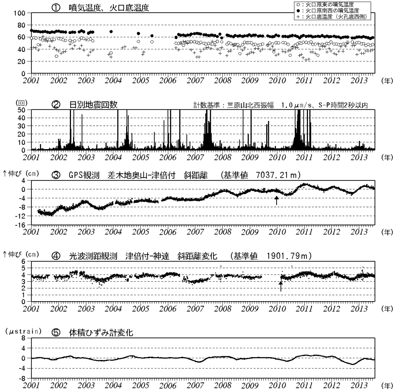
図2 伊豆大島 最近の火山活動経過図（2001年1月～2013年7月）
