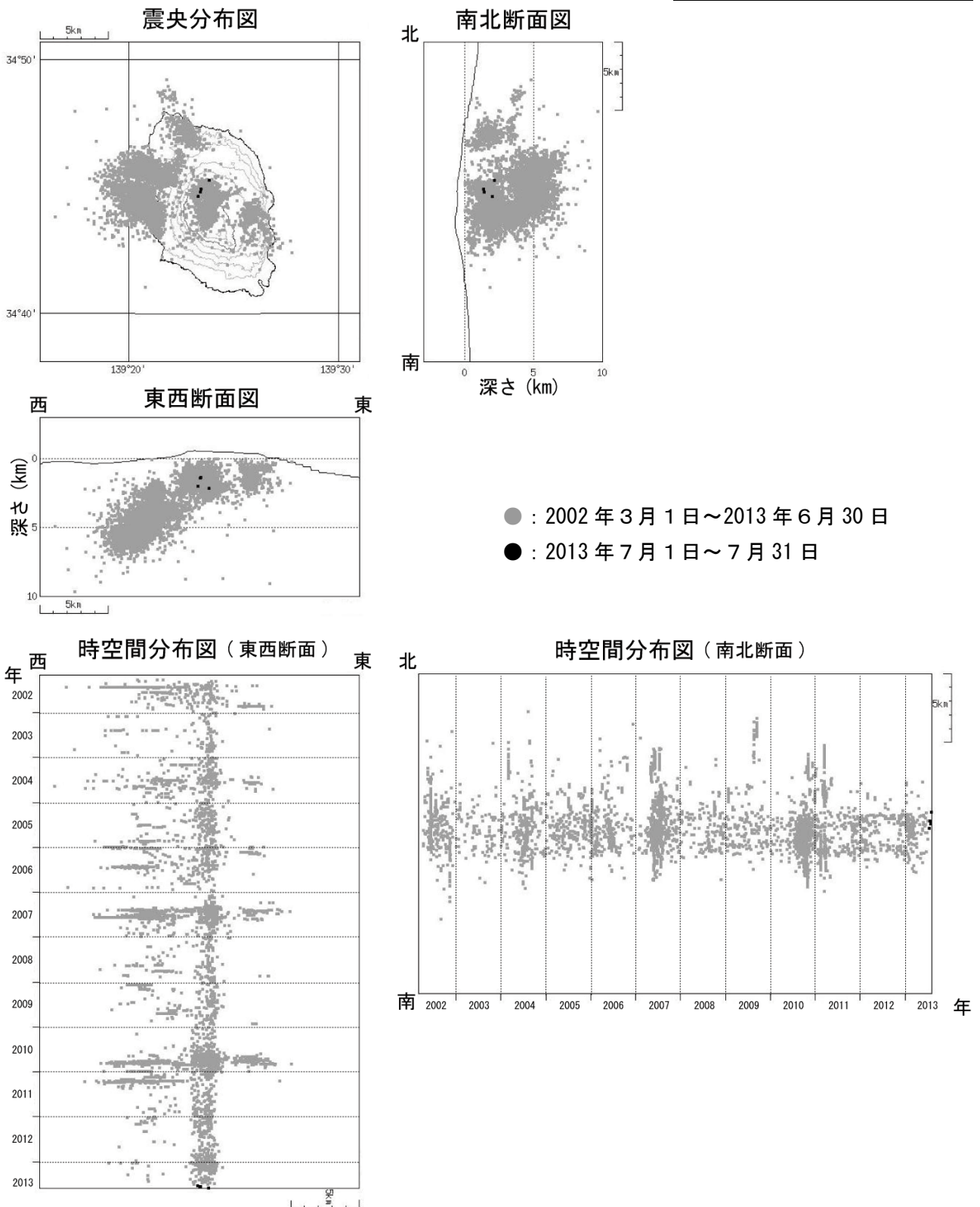
図 7 伊豆大島 震源分布図 (2002 年 3 月 1 日 ~ 2013 年 7 月 31 日)
