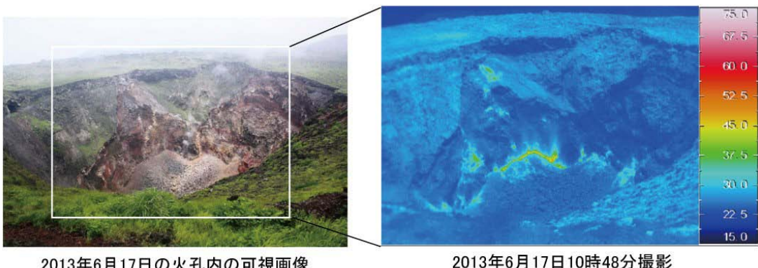
図5 伊豆大島 中央火口内の状況 (左) と地表面温度分布 1) (右)
