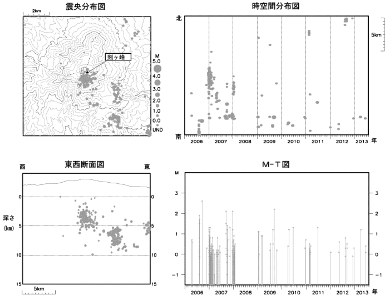
図 4 御嶽山 広域地震観測網による山体・周辺の震源分布図（2006 年 1 月 1 日～2013 年 7 月 31 日） ●：2006 年 1 月 1 日～2013 年 6 月 30 日 ●：2013 年 7 月 1 日～7 月 31 日 M（マグニチュード）は地震の規模を表します。 今期間、震源が決定された地震はありません。 図中の震源要素は一部暫定値が含まれており、後日変更することがあります。
