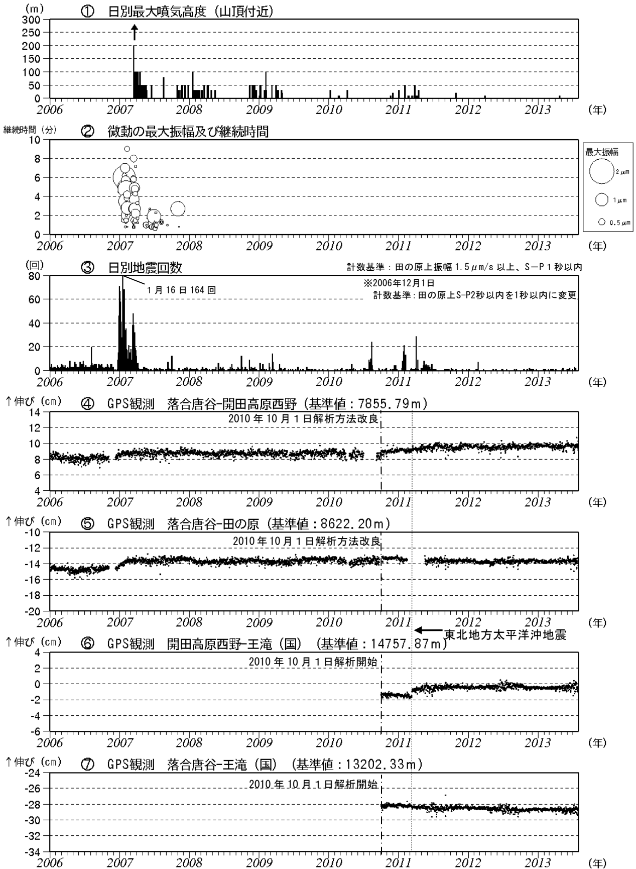
図3 御嶽山 最近の火山活動経過図 (2006年1月1日~2013年7月31日)
