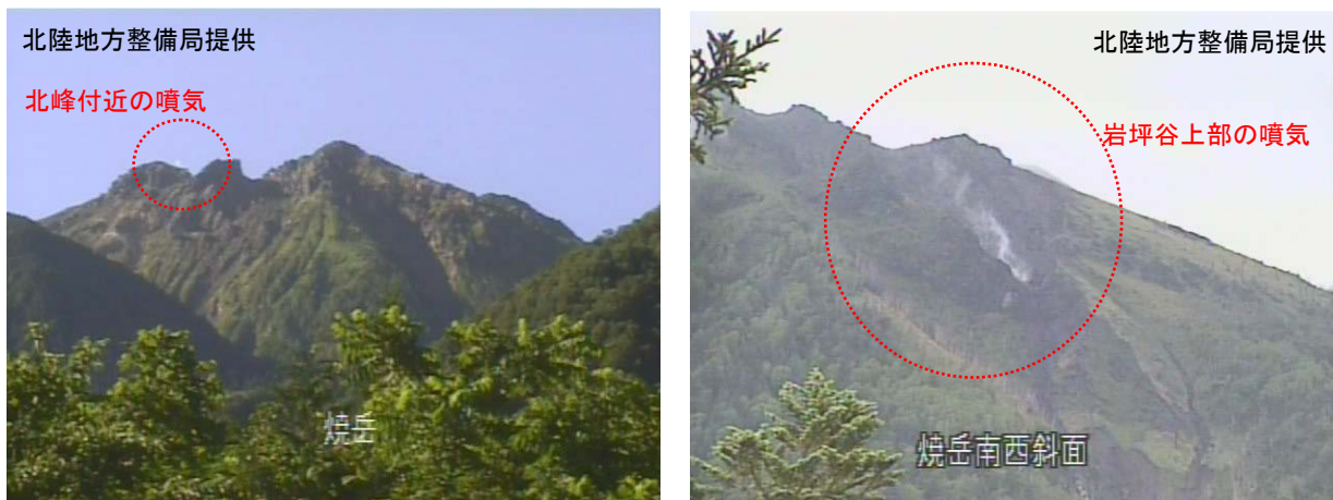
図 2 焼岳 山頂部及び南西斜面の状況 (左図：7月20日 焼岳北カメラ、右図：7月6日 焼岳南西斜面カメラ)
