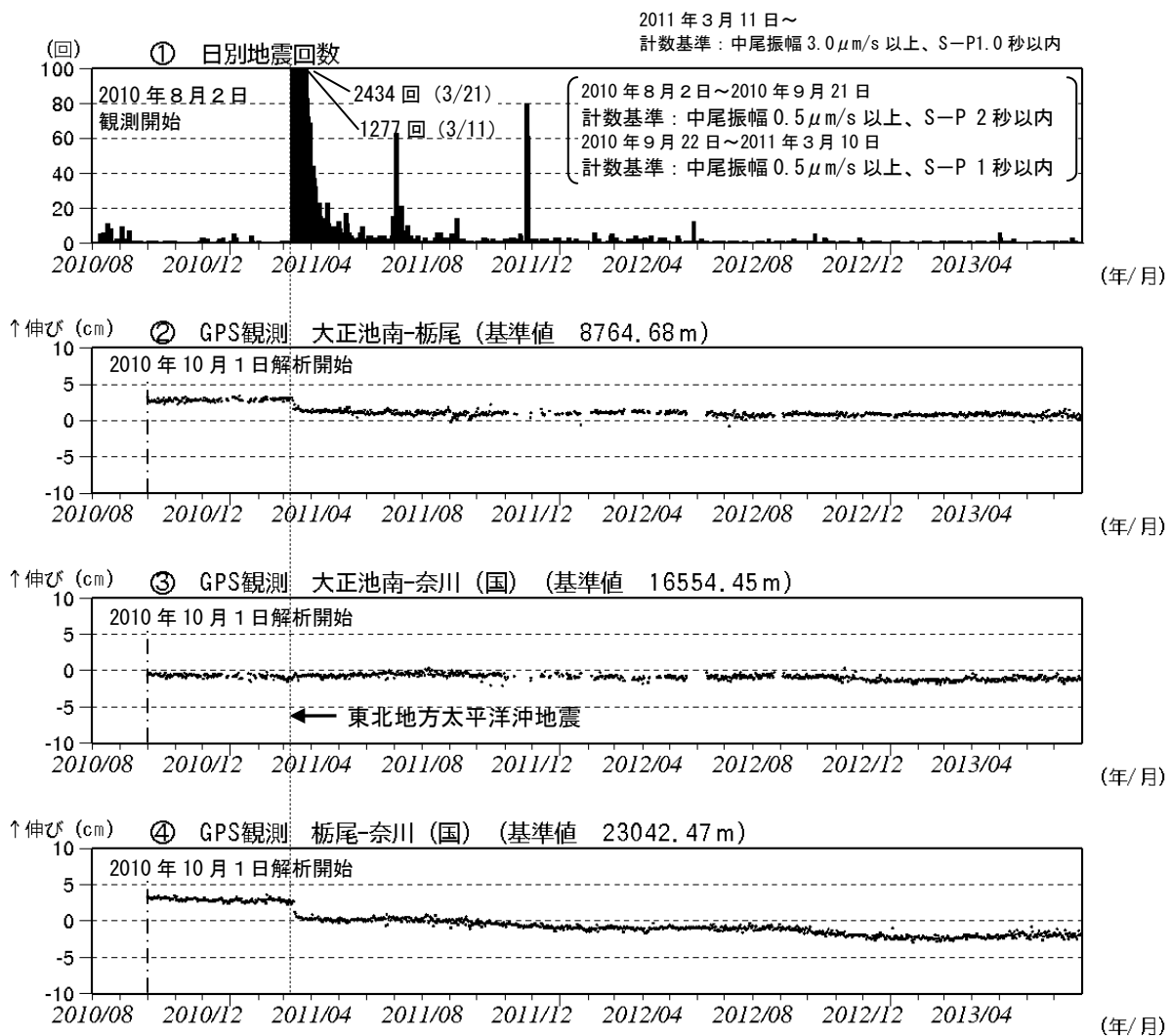
図 3 焼岳 火山活動経過図 (2010年8月2日～2013年7月31日)
