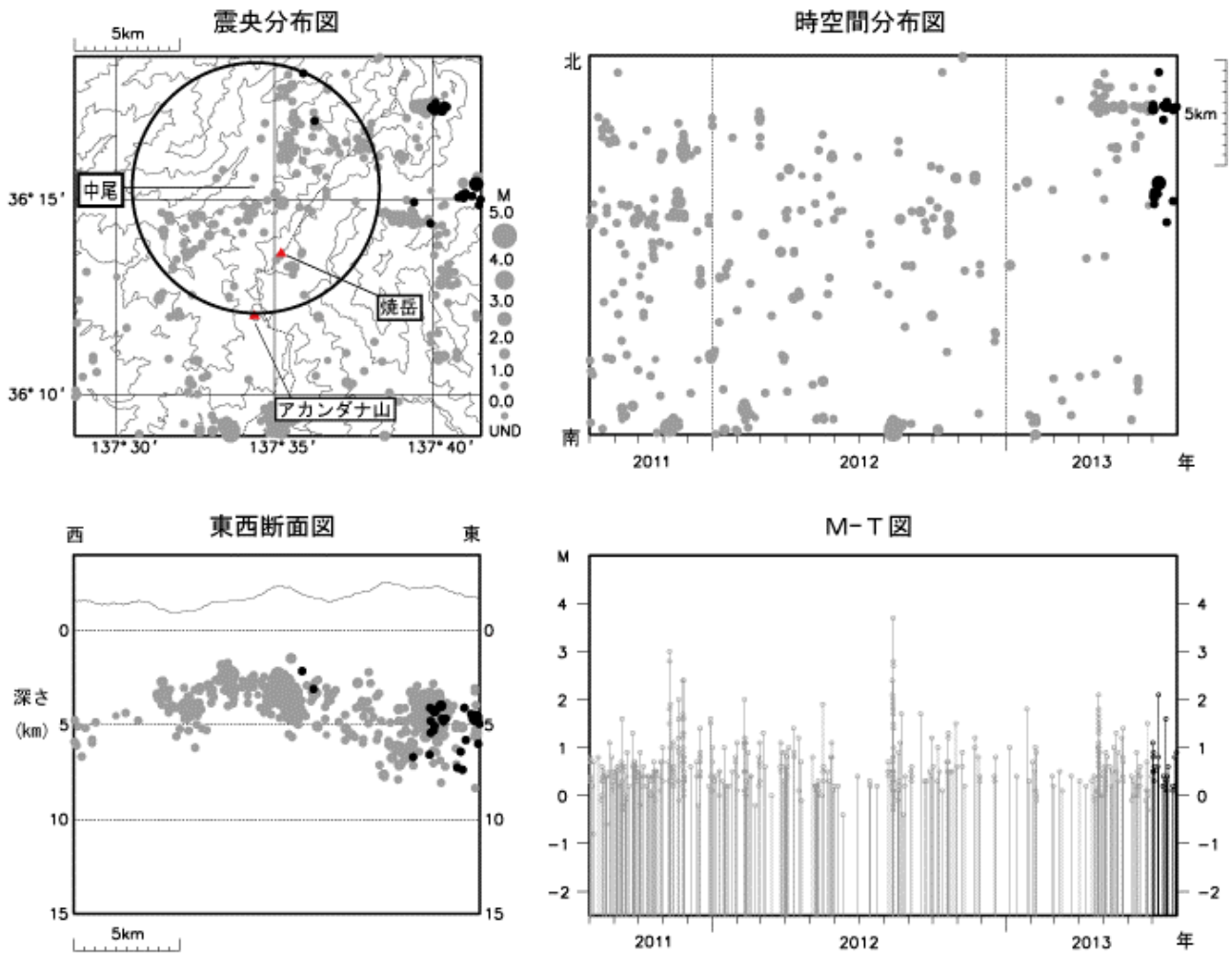
図4 焼岳 広域地震観測網による山体・周辺の地震活動(2011年8月1日～2013年7月31日)
