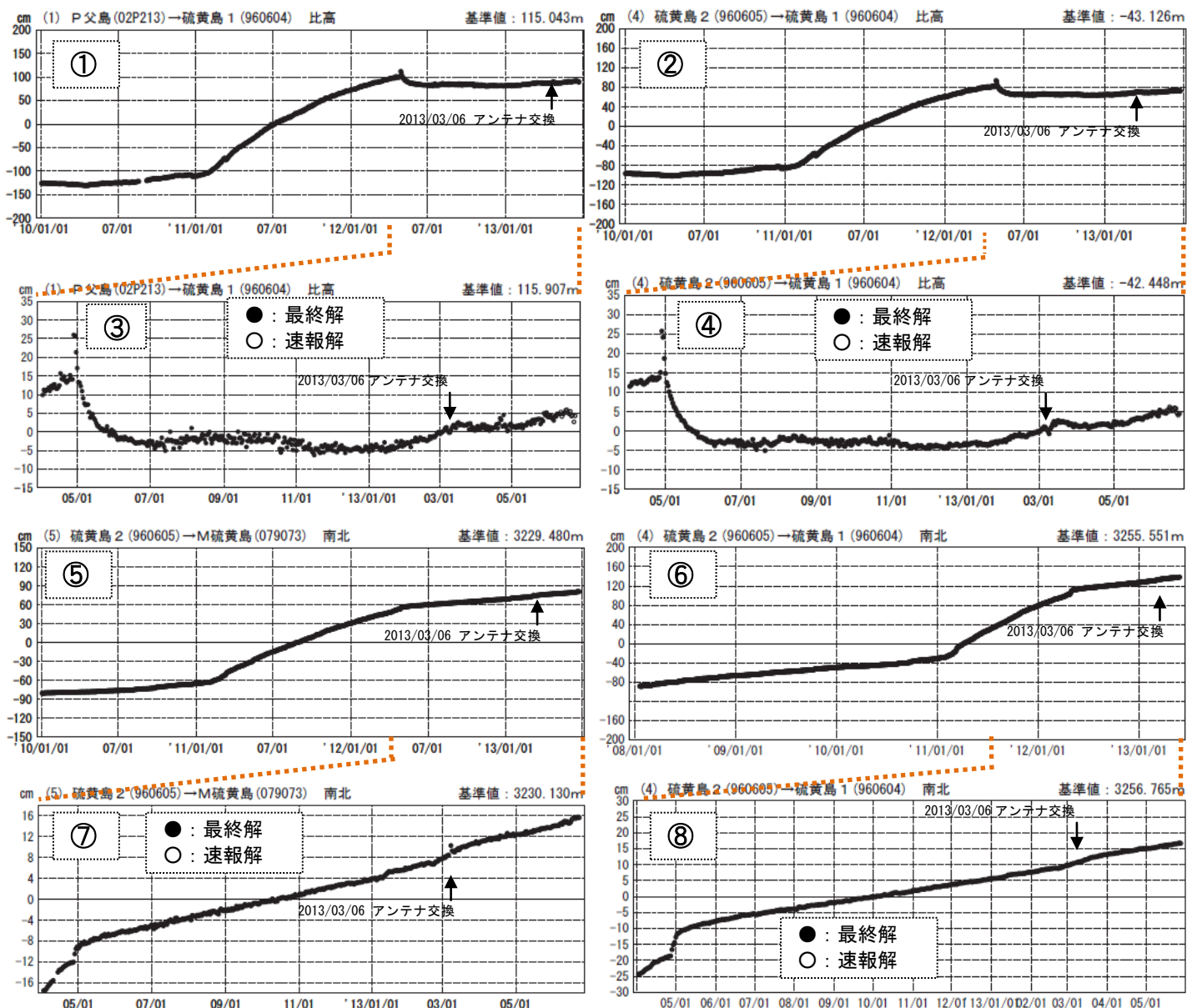
図 6 硫黄島 国土地理院による地殻変動観測結果 1) (2010 年 1 月 1 日～2013 年 6 月 22 日)
