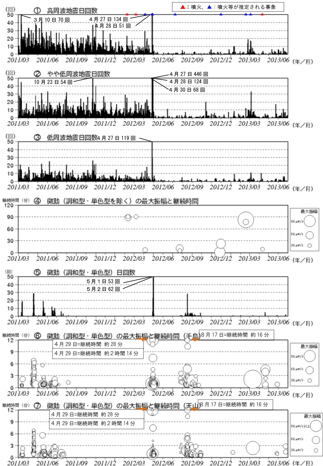
図5 硫黄島 火山活動経過図（2011年3月8日～2013年6月30日）
