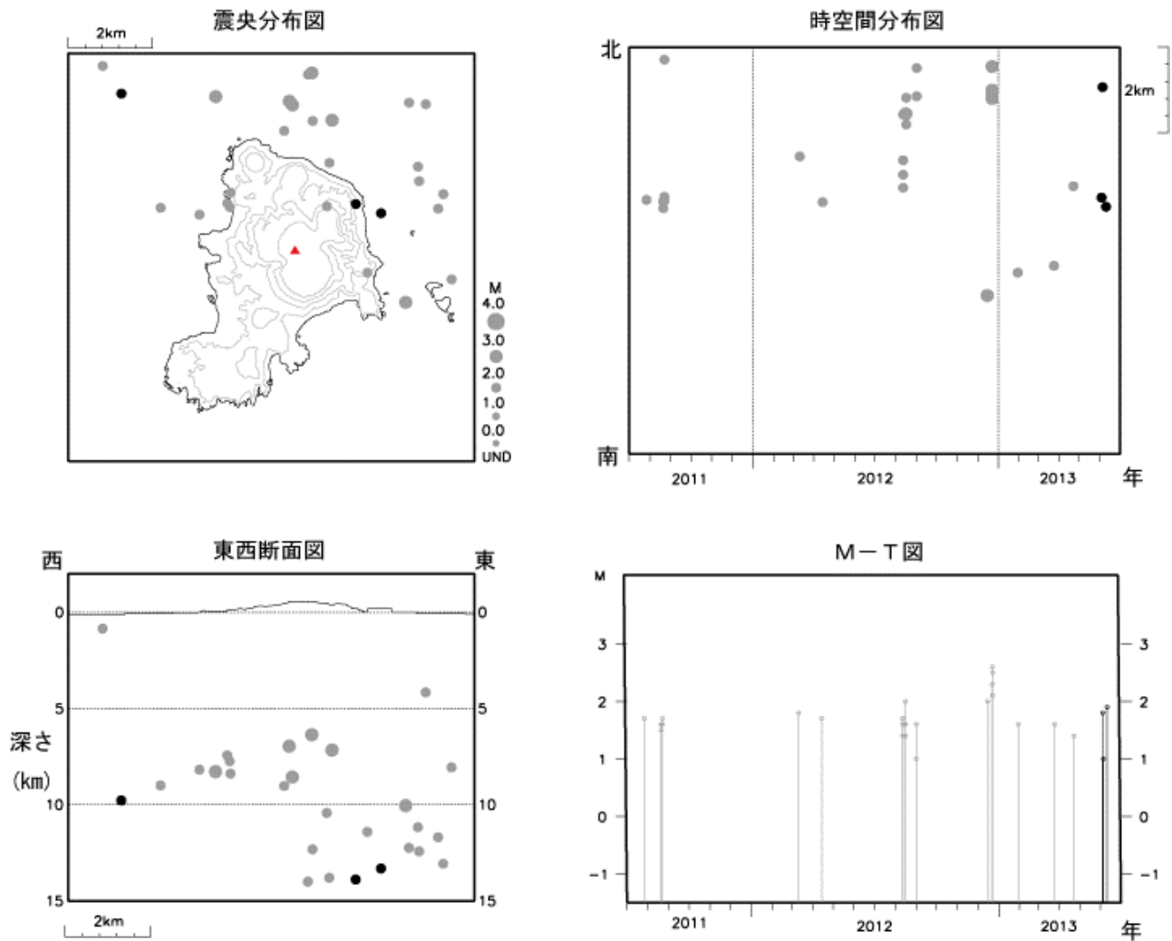
図 4 神津島 広域地震観測網による山体・周辺の地震活動（2011 年 7 月 1 日～2013 年 6 月 30 日）
