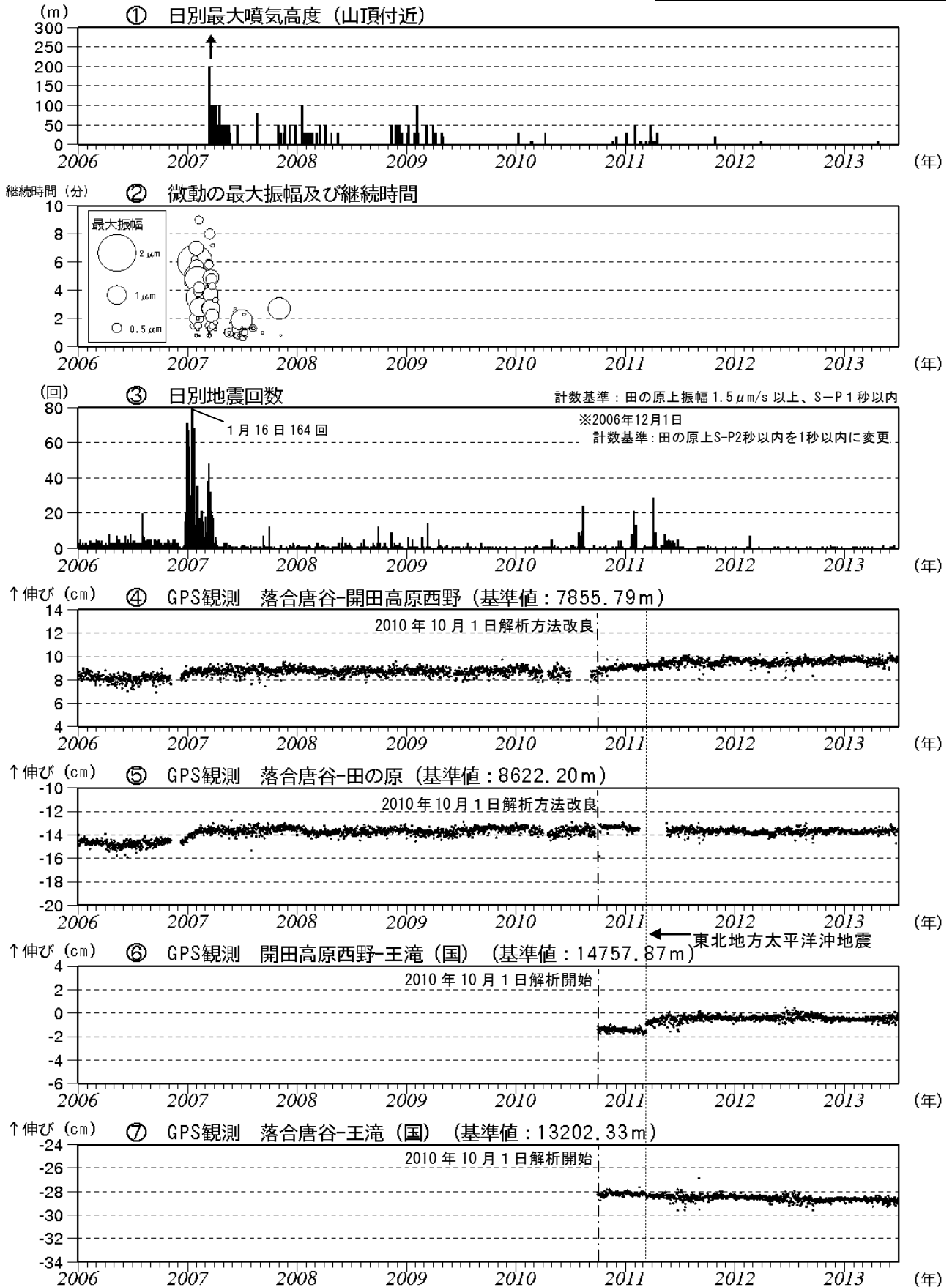
図3 御嶽山 最近の火山活動経過図 (2006年1月1日~2013年6月30日)
