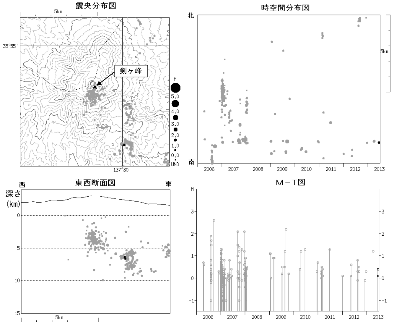
図 4 御嶽山 広域地震観測網による山体・周辺の震源分布図 (2006 年 1 月 1 日~2013 年 6 月 30 日) ● : 2006 年 1 月 1 日~2013 年 5 月 31 日 ● : 2013 年 6 月 1 日~6 月 30 日 M (マグニチュード) は地震の規模を表します。 図中の震源要素は一部暫定値が含まれており、後日変更することがあります。
