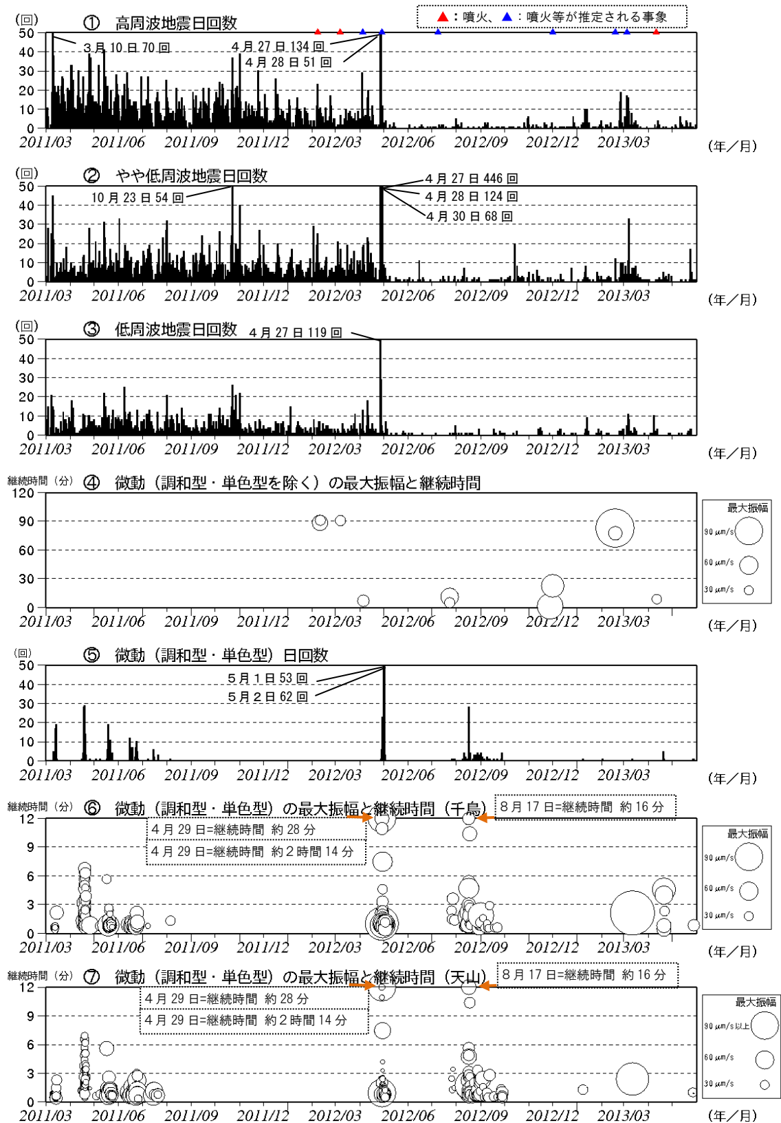
図5 硫黄島 火山活動経過図（2011年3月8日～2013年5月31日）
