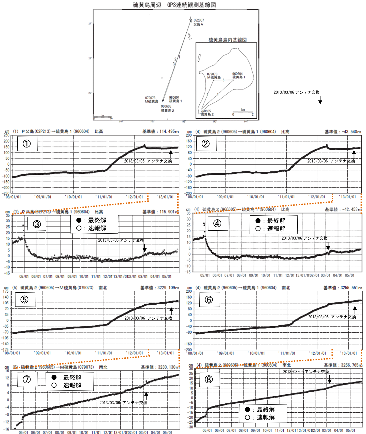
図6 硫黄島 国土地理院による地殻変動観測結果 1) (2008年1月1日～2013年5月27日)
