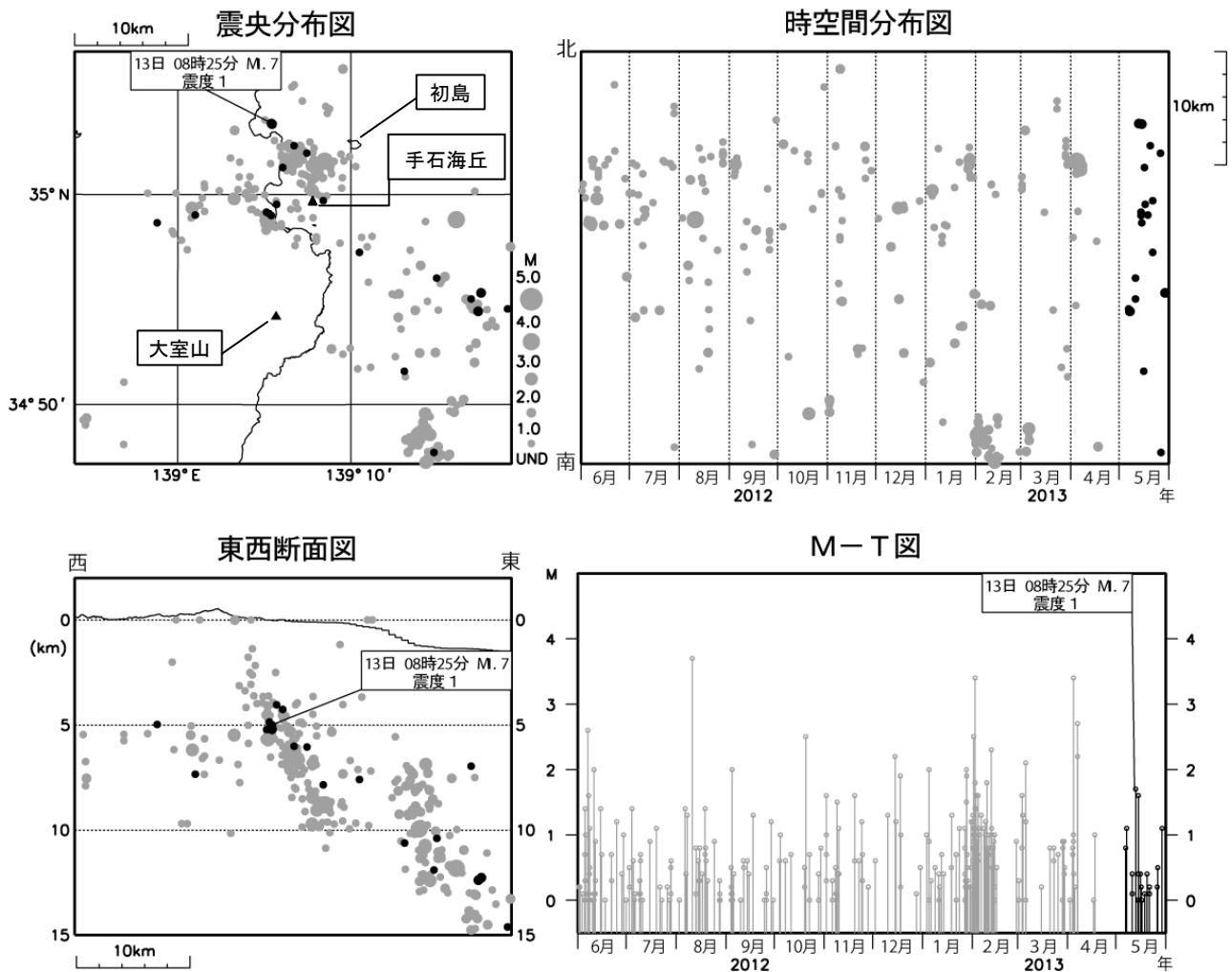
●：2012年6月1日～2013年4月30日 ●：2013年5月1日～5月31日 図 2 伊豆東部火山群 広域地震観測網による震源分布図（2012年6月1日～2013年5月31日） M（マグニチュード）は地震の規模を表します。 図中の震源要素は一部暫定値が含まれており、後日変更することがあります。
