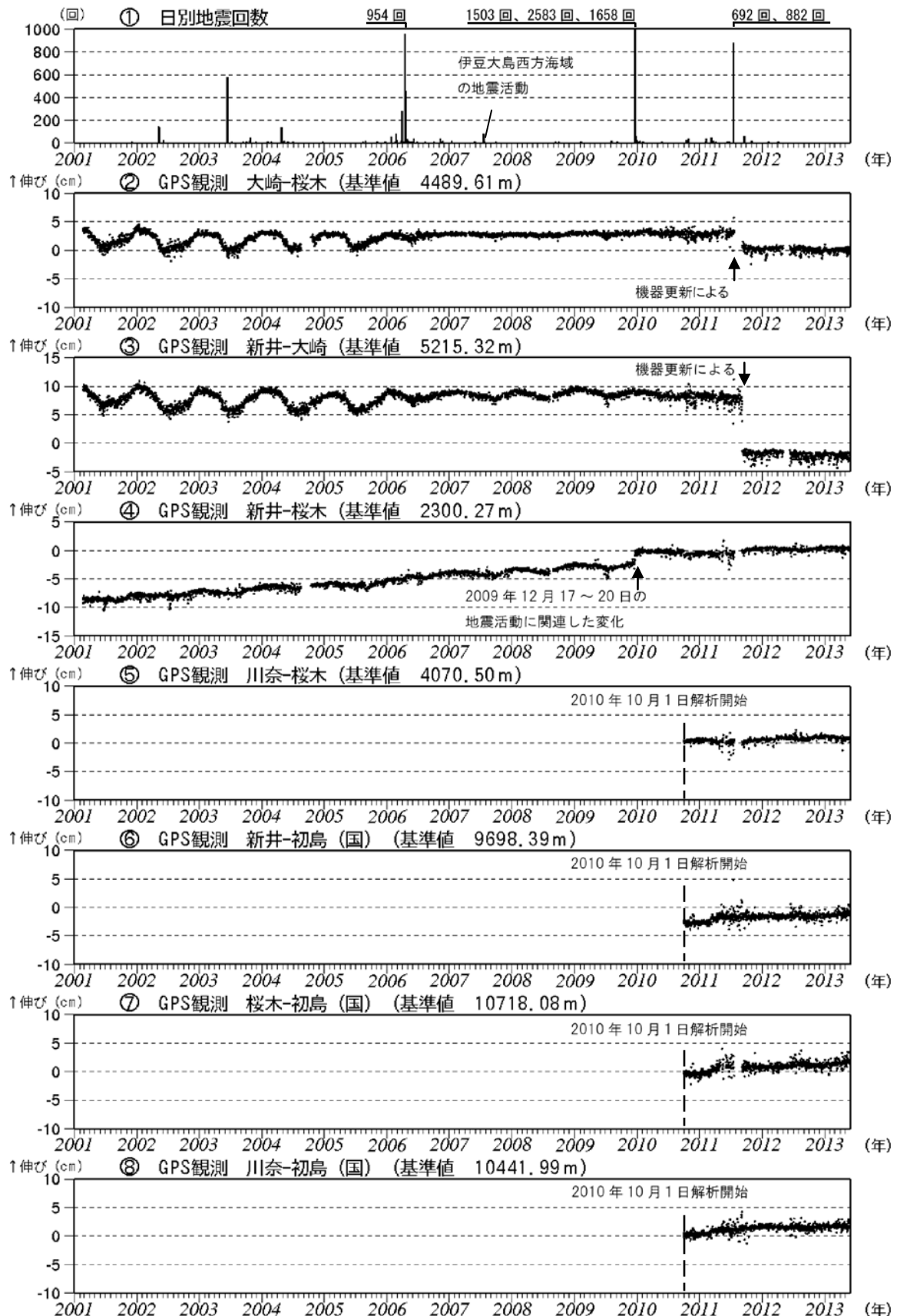
図3 伊豆東部火山群 最近の火山活動経過図（2001年1月～2013年5月）
