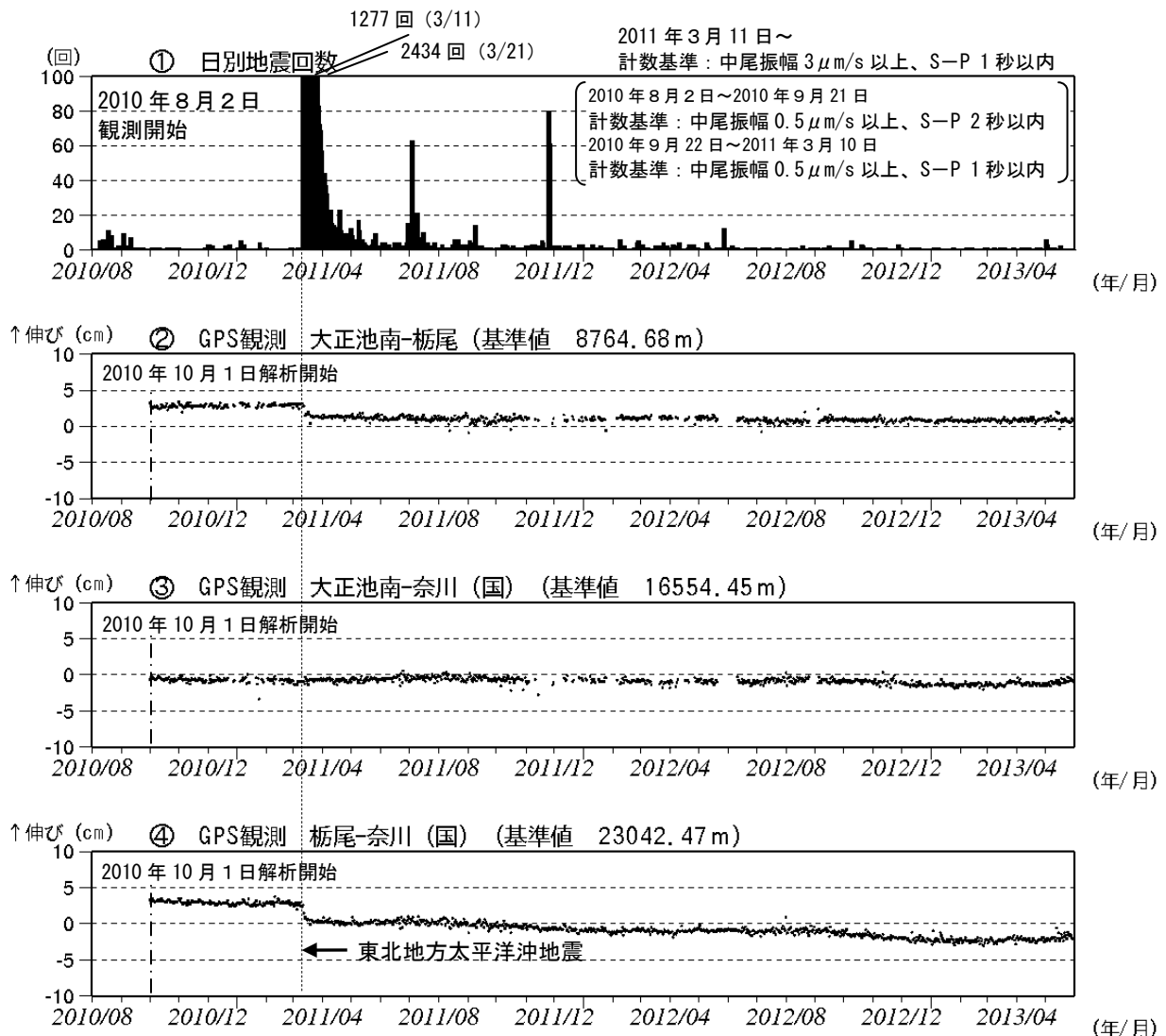
図3 焼岳 火山活動経過図 (2010年8月2日～2013年5月31日)
