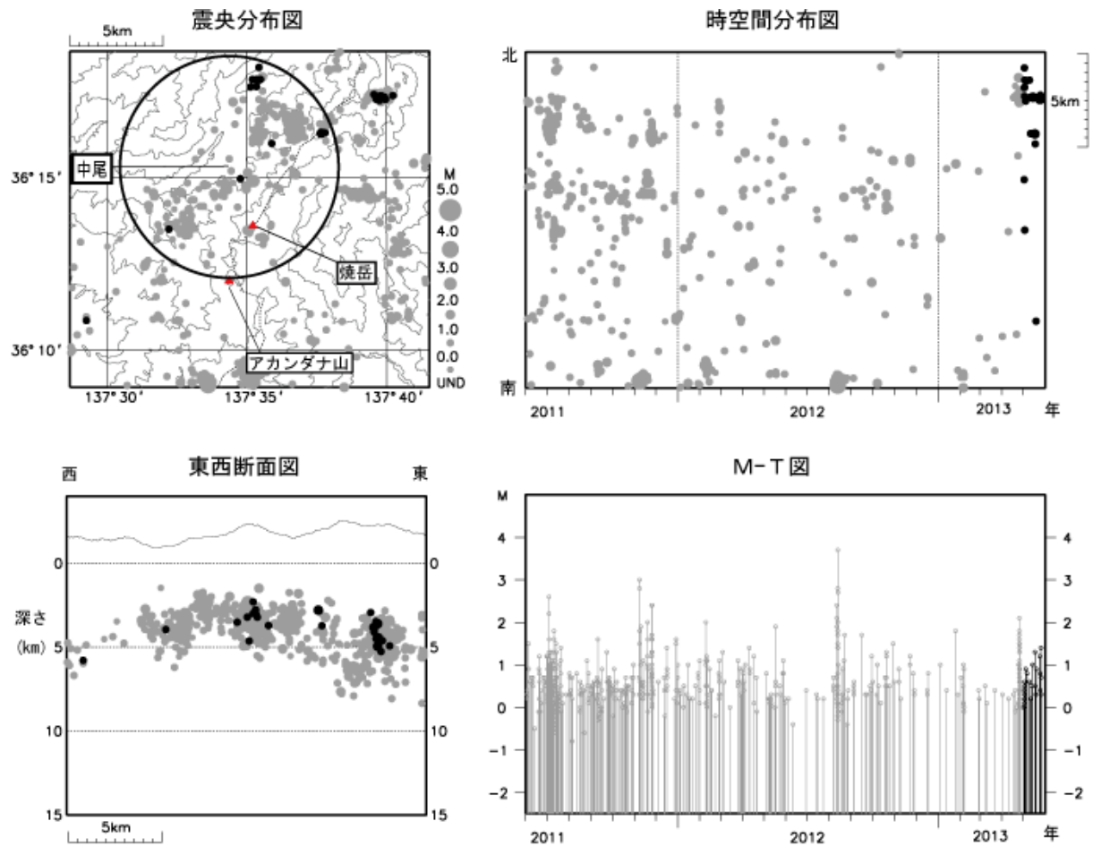
図4 焼岳 広域地震観測網による山体・周辺の地震活動(2011年6月1日～2013年5月31日)
