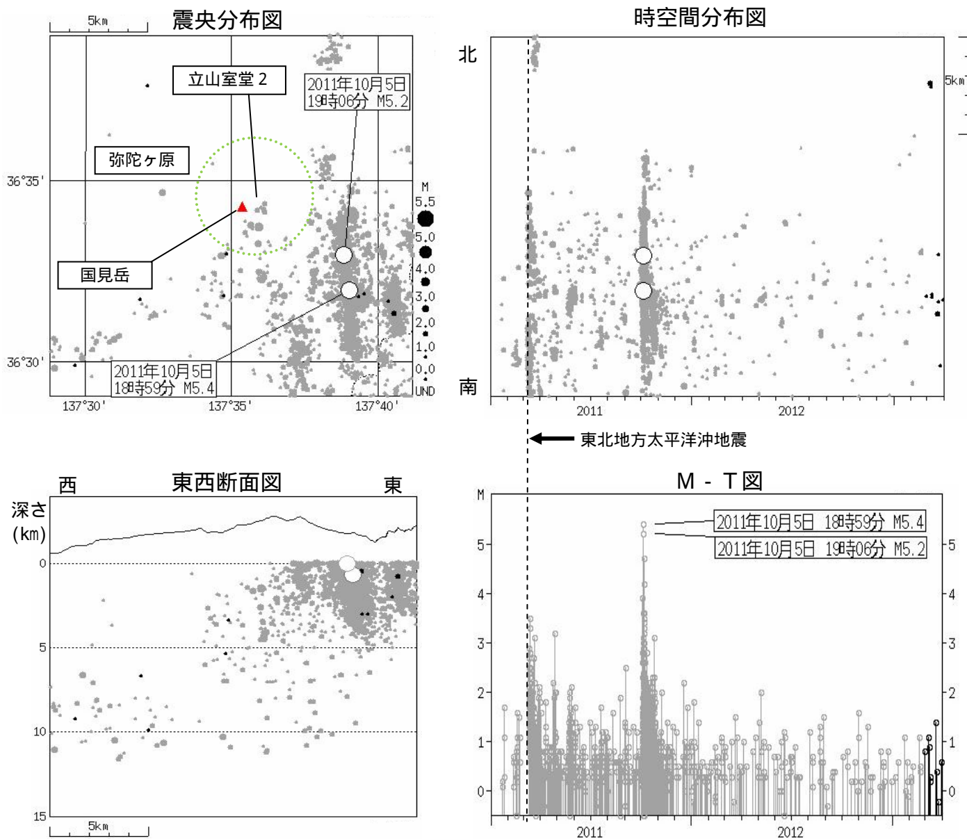
図2 弥陀ヶ原 広域地震観測網による山体・周辺の地震活動(2011年1月1日~2013年3月31日) : 2011年1月1日~2013年2月28日 : 2013年3月1日~3月31日 ・ 緑色の点線の円は、立山室堂に設置した地震計(立山室堂2)でS-P時間1秒以内となるおよその範囲を示します。 ・ 今期間、周辺の地震活動は低下しながら継続しています。 ・ 弥陀ヶ原近傍の地震活動は、低調な状況で経過しました。 ・ M(マグニチュード)は地震の規模を表します。 ・ 図中の震源要素は一部暫定値が含まれており、後日変更することがあります。
